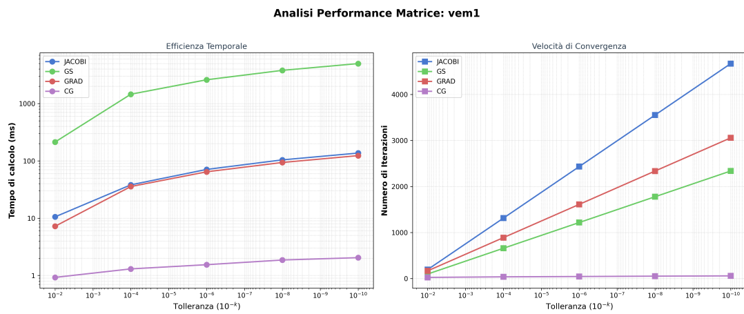
Figura 3: Matrice VEM1: tempo di calcolo e numero di iterazioni al variare della tolleranza.
