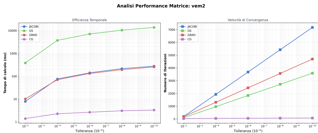
Figura 4: Matrice VEM2: tempo di calcolo e numero di iterazioni al variare della tolleranza.
