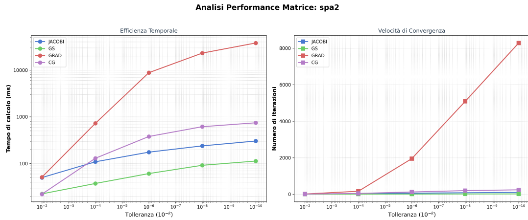
Figura 2: Matrice SPA2: tempo di calcolo e numero di iterazioni al variare della tolleranza.
