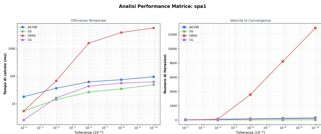
Figura 1: Matrice SPA1: tempo di calcolo e numero di iterazioni al variare della tolleranza.
