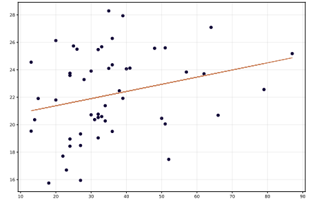
(d) Repulsing triangles corr = 0.26, p = 0.05
