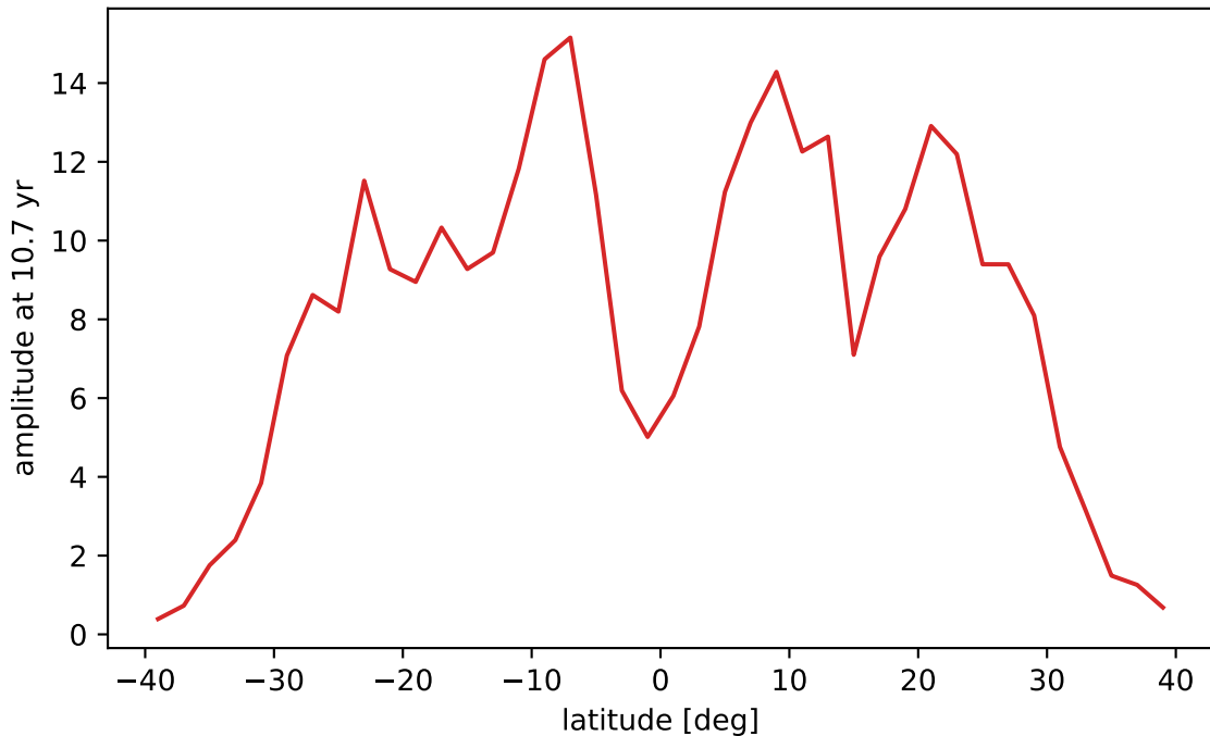
Cycle-amplitude vs. latitude
