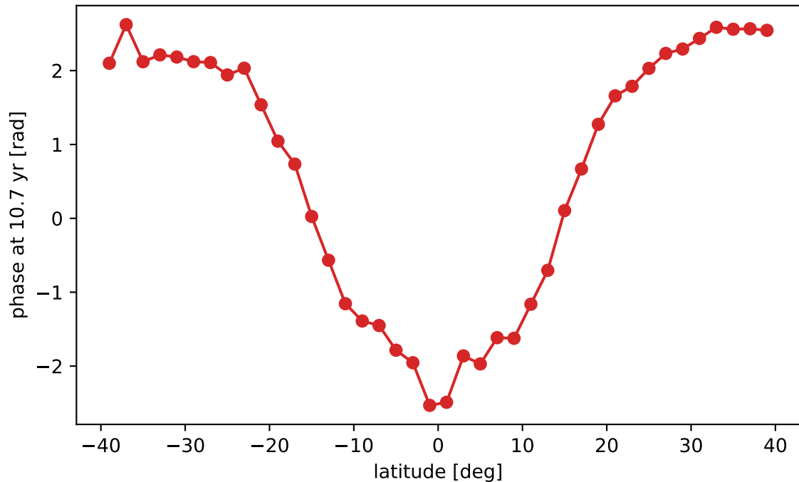
Cycle-phase vs. latitude (unwrapped)
