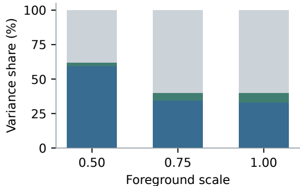
AdamCodd
