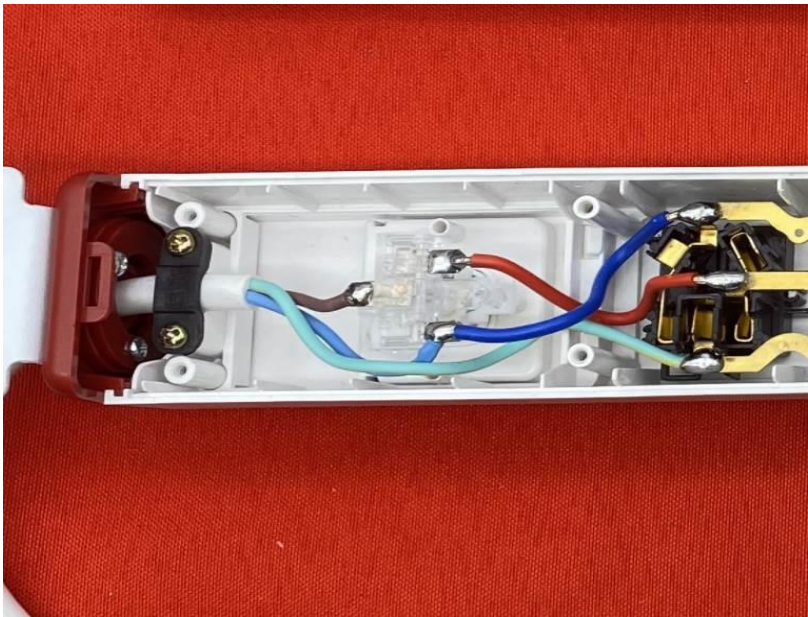
内部结构
