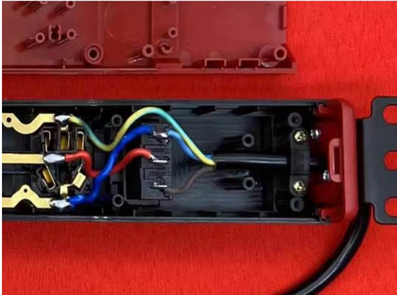
内部结构
