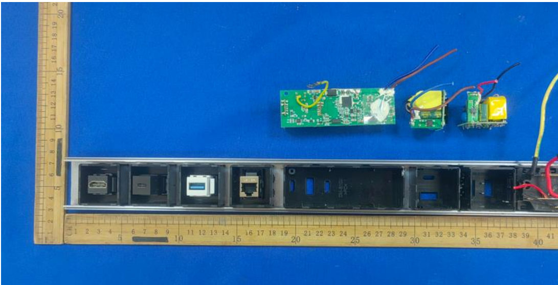
内部结构8 (搭配USB模块1+USB模块2+USB模块3+电信端口)
