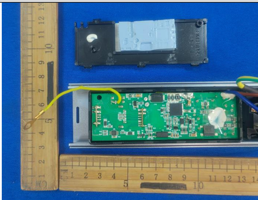
内部结构7 (搭配USB模块3)
