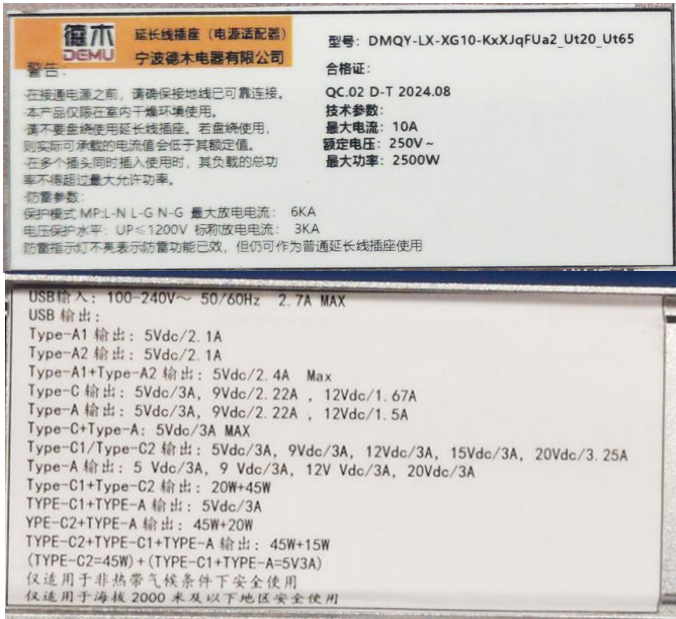
产品铭牌 (仅型号, 输入输出规格不同)
