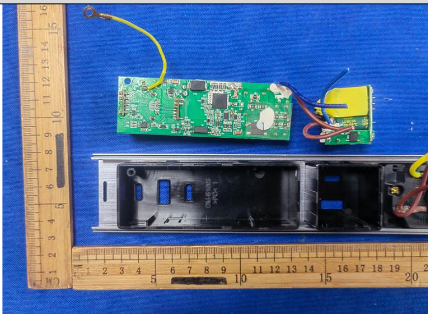
内部结构4 (搭配USB模块2+USB模块3)
