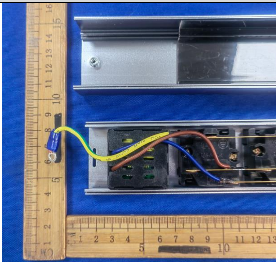
内部结构6 (搭配USB模块2)
