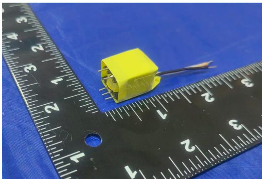
USB模块1变压器外观
