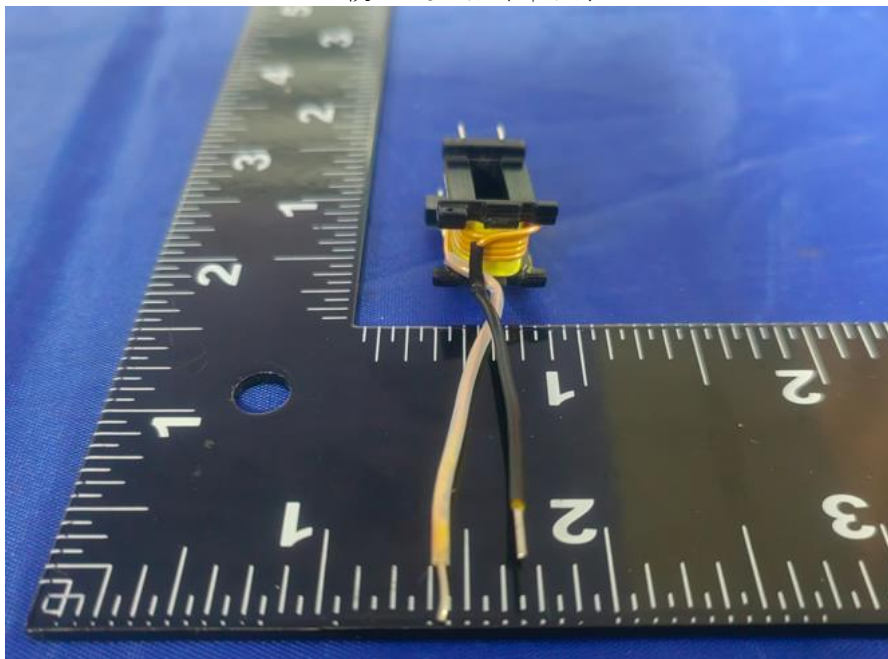
USB模块1变压器内部结构
