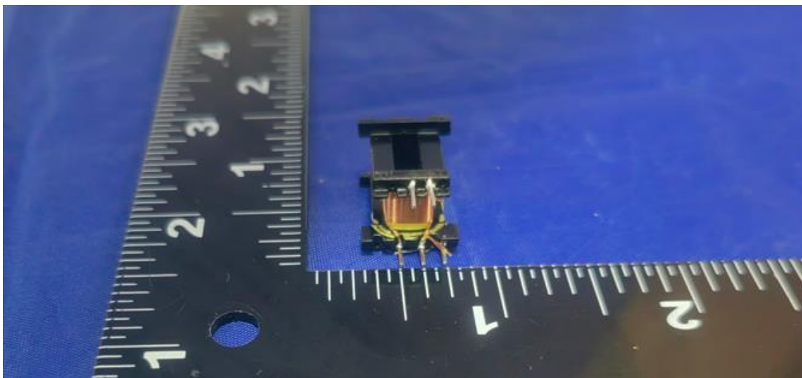
USB模块2变压器内部结构
