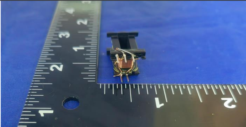
USB模块2变压器内部结构
