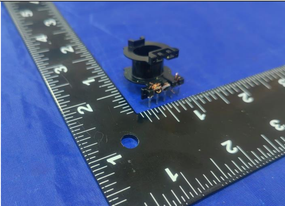
USB模块3变压器骨架
