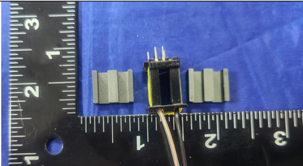
USB模块2变压器内部结构
