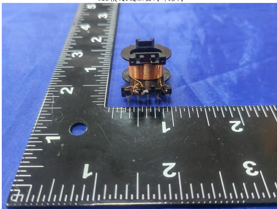
USB模块3变压器内部结构
