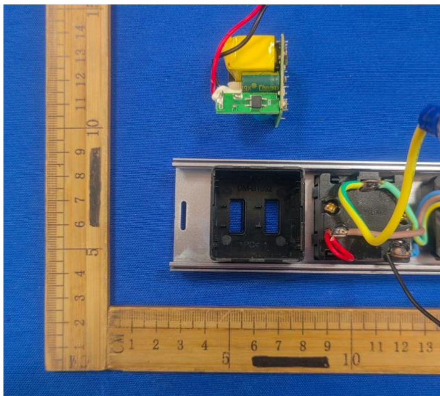
内部结构5 (搭配USB模块1)
