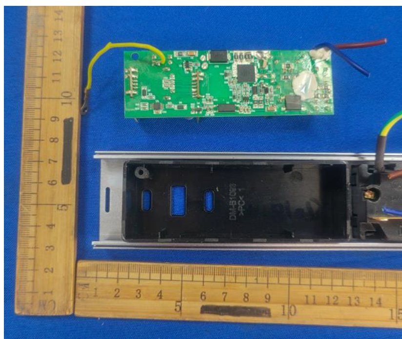
内部结构7 (搭配USB模块3)
