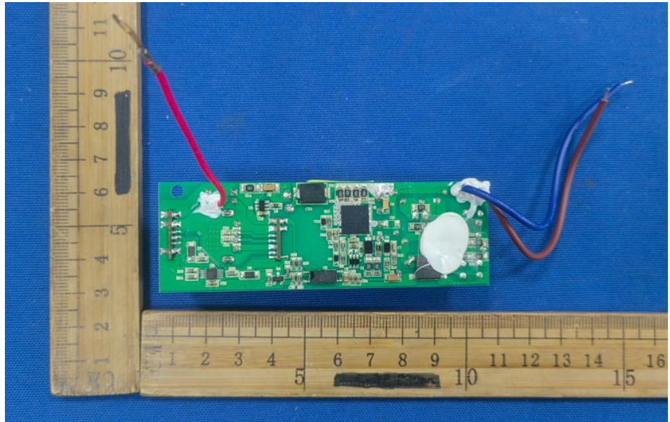
USB模块3反面
