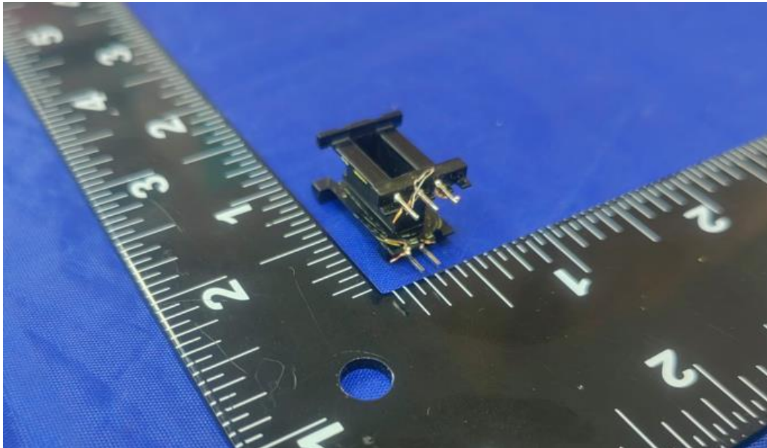
USB模块2变压器骨架
