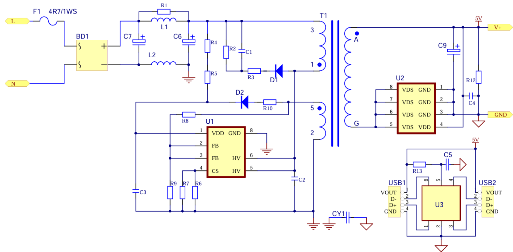
产品电气原理图：（USB模块1）
