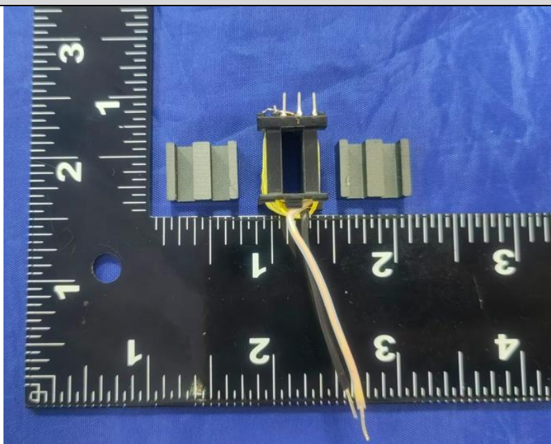
USB模块1变压器内部结构
