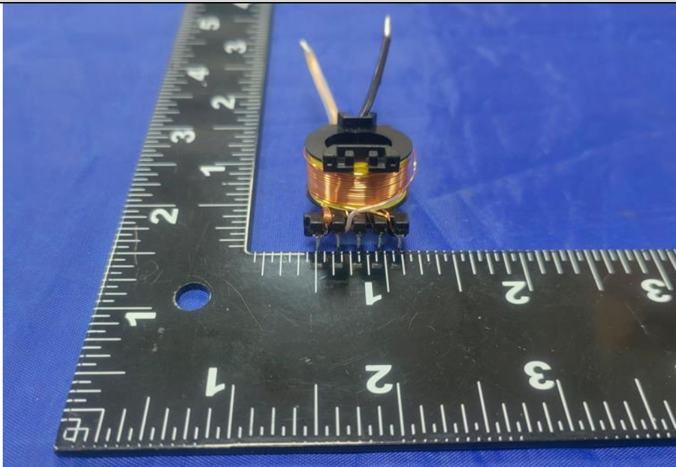
USB模块3变压器内部结构
