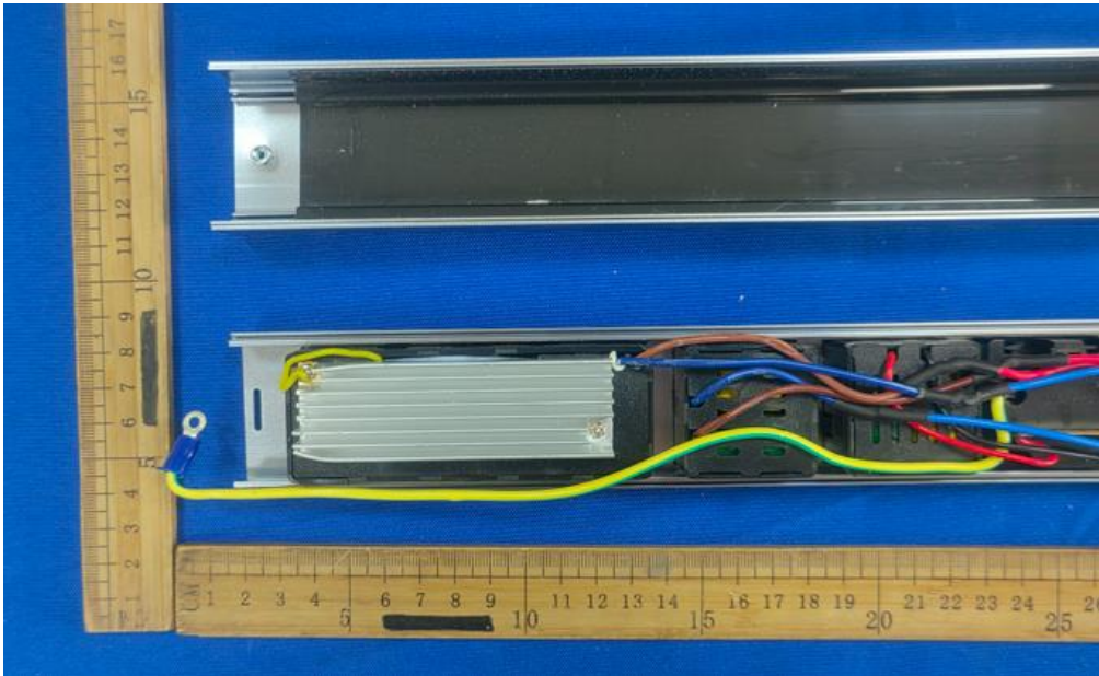
内部结构1（搭配USB模块1+USB模块2+USB模块3）
