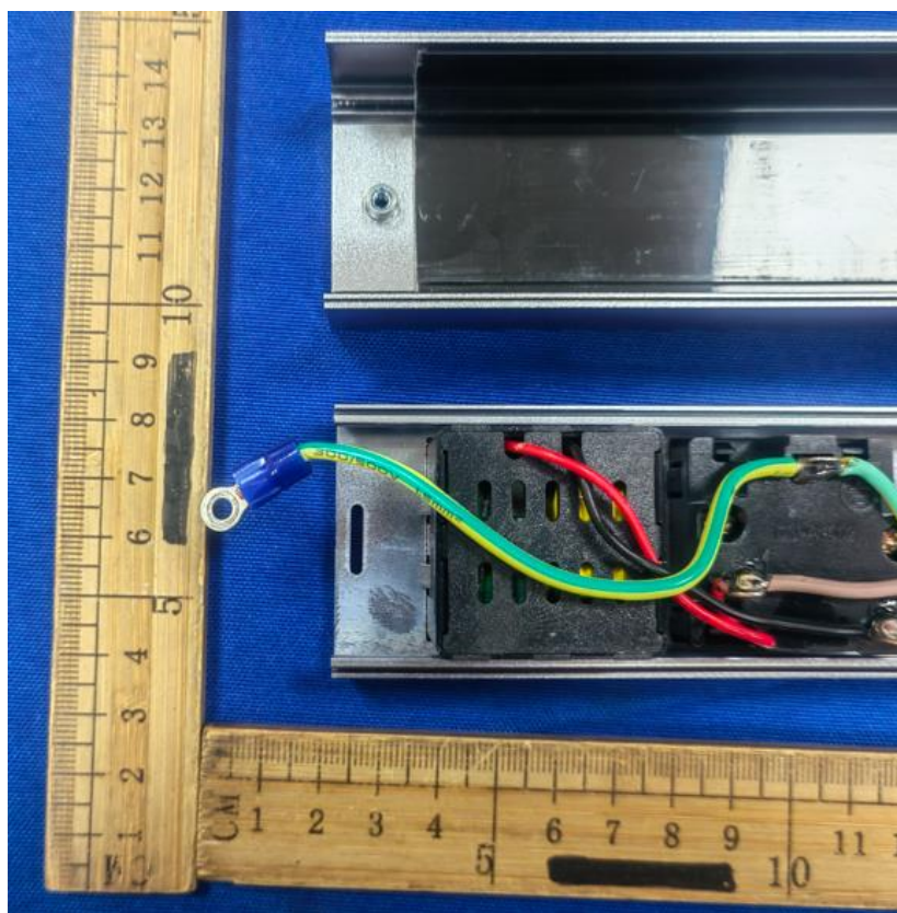
内部结构5 (搭配USB模块1)
