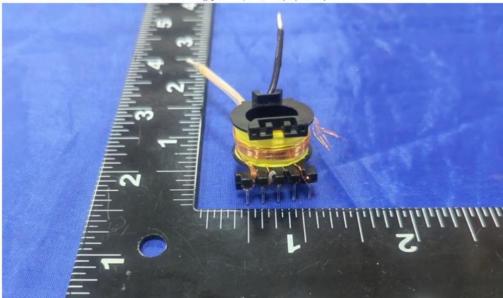
USB模块3变压器内部结构
