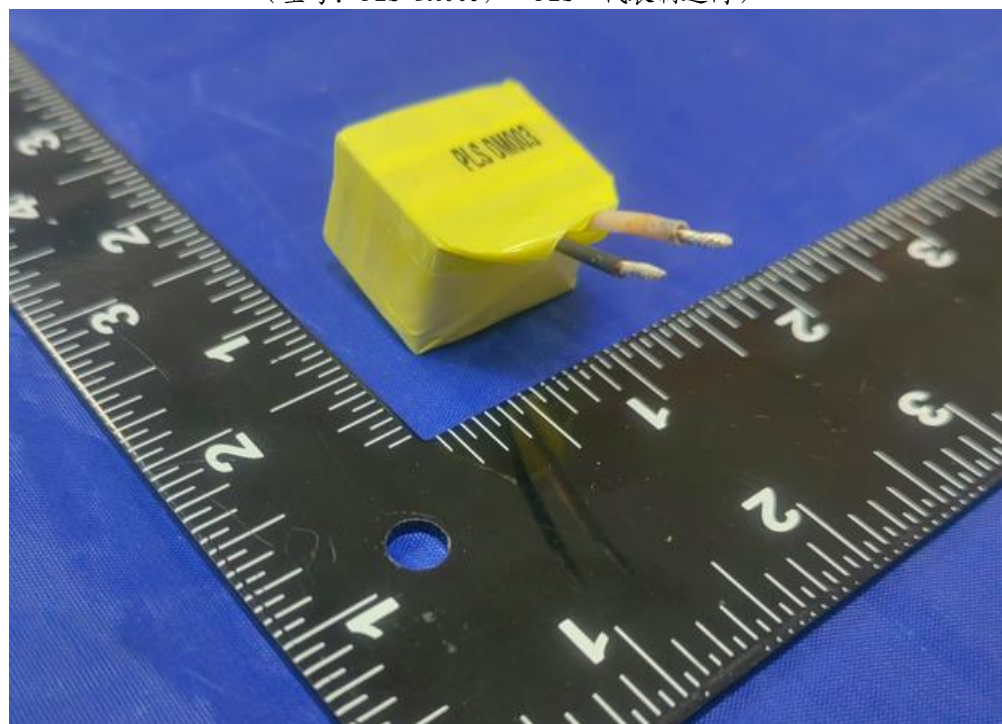
USB模块3变压器外观
