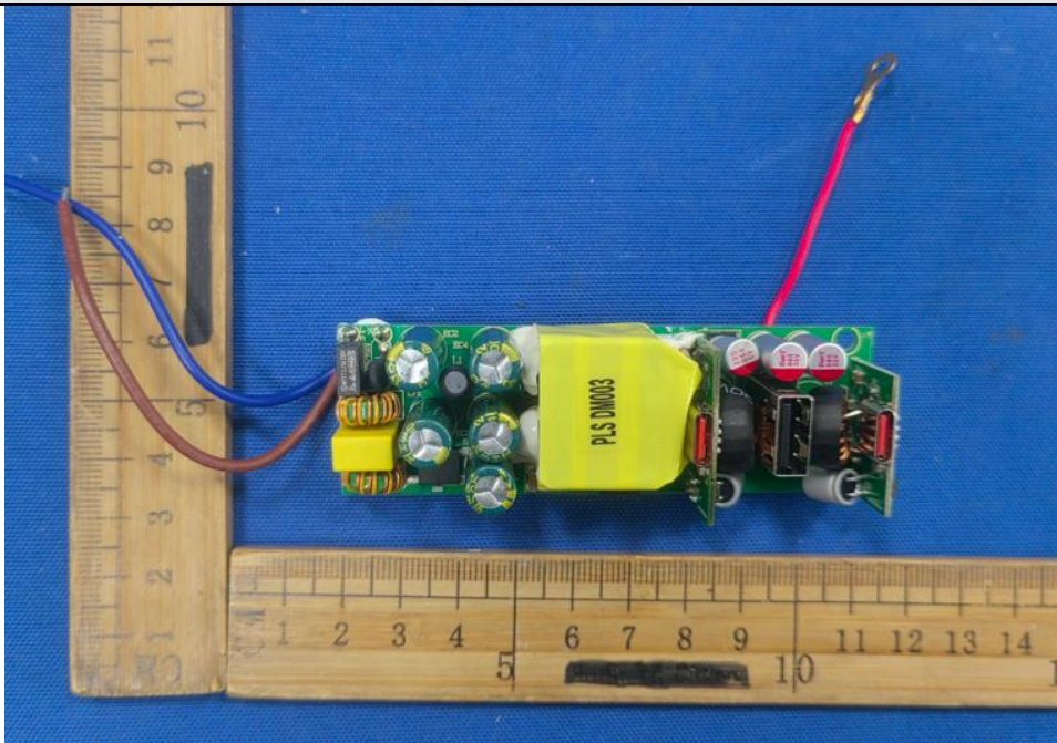
USB模块3正面
