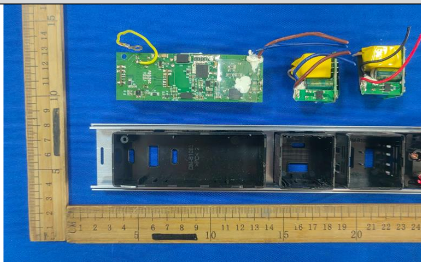
内部结构1 (搭配USB模块1+USB模块2+USB模块3)
