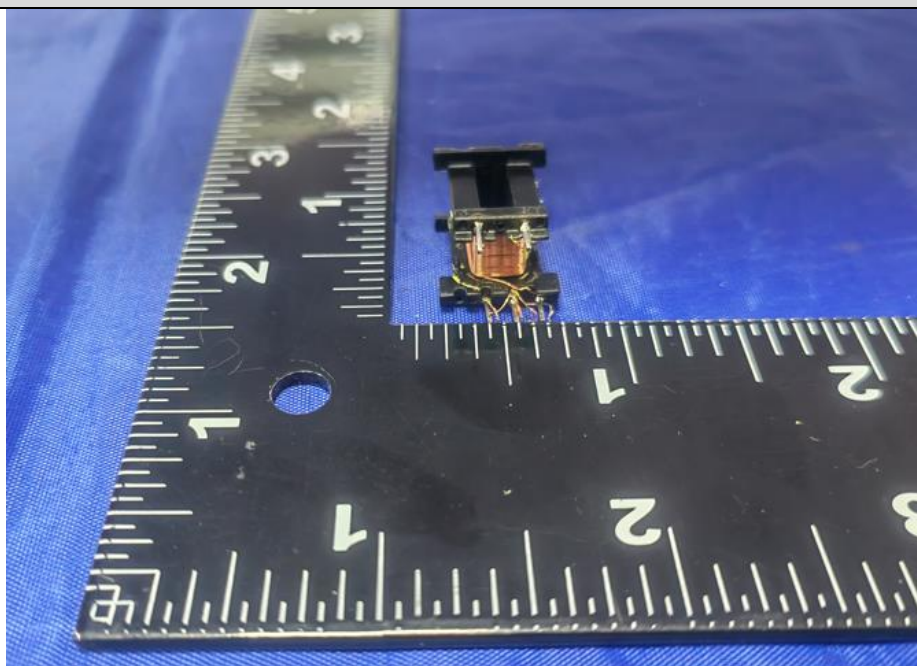
USB模块1变压器内部结构
