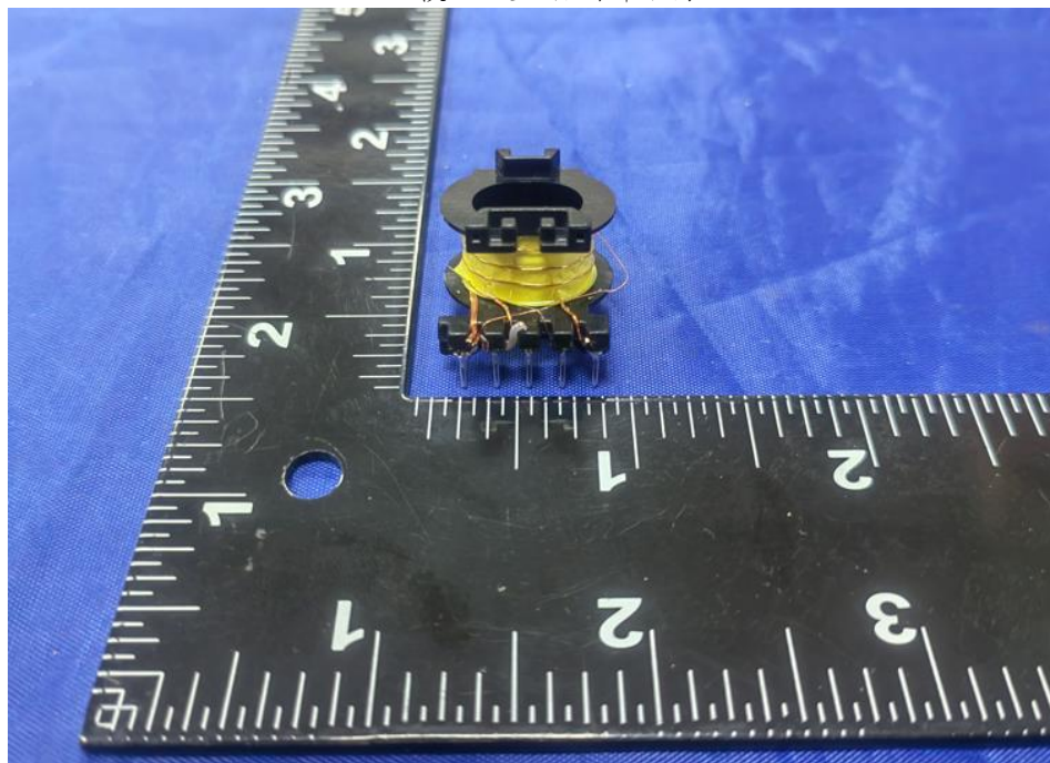
USB模块3变压器内部结构
