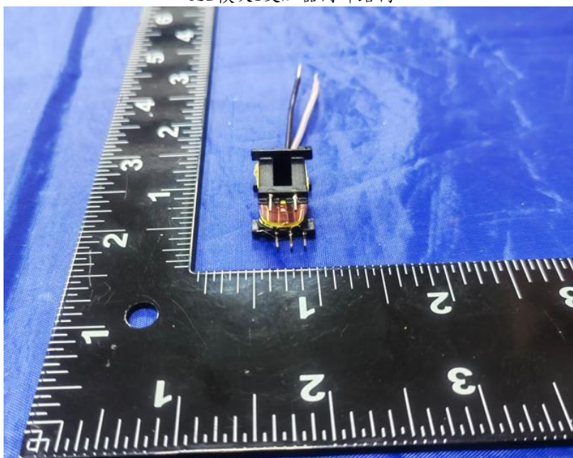
USB模块1变压器内部结构
