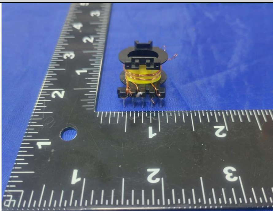
USB模块3变压器内部结构
