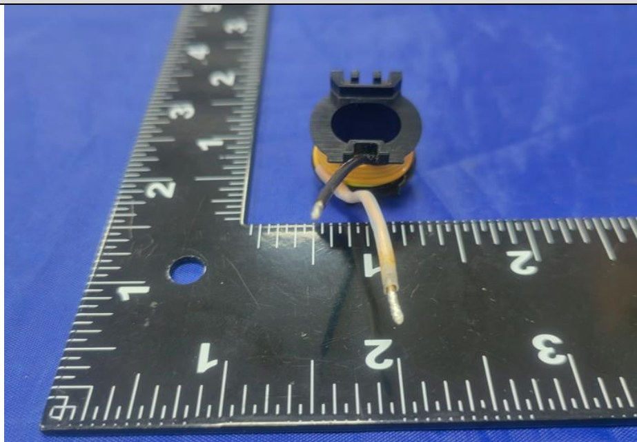
USB模块3变压器内部结构
