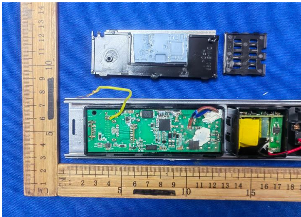
内部结构3 (搭配USB模块1+USB模块3)
