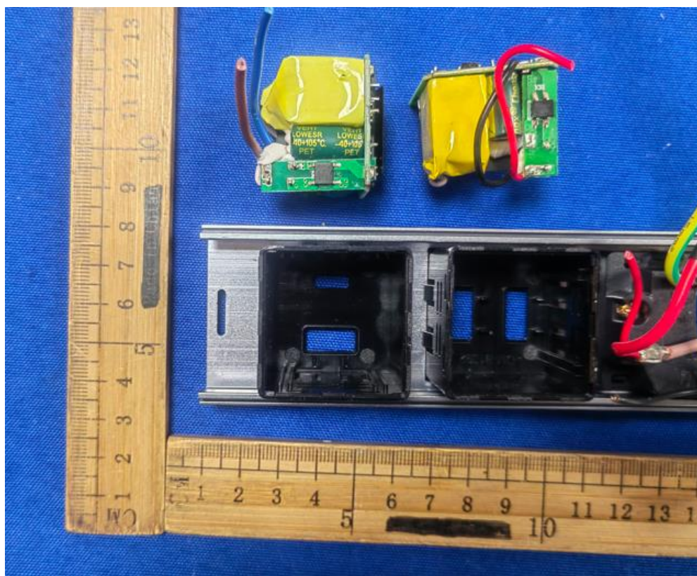
内部结构2 (USB模块1+USB模块2)
