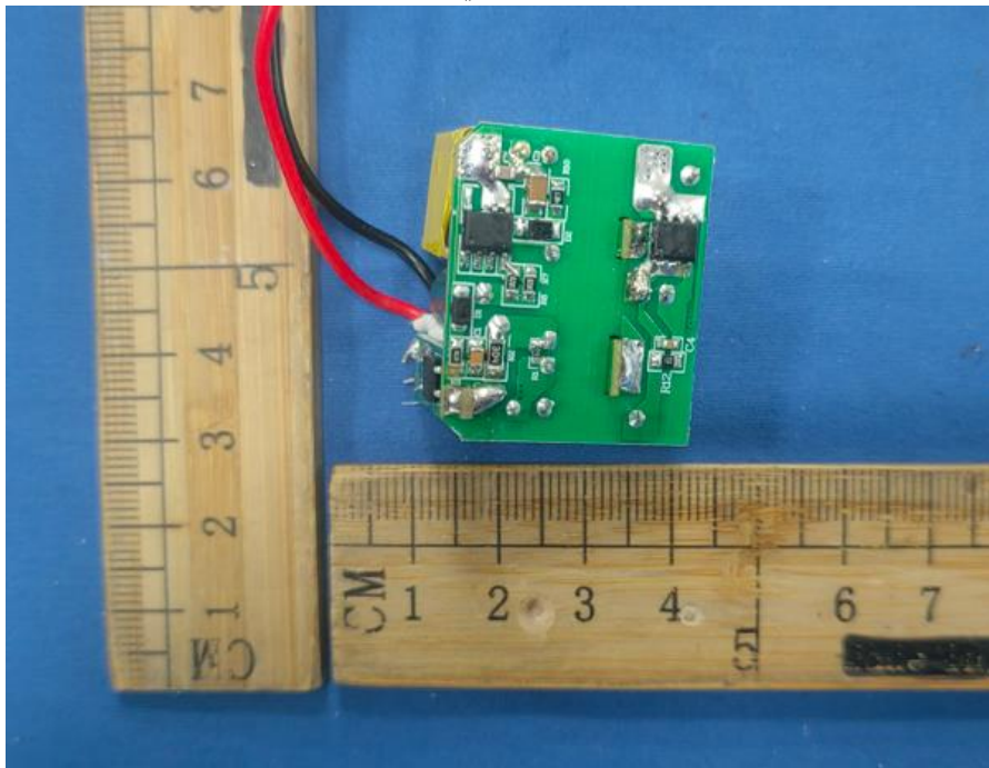
USB模块1反面
