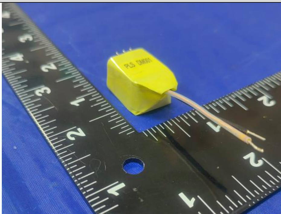
USB模块1变压器外观
