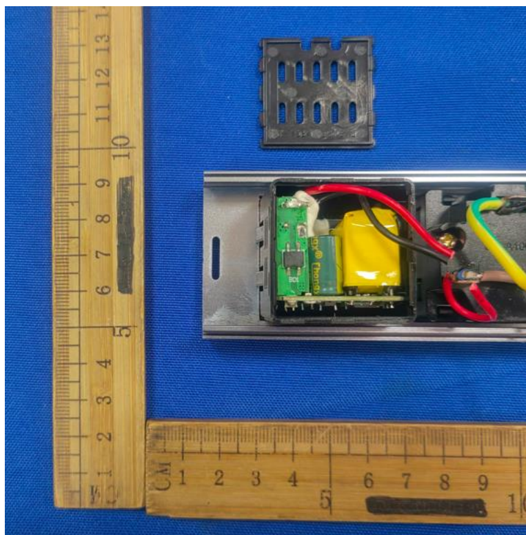
内部结构2 (USB模块1)
