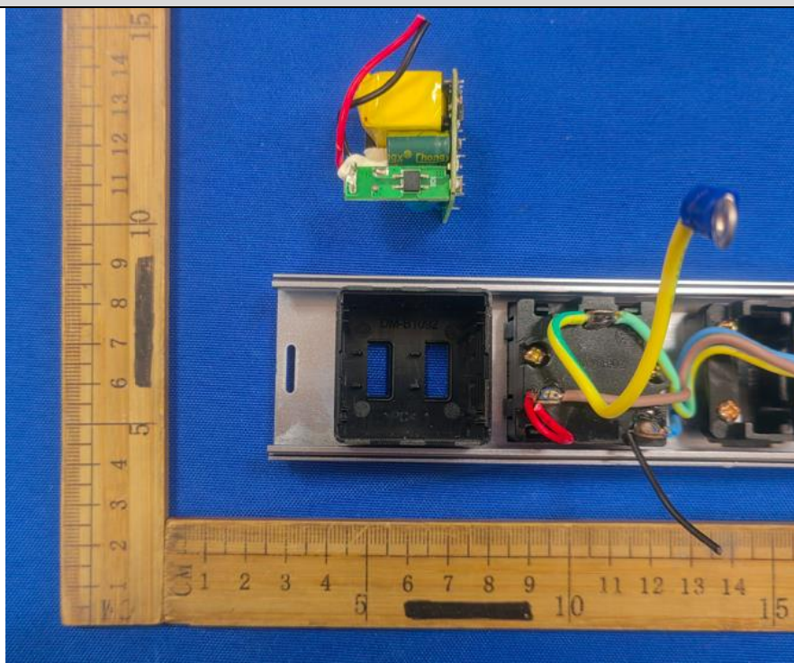
内部结构2 (USB模块1)
