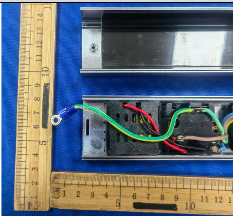
内部结构2 (USB模块1)
