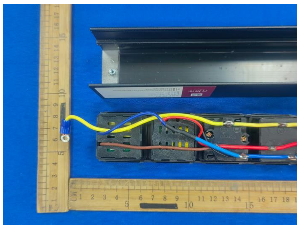
内部结构1 (USB模块1+USB模块2)
