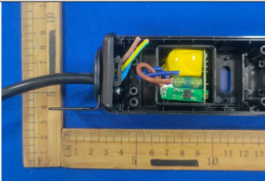
内部结构3 (USB模块2)
