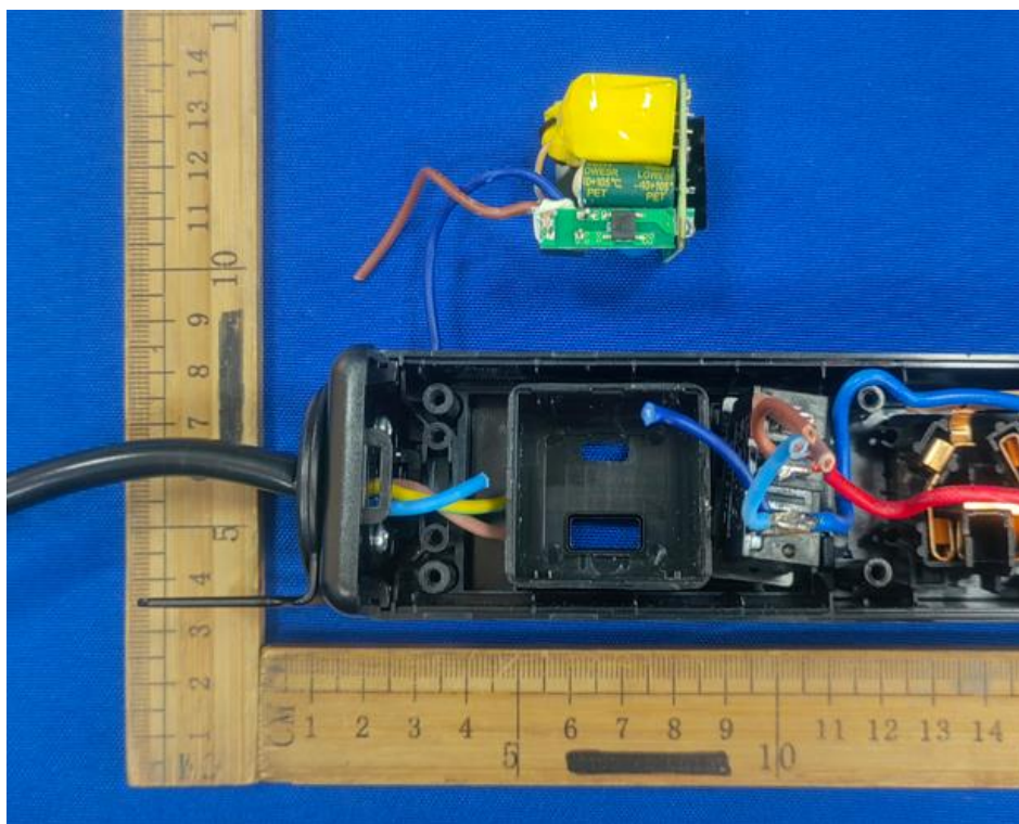
内部结构3 (USB模块2)
