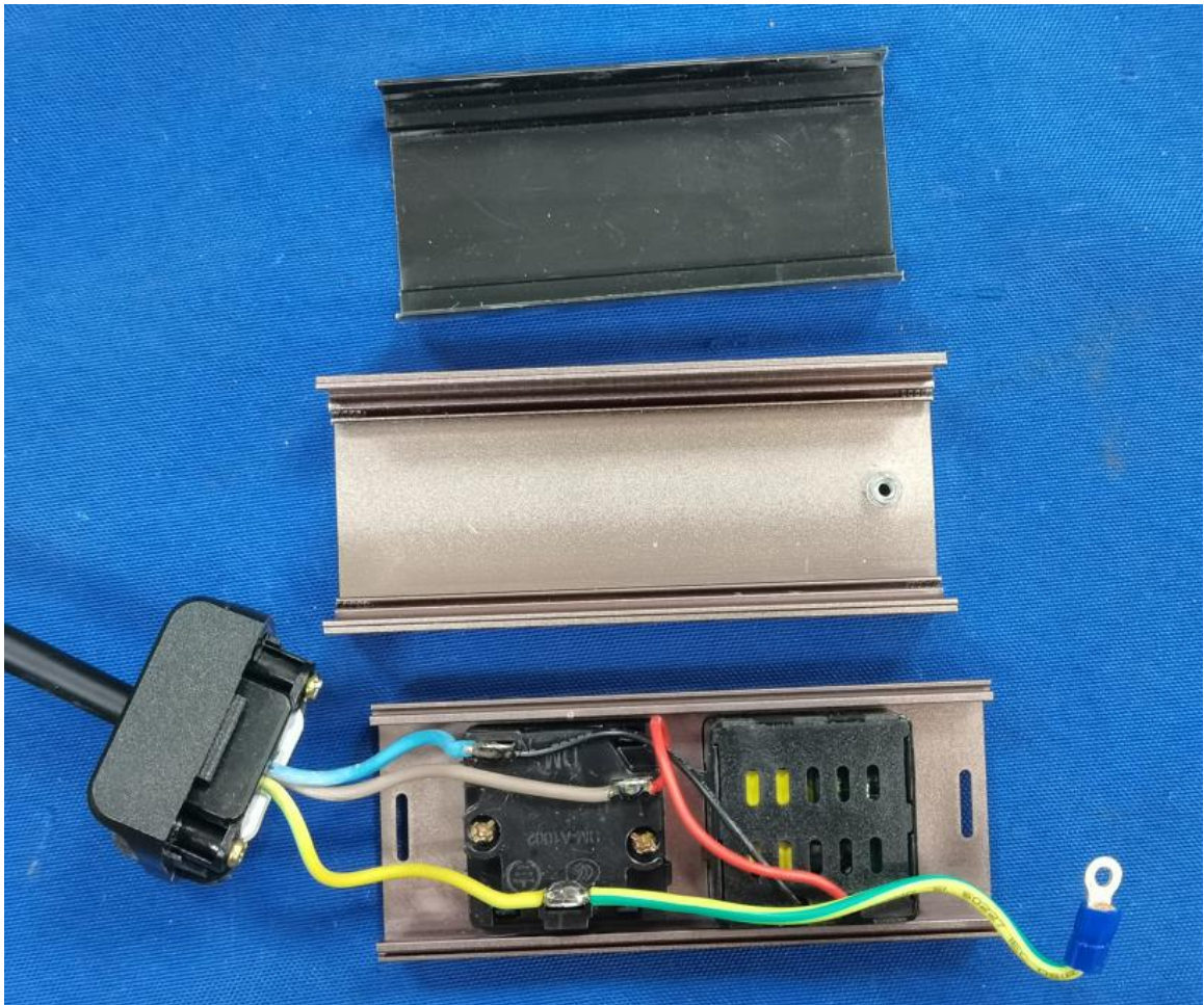
DMQY-LX-XG1-Ua2 内部结构
