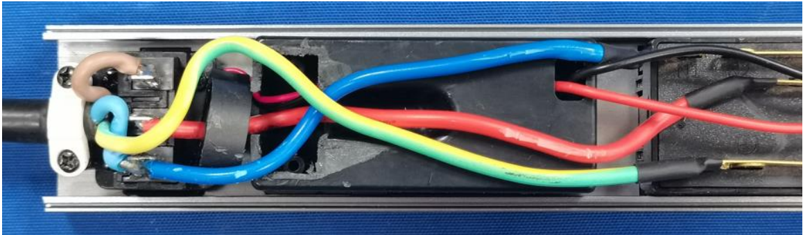
DMQY-TY16-XG20-KxXJqFUa2_Ut20_Ut65 内部结构
