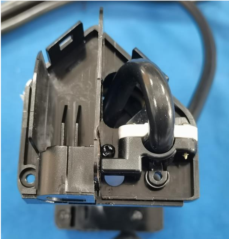
DMQY-ZM-XG1-Ua2 导线固定装置
