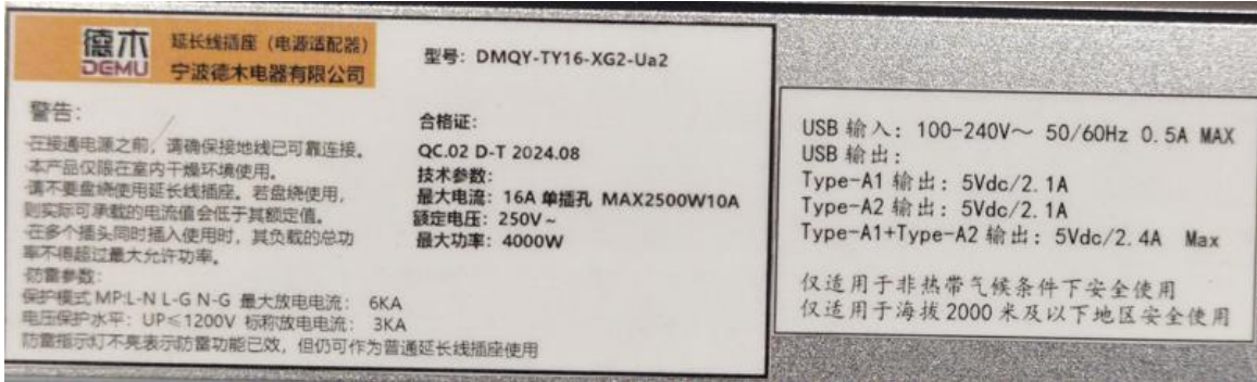
DMQY-TY16-XG2-Ua2 标志
