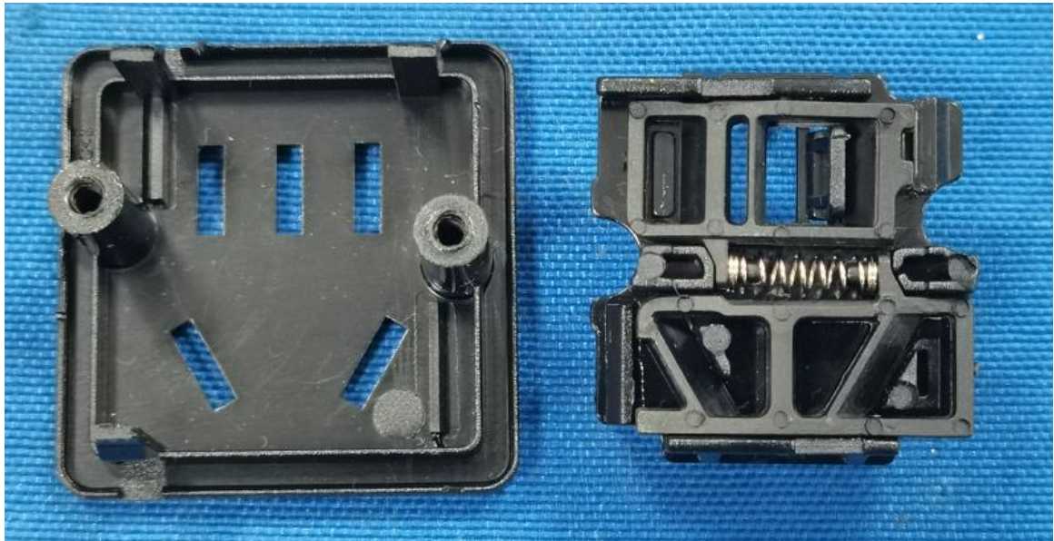
DMQY-TY16-XG20-KxXJqFUa2_Ut20_Ut65 内部结构
