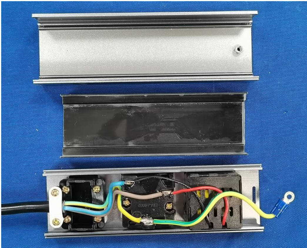
DMQY-TY10-XG1-Ua2 内部结构
