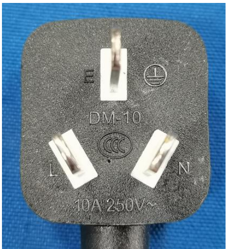
DMQY-LX-XG10-KxXJqFUa2_Ut20_Ut65 插头
