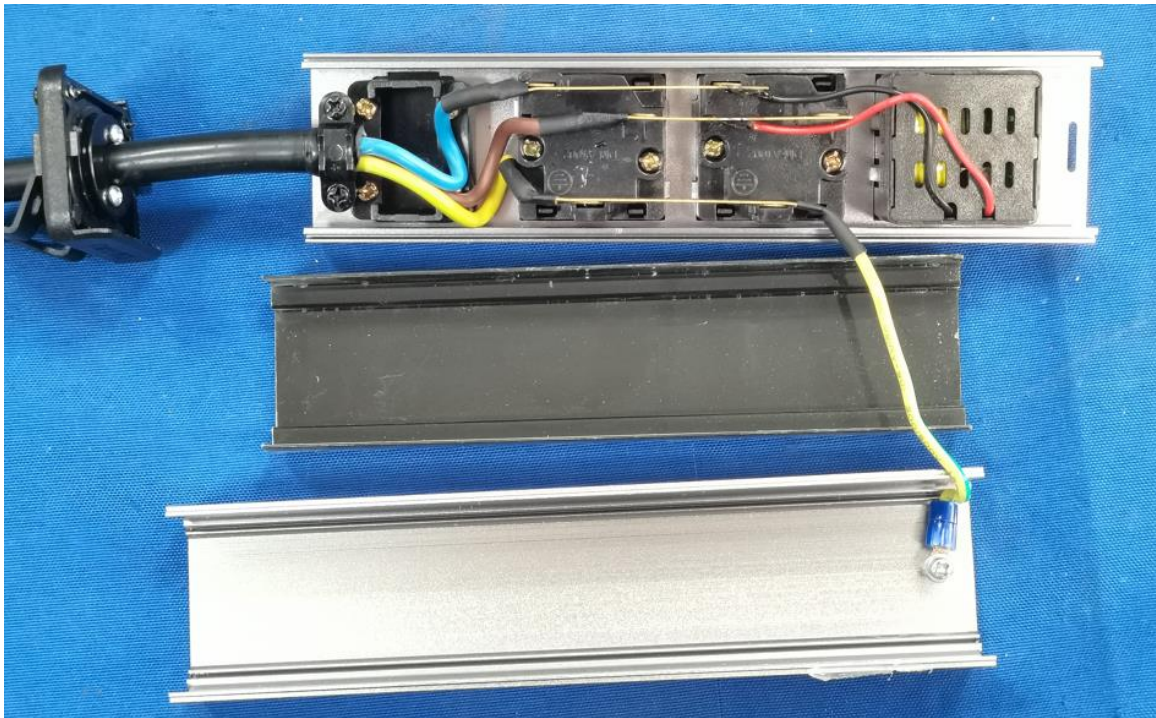
DMQY-TY16-XG2-Ua2 内部结构
