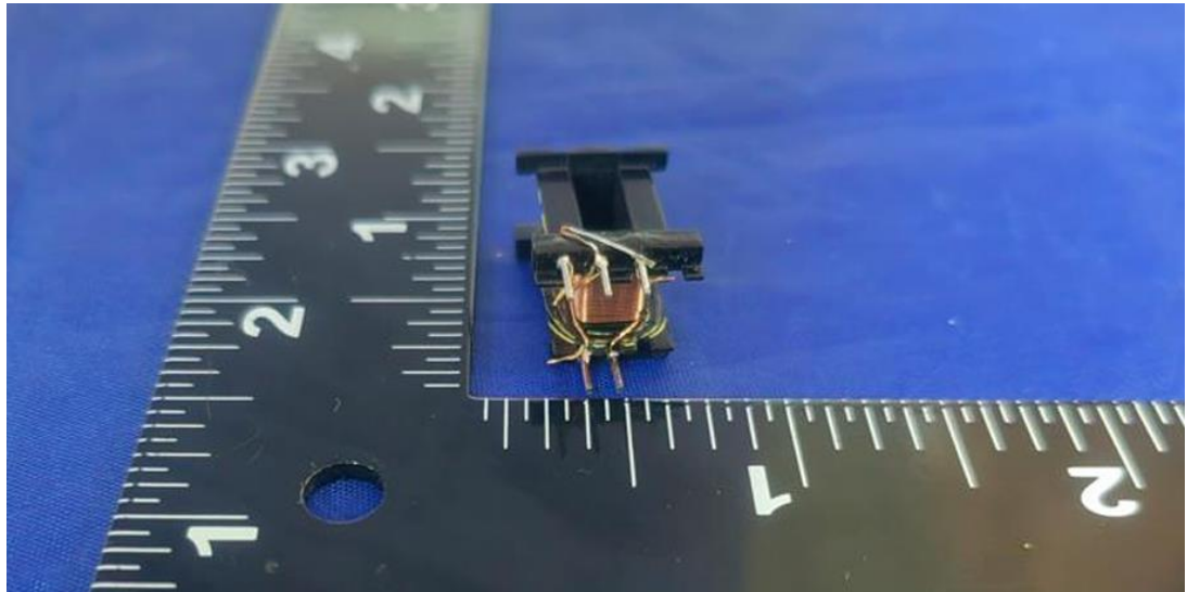
USB模块2变压器内部结构
