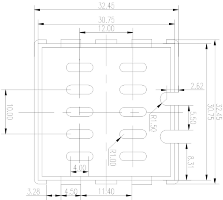
绝缘挡板尺寸 (用于USB模块1和USB模块2)
