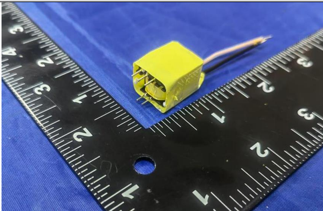
USB模块2变压器外观
