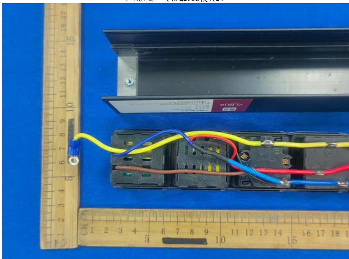
内部结构1 (USB模块1+USB模块2)
