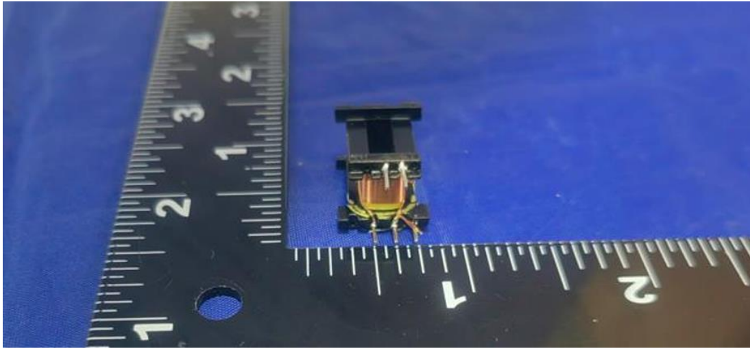
USB模块2变压器内部结构
