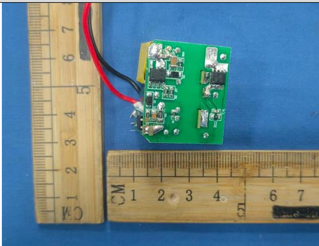
USB模块1反面
