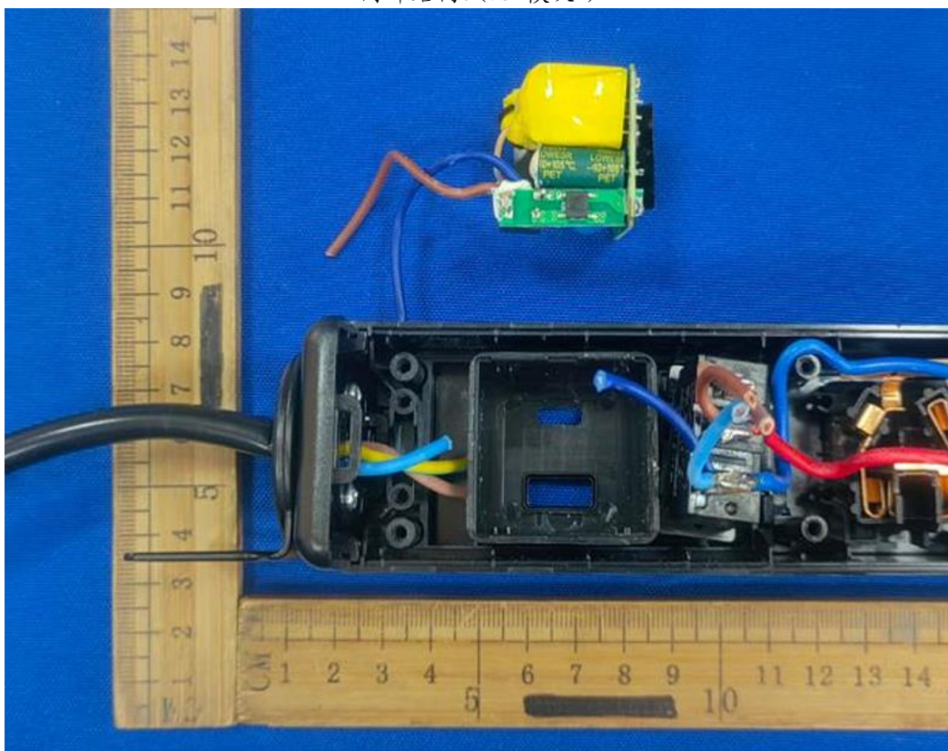
内部结构3 (USB模块2)
