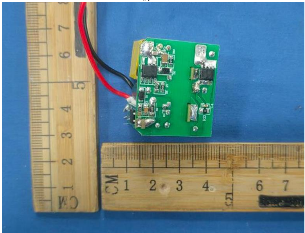
USB模块1反面
