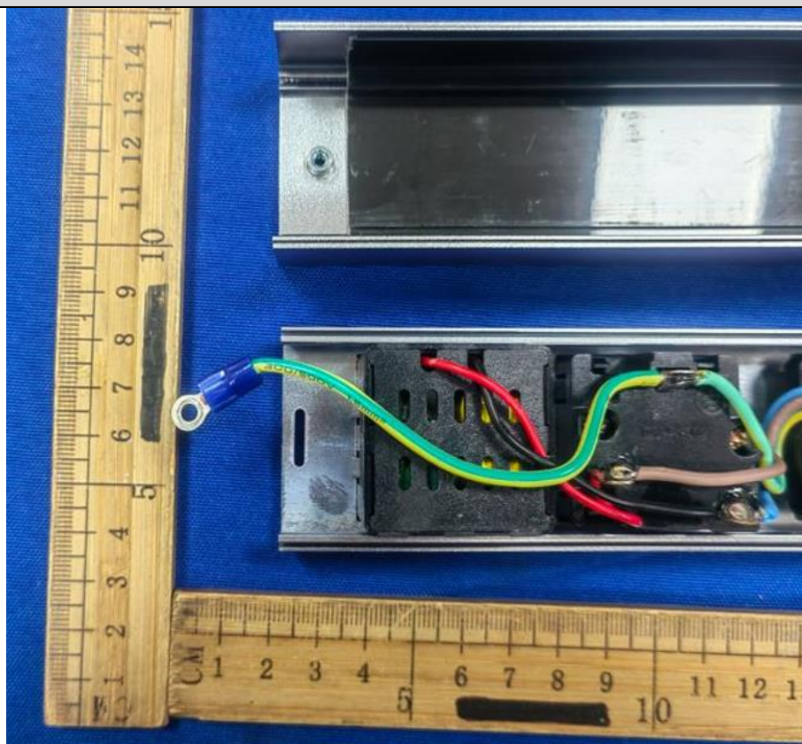
内部结构2 (USB模块1)
