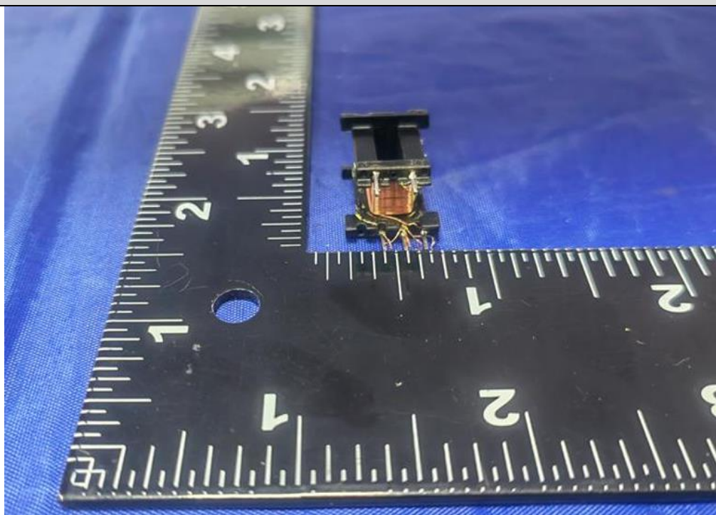
USB模块1变压器内部结构
