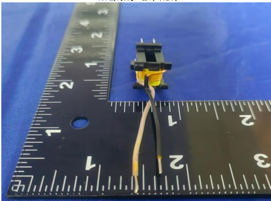
USB模块1变压器内部结构
