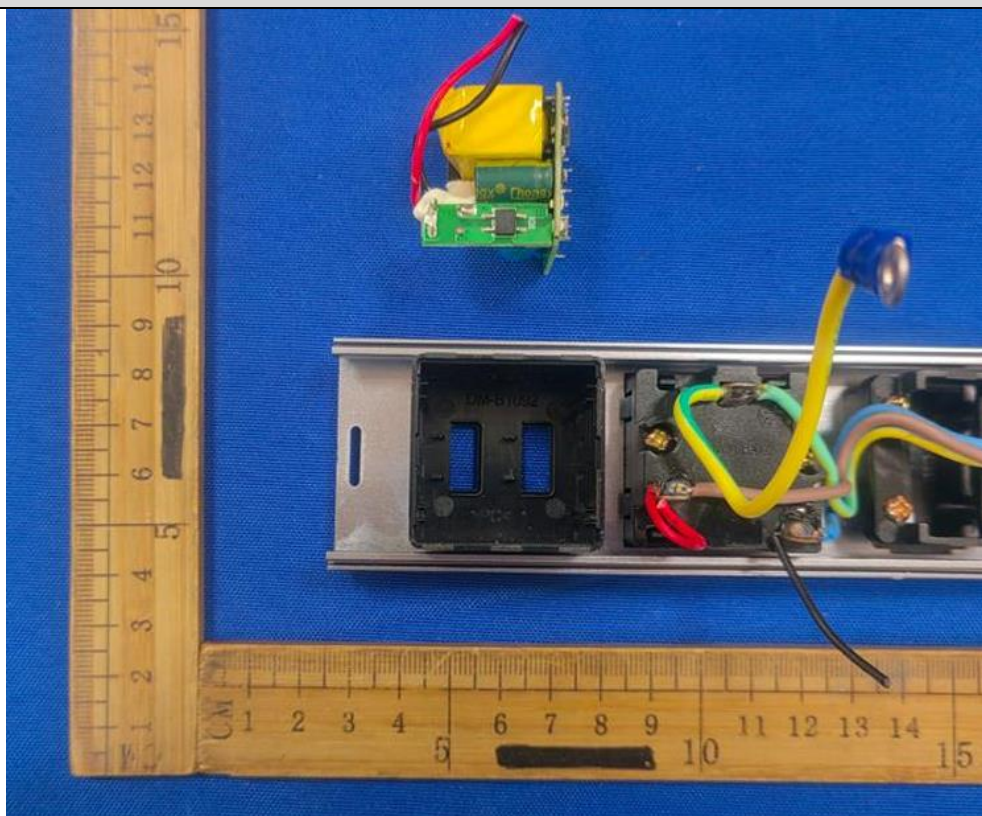
内部结构2 (USB模块1)
