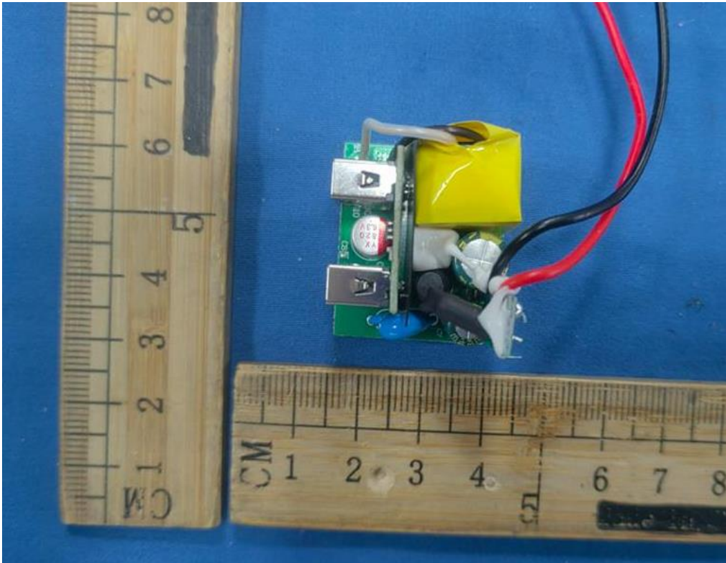
USB模块1正面
