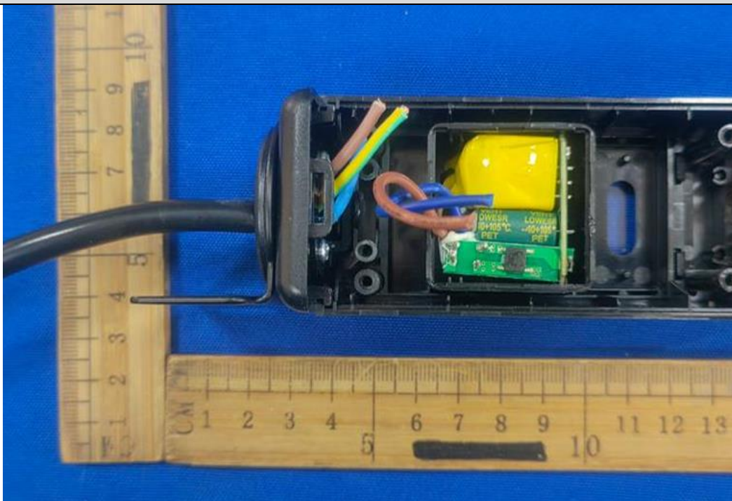
内部结构3 (USB模块2)
