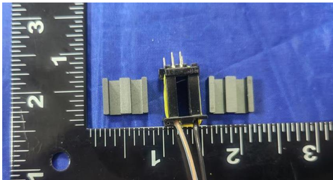
USB模块2变压器内部结构
