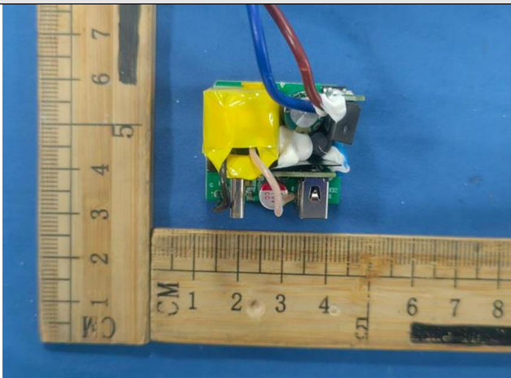
USB模块2正面
