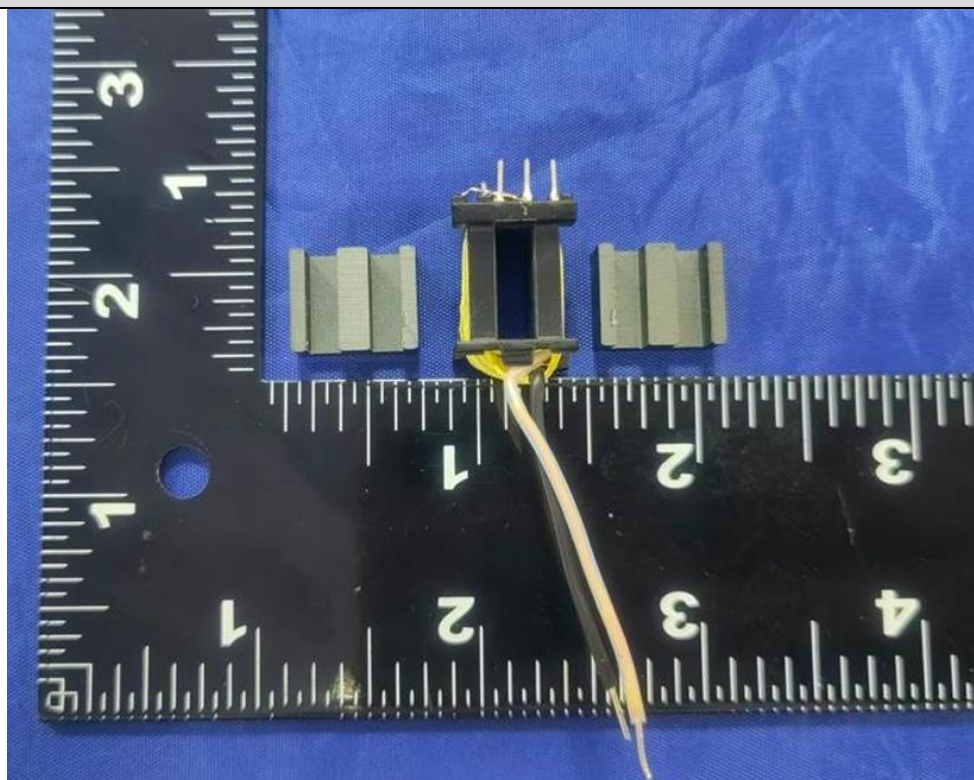
USB模块1变压器内部结构
