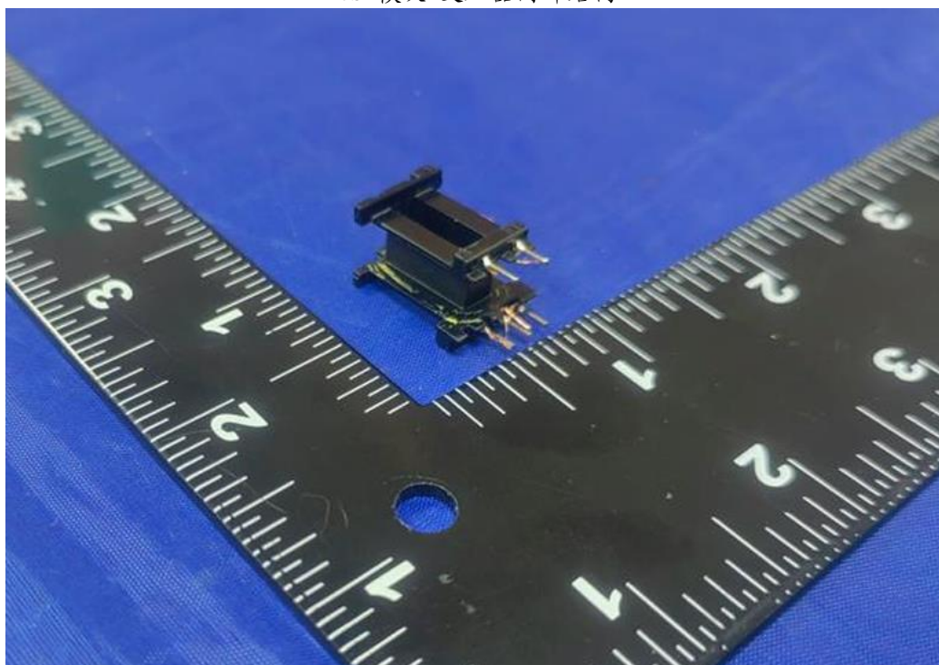
USB模块1变压器骨架
