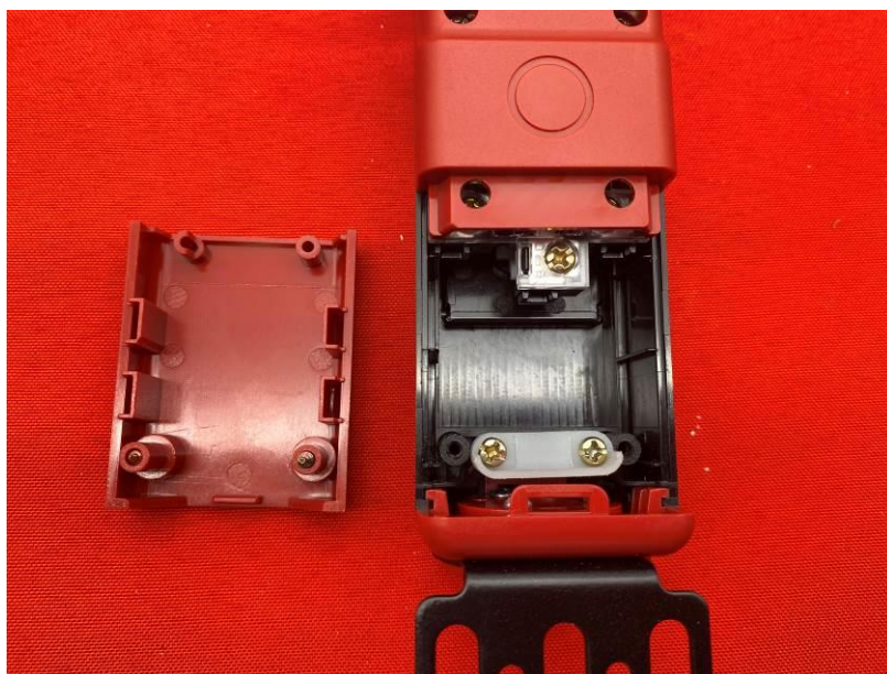
内部结构 (接线端子)
