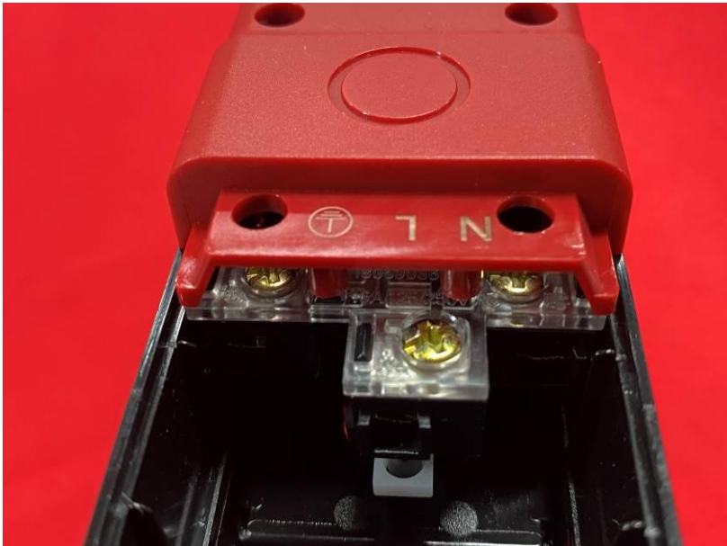
铭 牌（接线端子）
