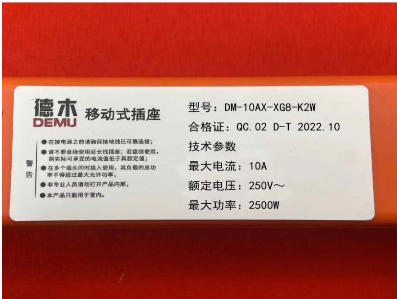
铭 牌
