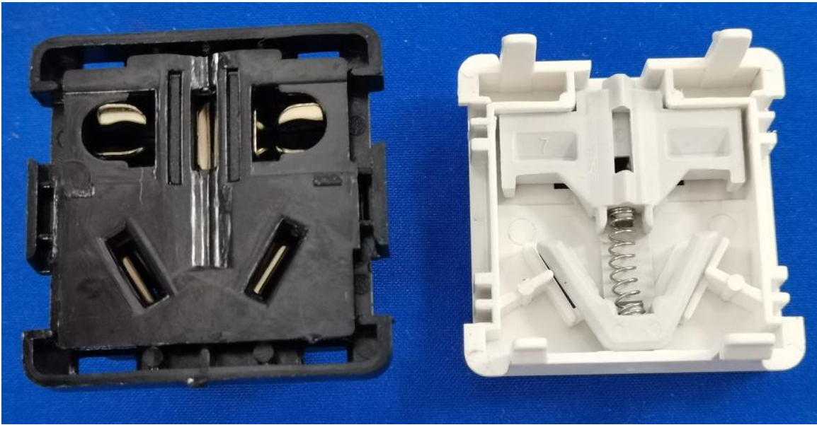
DM-10-XG6-KU4(白) 插座功能件
