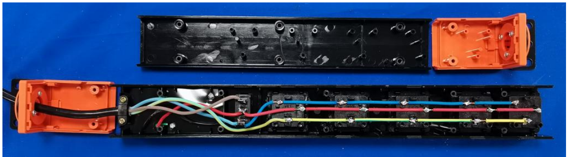
DM-10-XG5-KU4(黑) 内部结构
