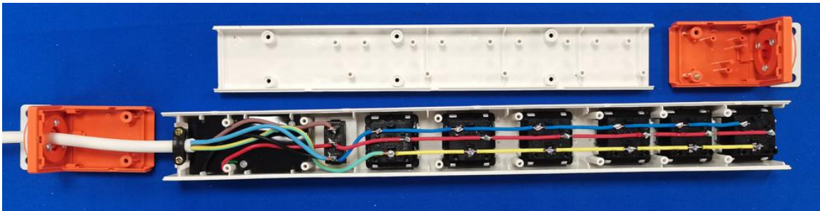
DM-10-XG6-KU4(白) 内部结构
