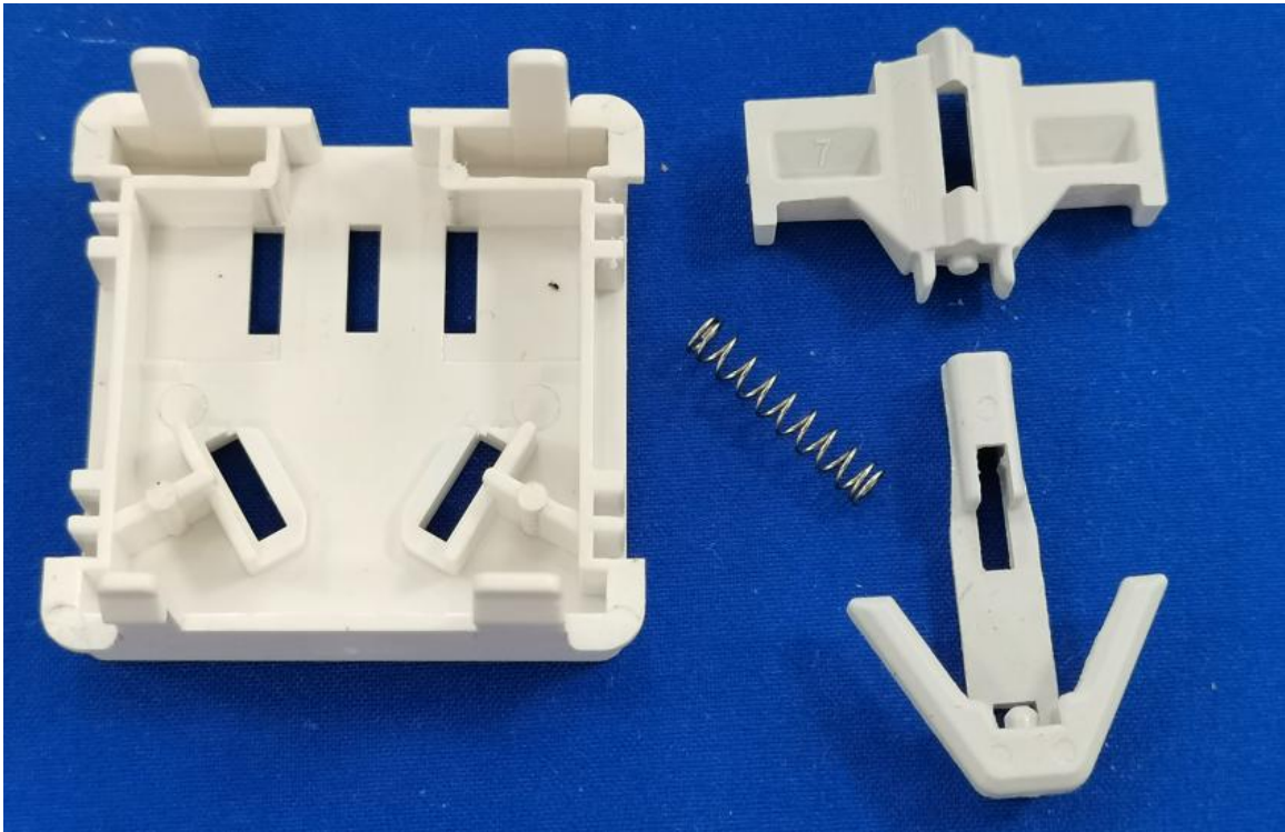
DM-10-XG6-KU4(白) 内部结构
