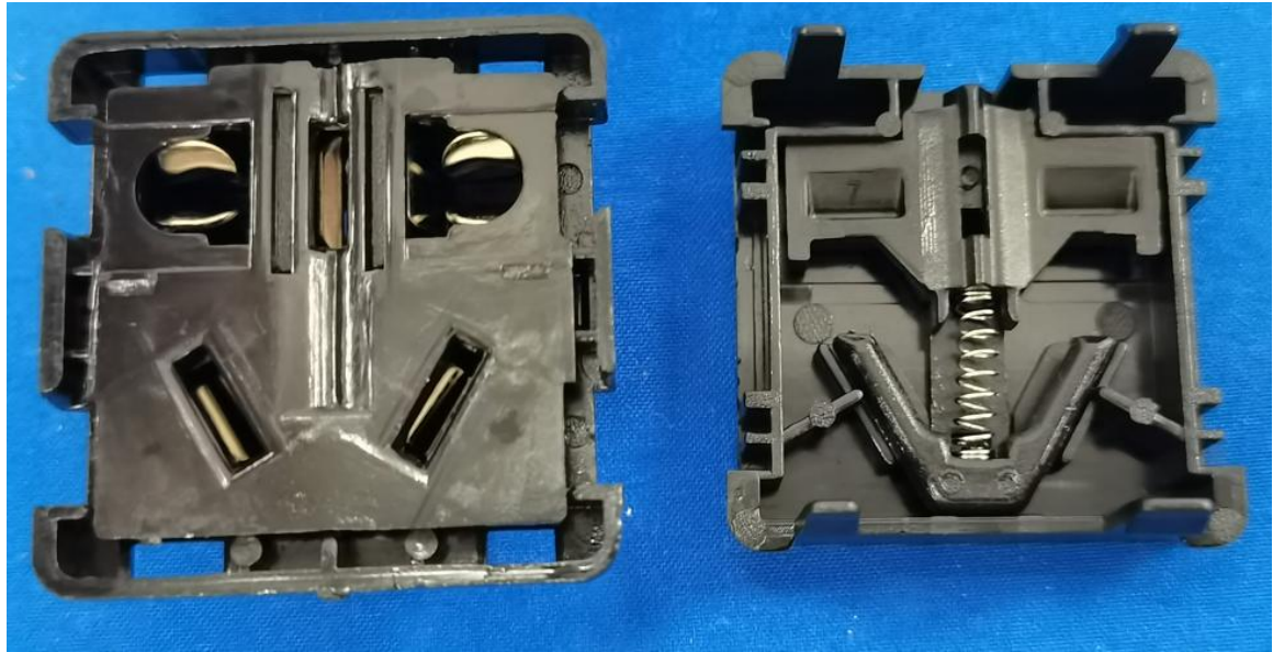
DM-10-XG6-KU4 (黑) 插座功能件
