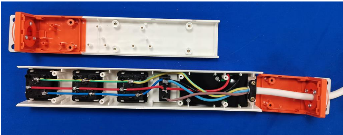
DM-10-XG3-KU4(白) 内部结构
