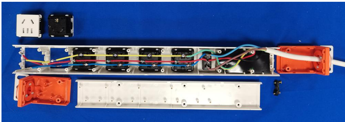
DM-10-XG6-KU4(白) 内部结构
