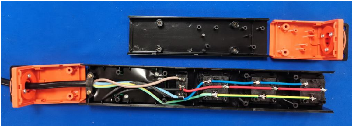
DM-10-XG3-KU4(黑) 内部结构
