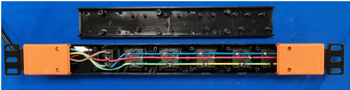
DM-10-XG6-KU4(黑) 内部结构
