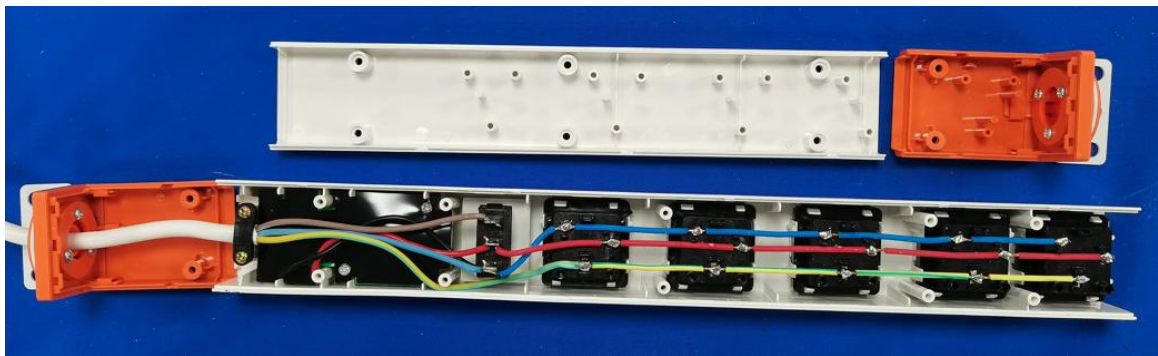
DM-10-XG5-KU4(白) 内部结构
