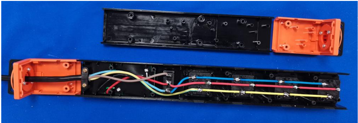
DM-10-XG4-KU4(黑) 内部结构
