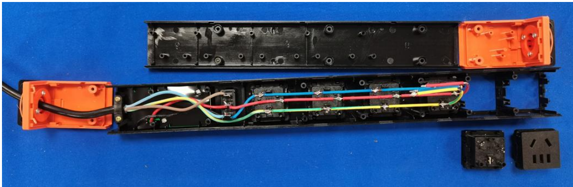
DM-10-XG6-KU4(黑) 内部结构
