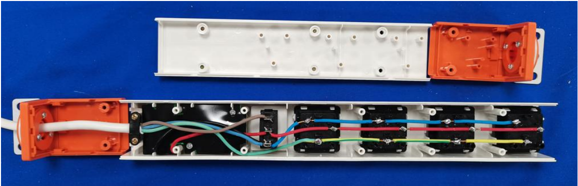
DM-10-XG4-KU4(白) 内部结构
