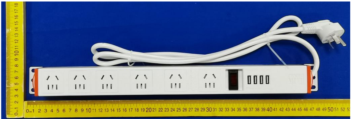
DM-10-XG6-KU4(白) 外观
