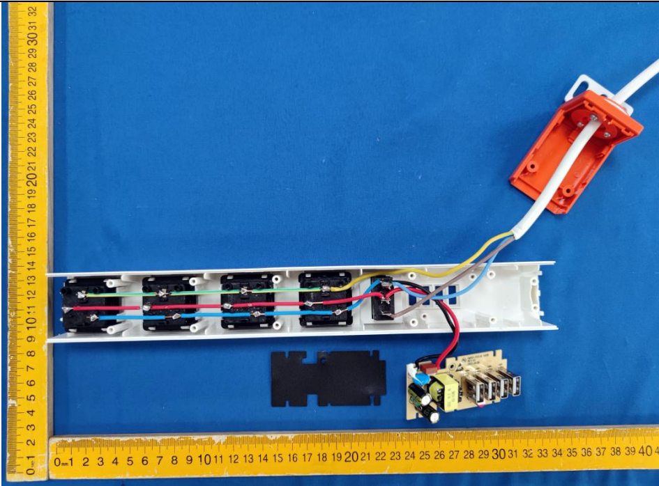
内部结构
