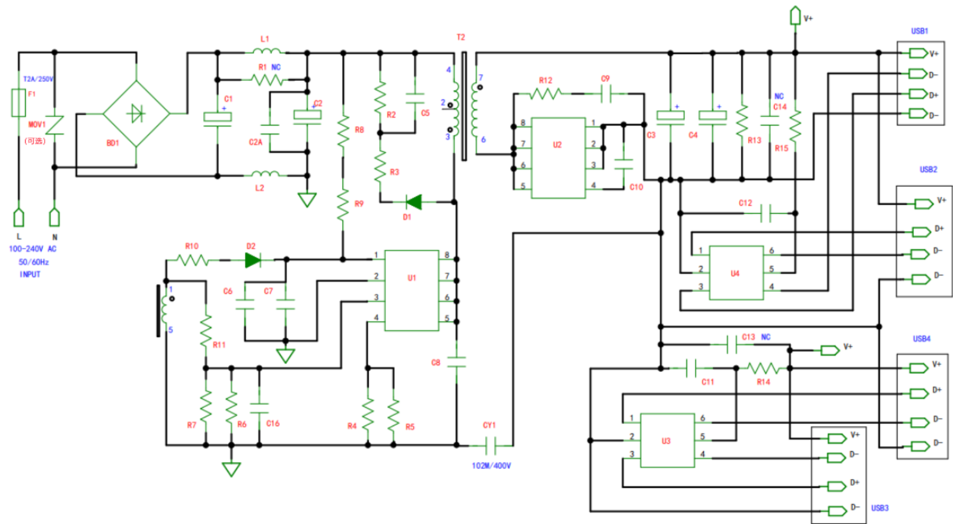
产品电气原理图: USB模块1 (结构一)
