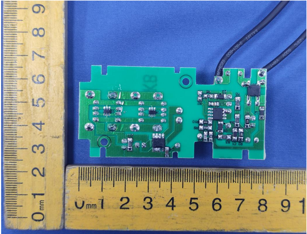
USB2模块背面
