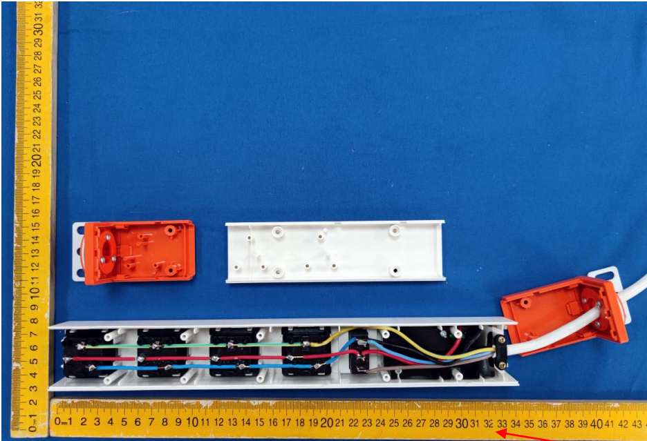
内部结构 (箭头所指为USB模块位置, 绝缘垫片位于其背部)
