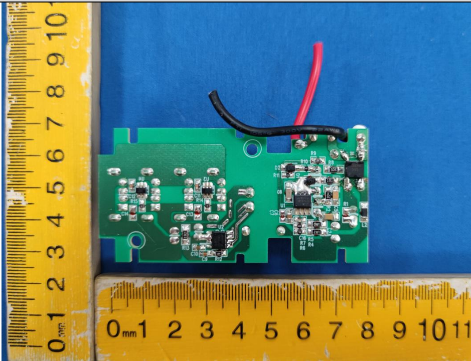
USB1模块背面 (结构一)
