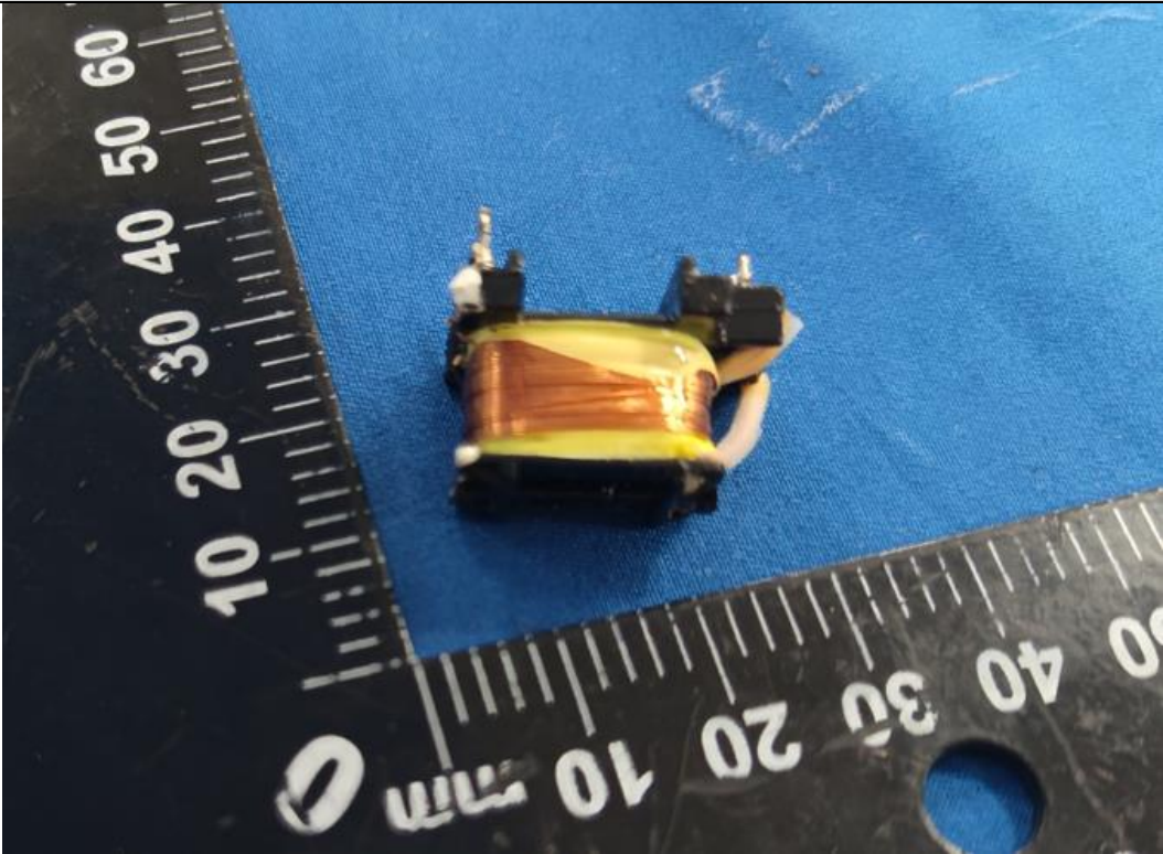
变压器内部结构 (初级绕组)
