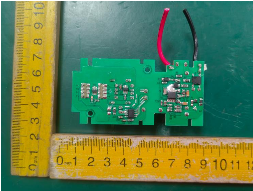
USB1模块背面（结构二） 本次增加
