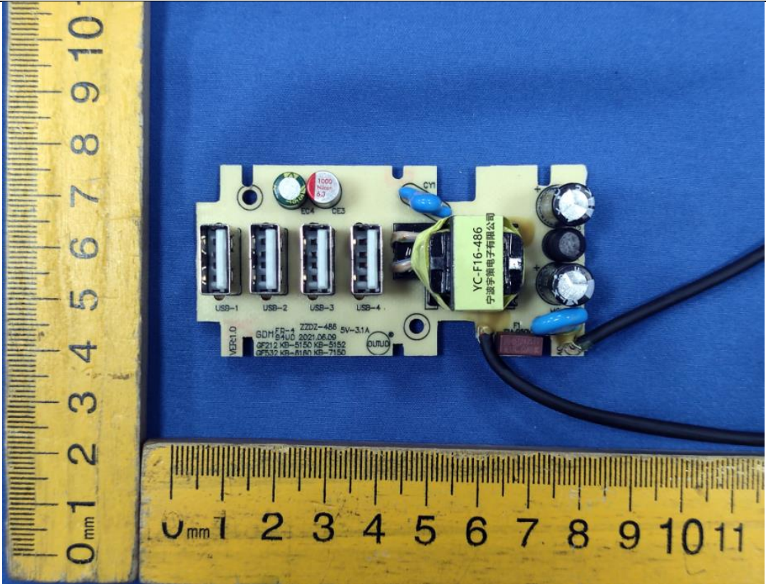
USB2模块正面
