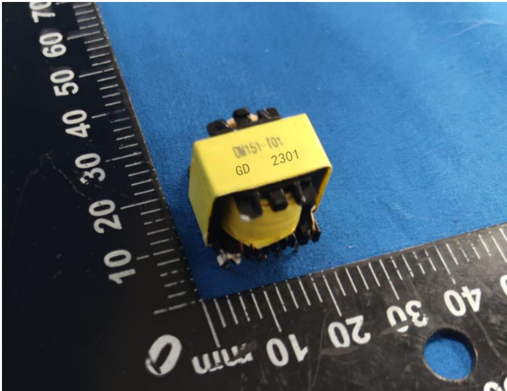
变压器外观
