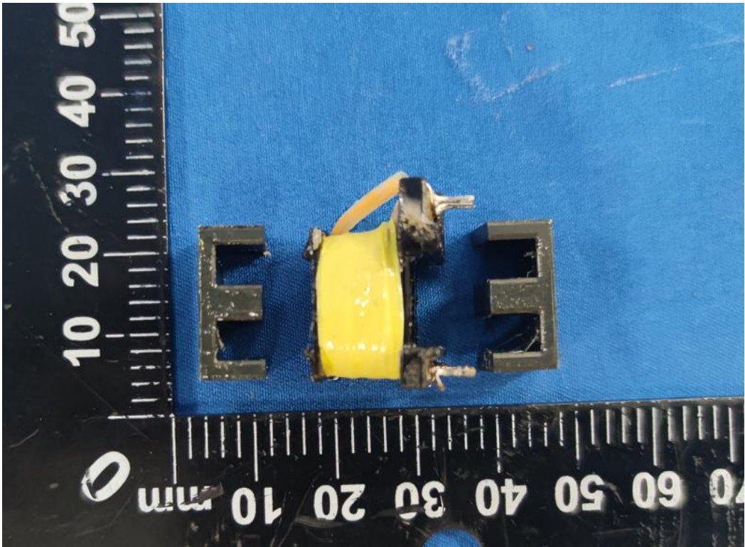
变压器内部结构
