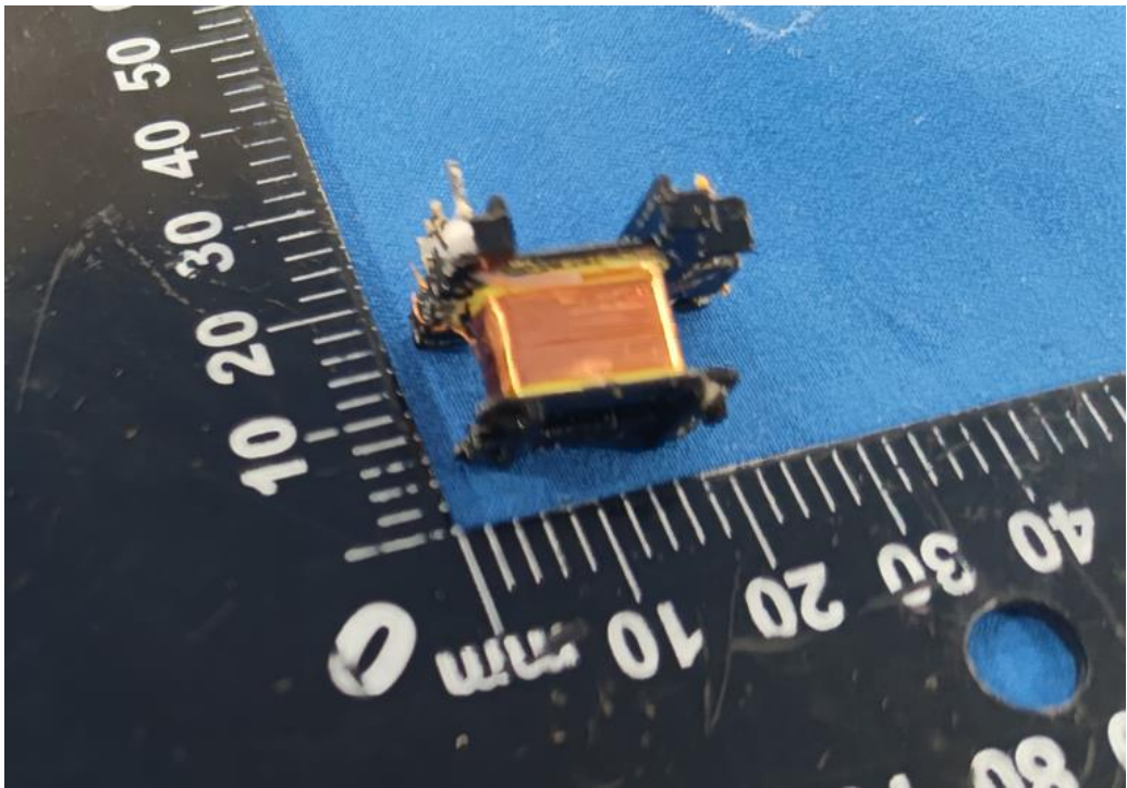
变压器内部结构 (初级绕组)
