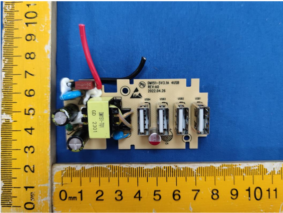
USB1模块正面 (结构一)
