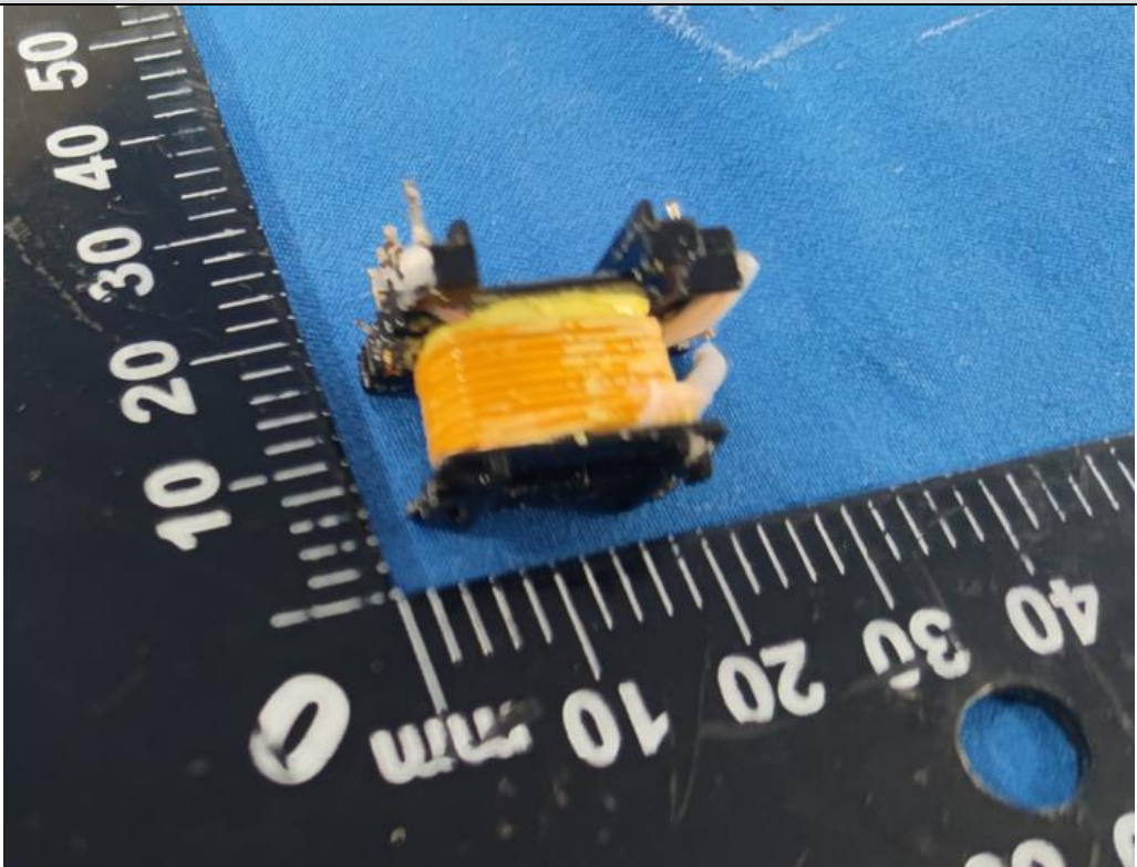
变压器内部结构 (次级绕组)
