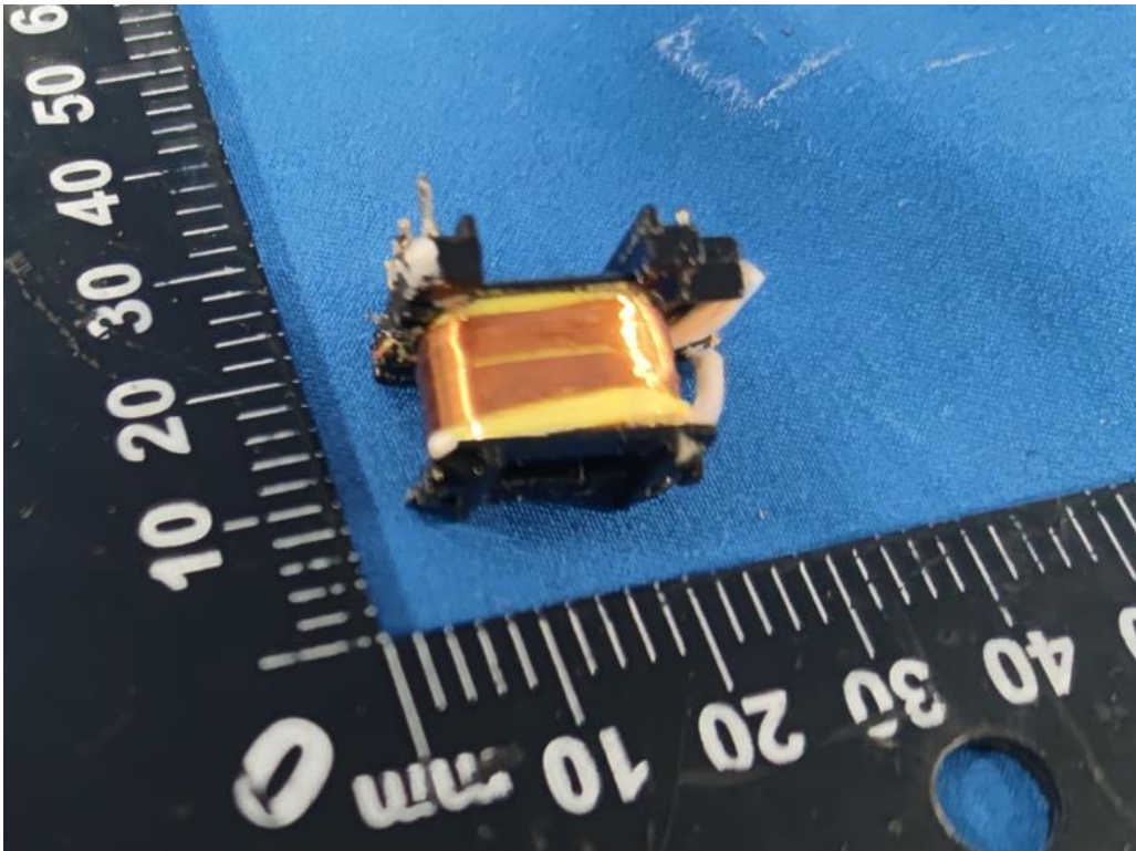
变压器内部结构 (初级绕组)
