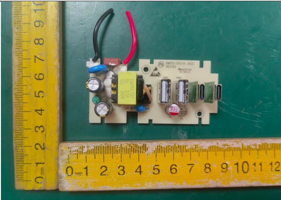
USB1模块正面（结构二） 本次增加
