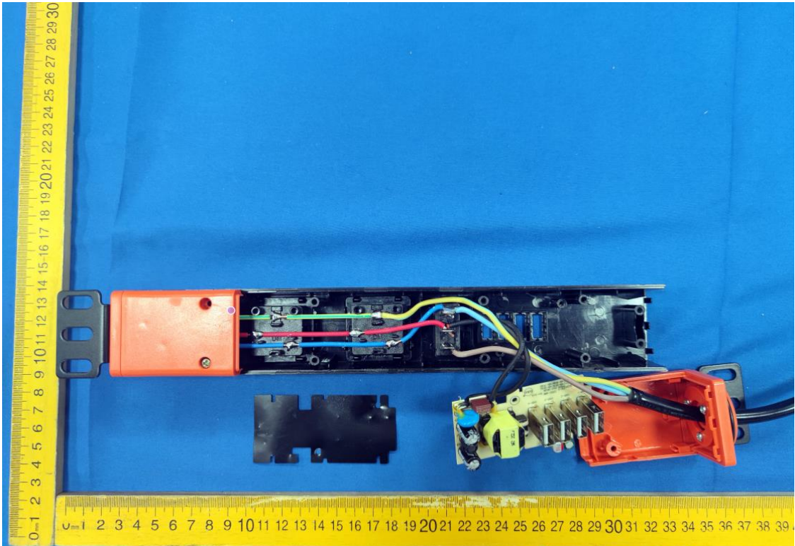
内部结构
