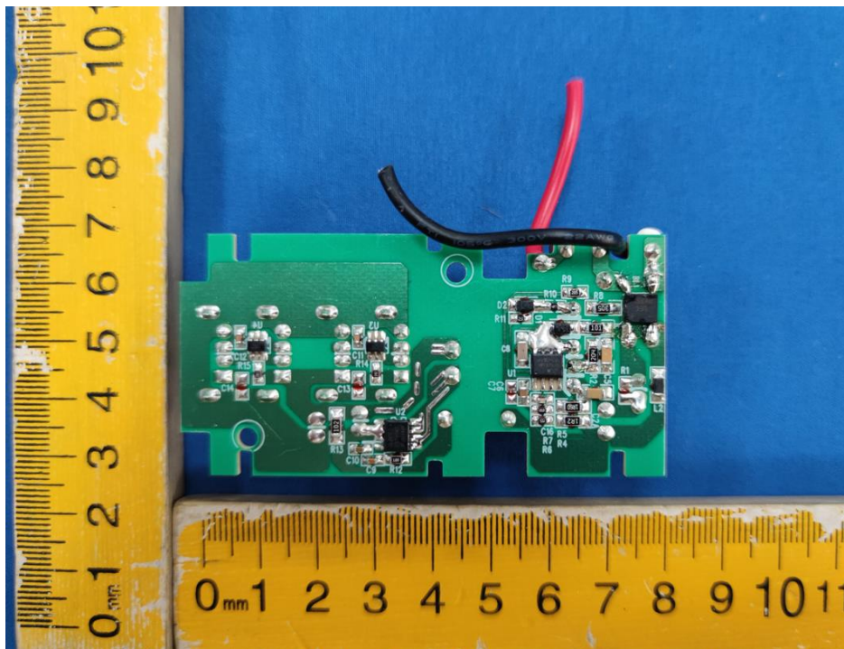
USB1模块背面 (结构一)
