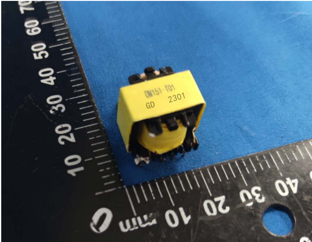
变压器外观
