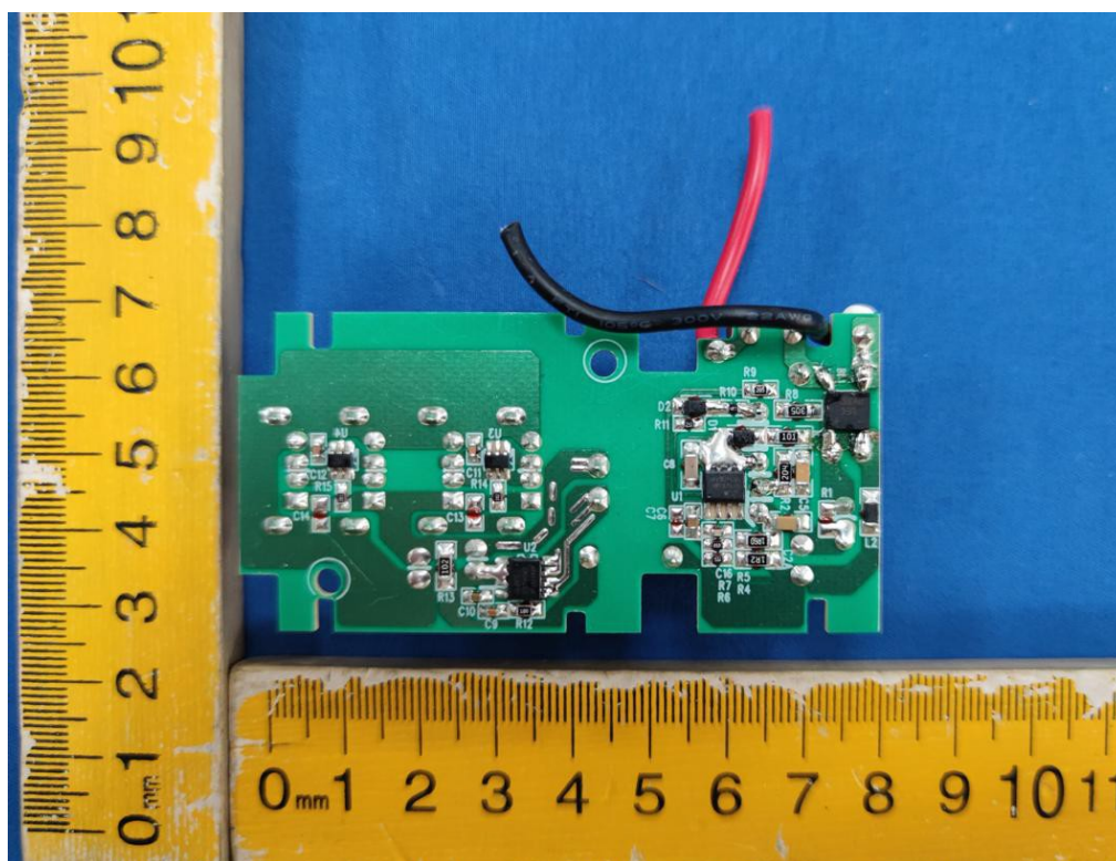
主板背面 (型号: DM151)
