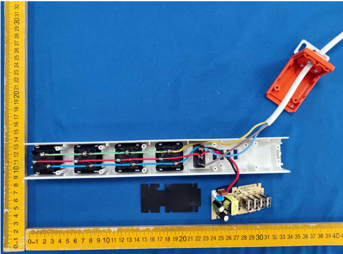
内部结构
