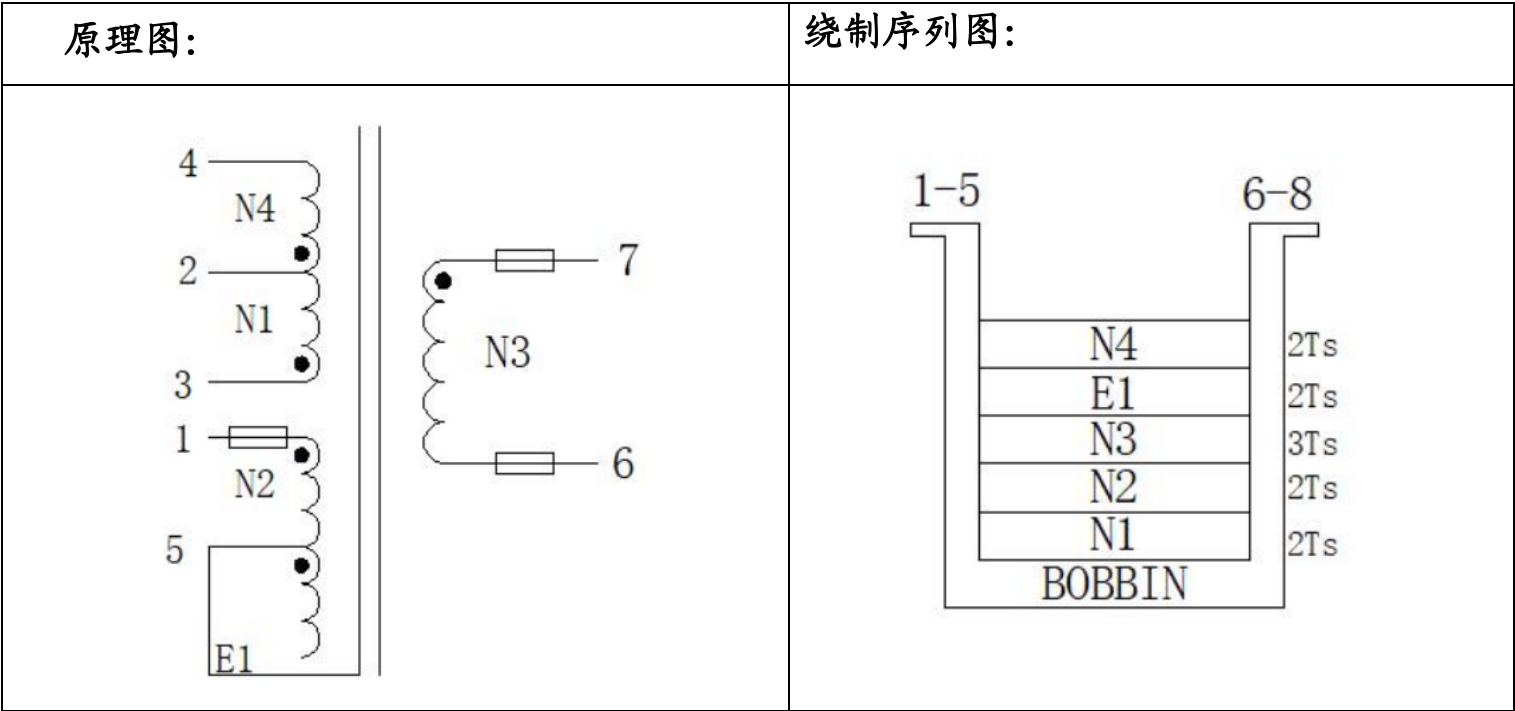
变压器原理图和结构图:
