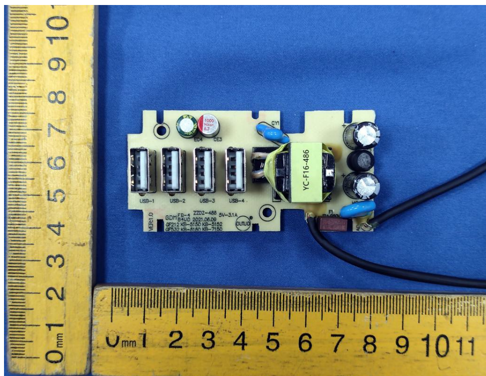
主板正面 (型号: ZDZ-486)
