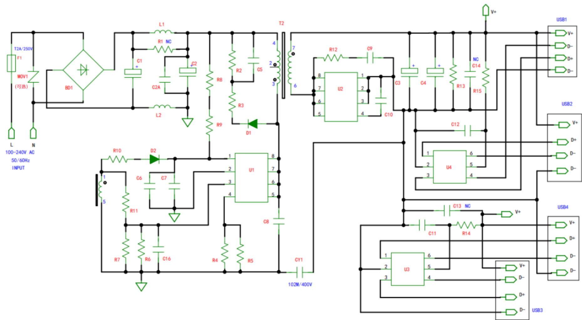
产品电气原理图:
