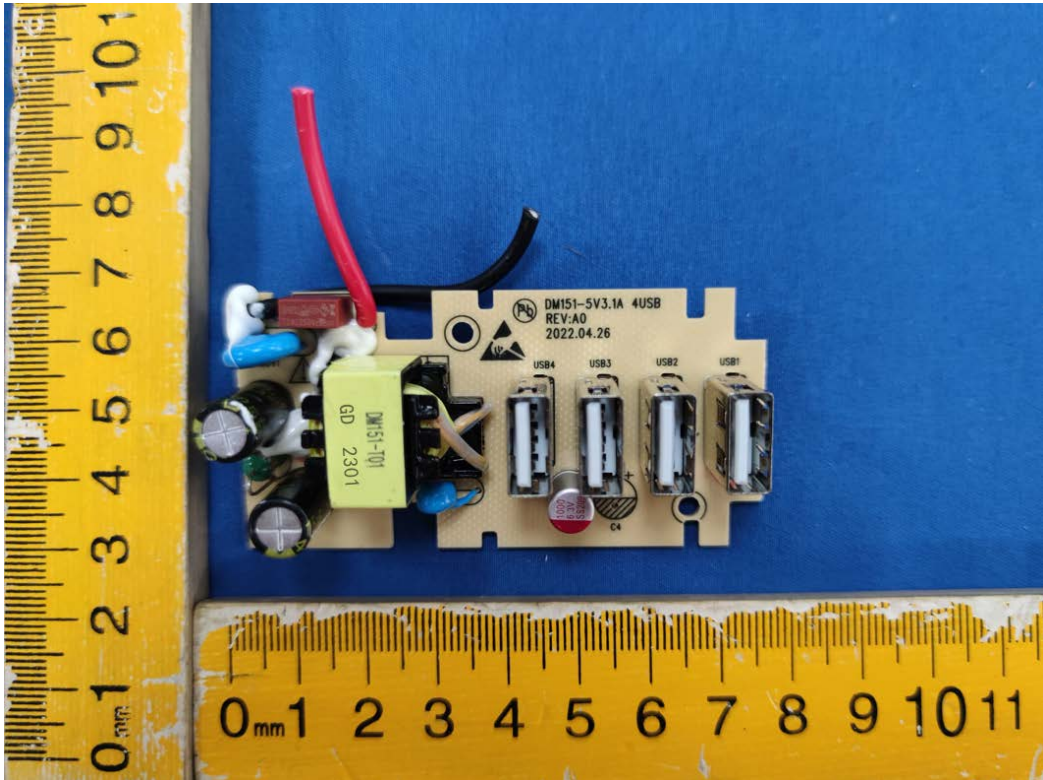
USB模块正面
