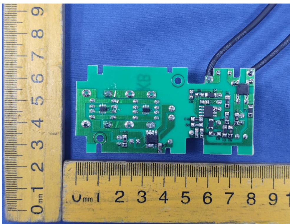
主板背面 (型号: ZDZ-486)
