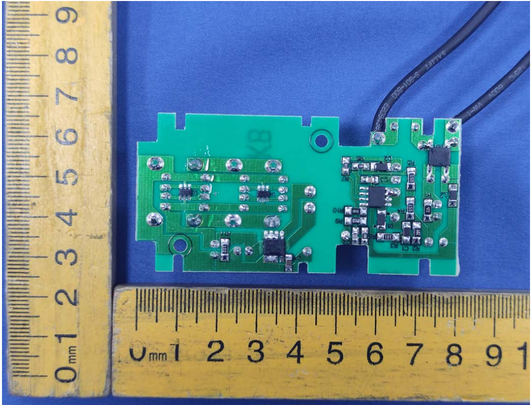
USB模块背面
