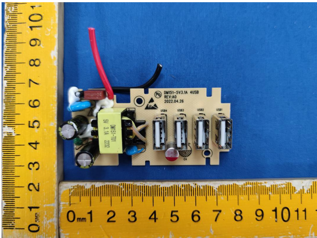
主板正面 (型号: DM151)
