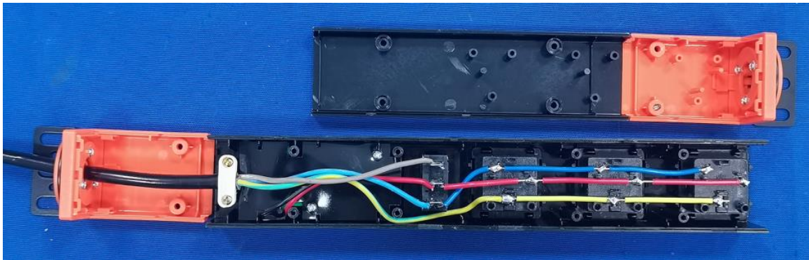
DM-10-XG3-KU2C2（黑） 内部结构
