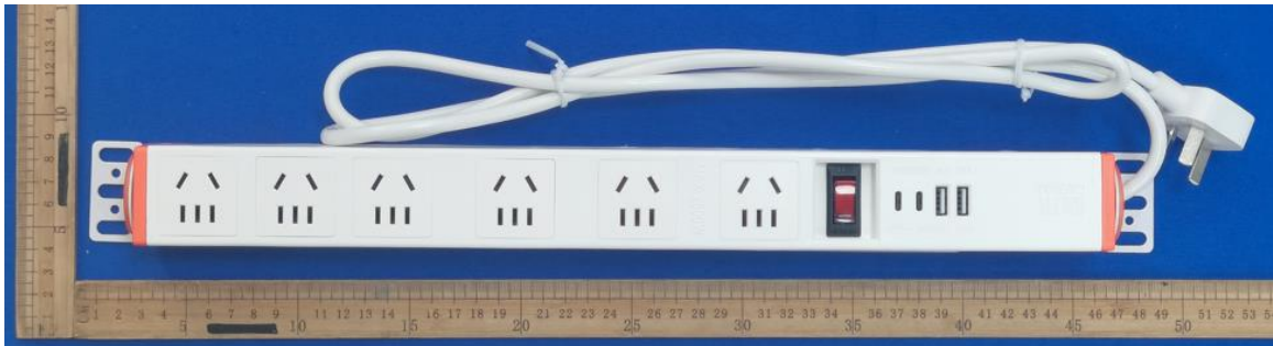
DM-10-XG6-KU2C2（白） 外观
