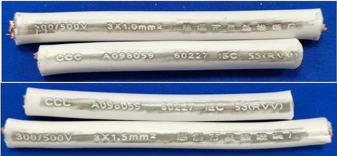
DM-10-XG6-KU2C2（白） 配线
