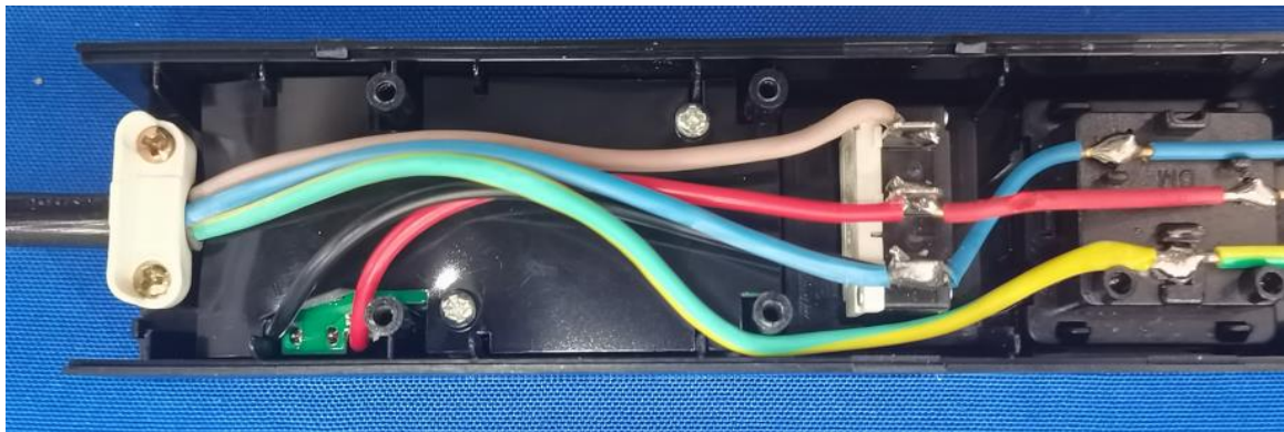
DM-10-XG6-KU2C2 (黑) 内部结构
