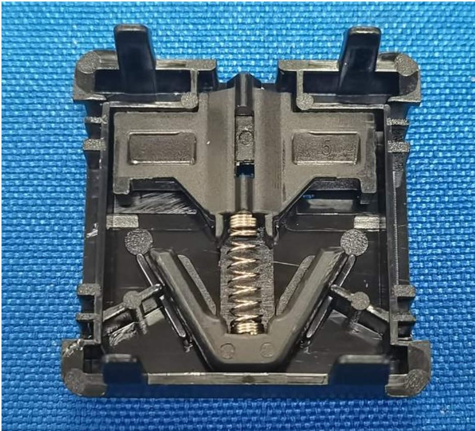
DM-10-XG6-KU2C2（黑） 内部结构
