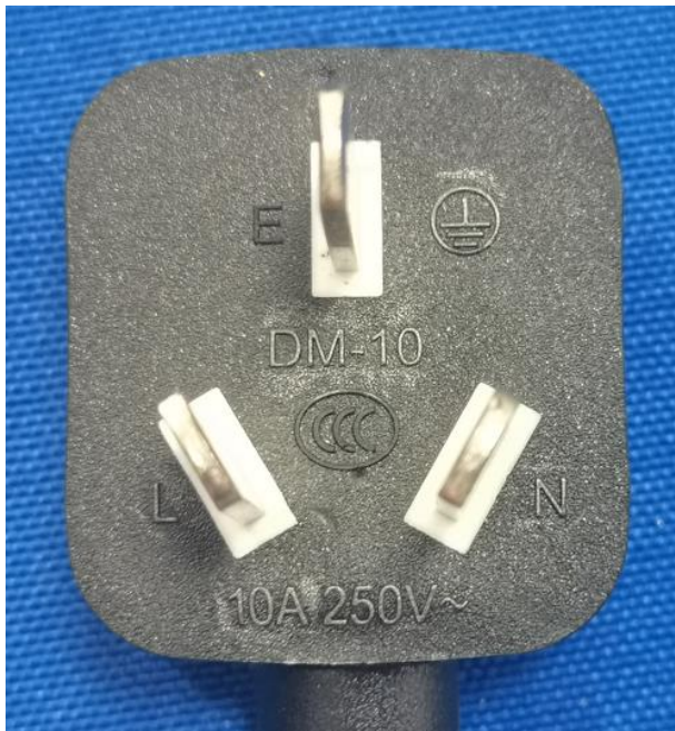
DM-10-XG6-KU2C2 (黑) 插头
