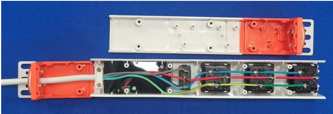
DM-10-XG3-KU2C2（白） 内部结构
