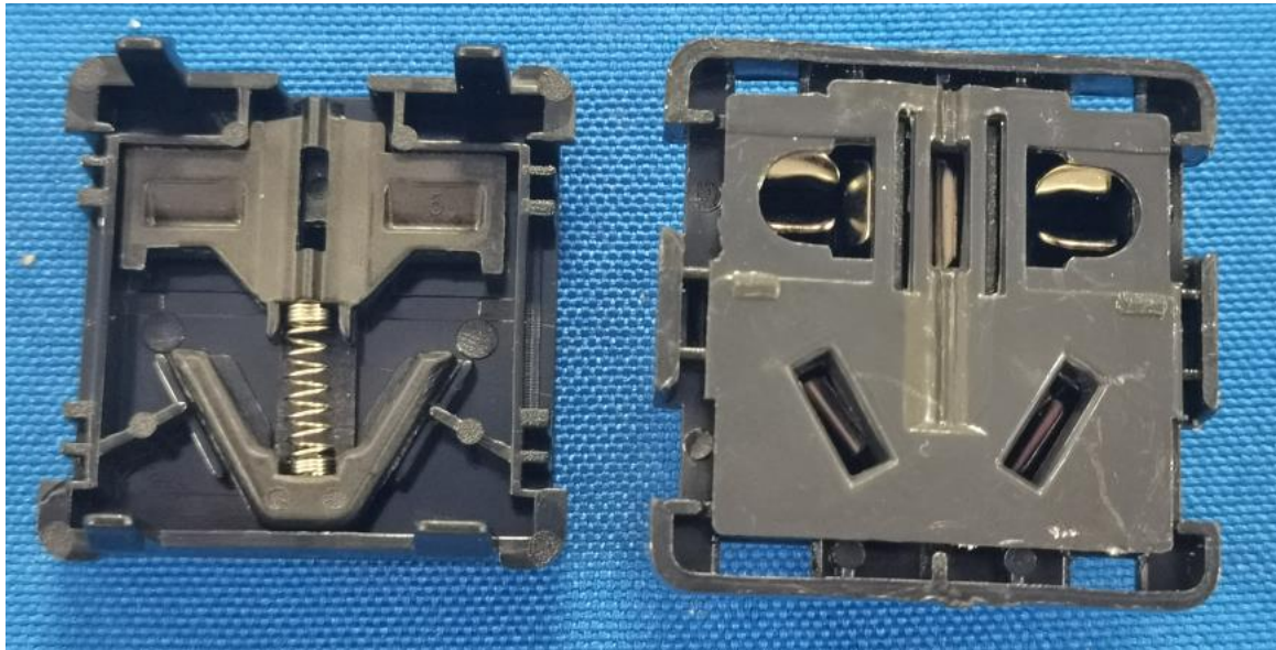
DM-10-XG6-KU2C2 (黑) 内部结构
