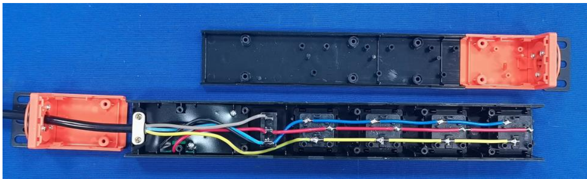
DM-10-XG4-KU2C2（黑） 内部结构
