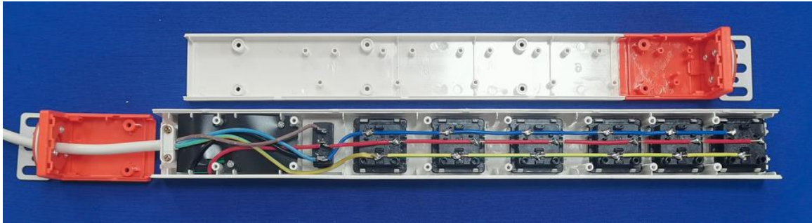
DM-10-XG6-KU2C2（白） 内部结构
