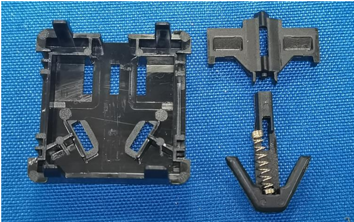
DM-10-XG6-KU2C2（黑） 内部结构
