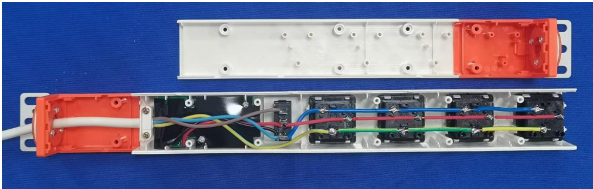
DM-10-XG4-KU2C2（白） 内部结构
