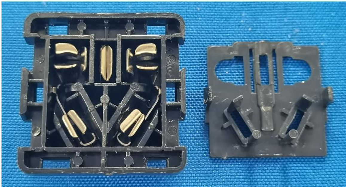
DM-10-XG6-KU2C2 (黑) 内部结构
