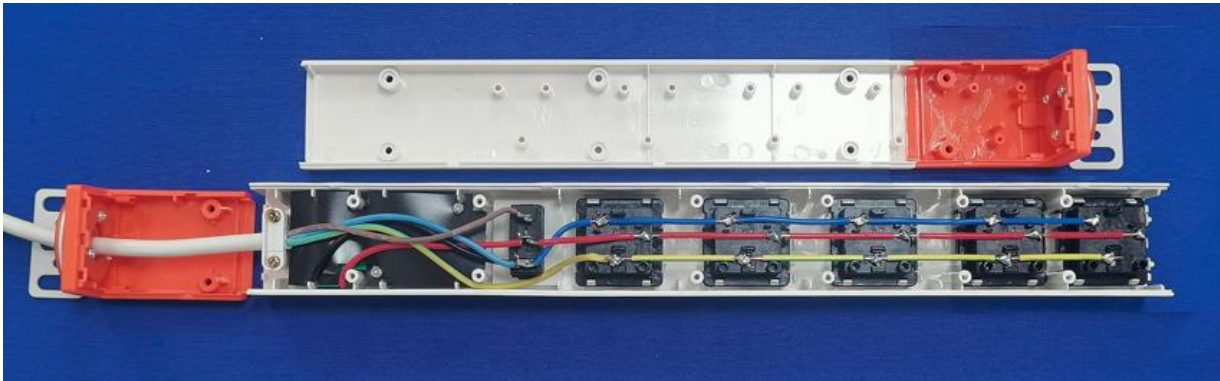
DM-10-XG5-KU2C2（白） 内部结构
