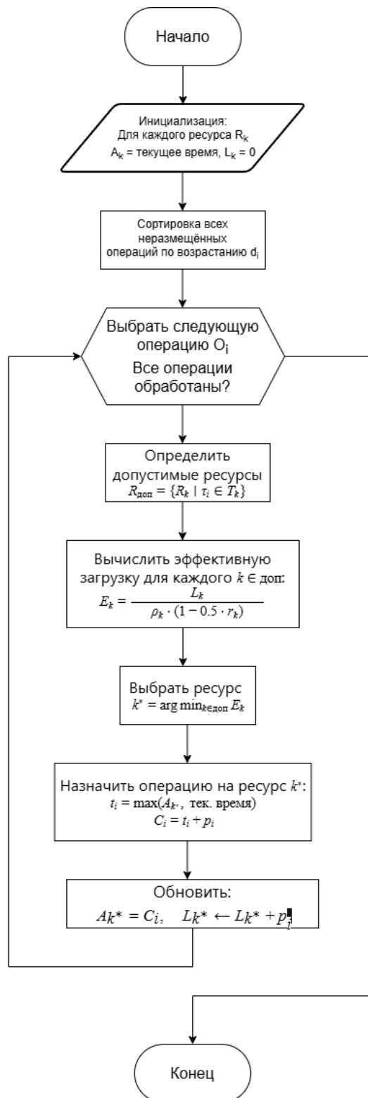
Рисунок 2.1 – Блок-схема эвристического алгоритма EDD+LWKR
