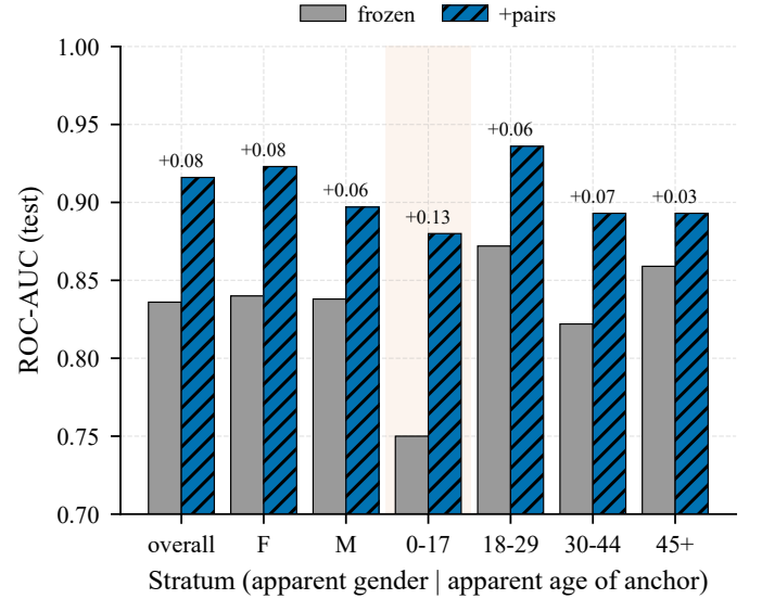
Рис. 5. Аудит по кажущимся стратам: frozen против +pairs ROC-AUC по стратам кажущихся пола/возраста. Все страты улучшаются; максимальный прирост — у младшей группы (0–17), где frozen слабее всего.
