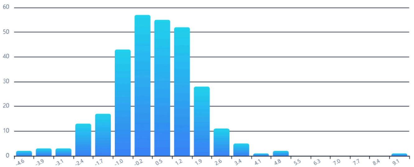
殘差分佈
