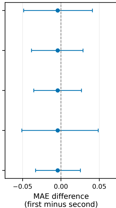
KcatNet - PMAK
