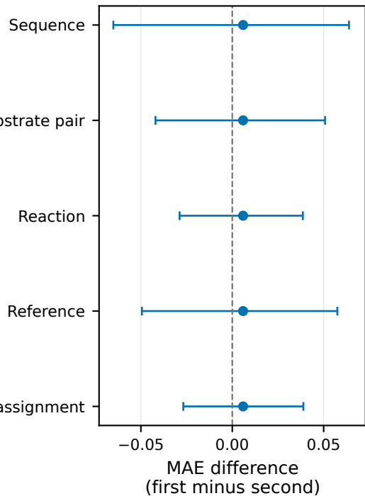
KcatNet - TurNuP
