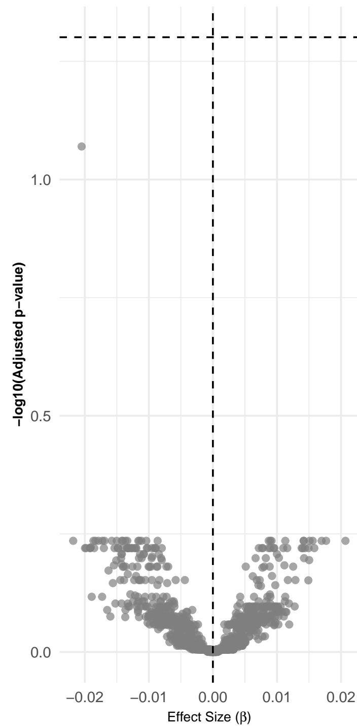
ECAS_SCORE (BEADdel)
