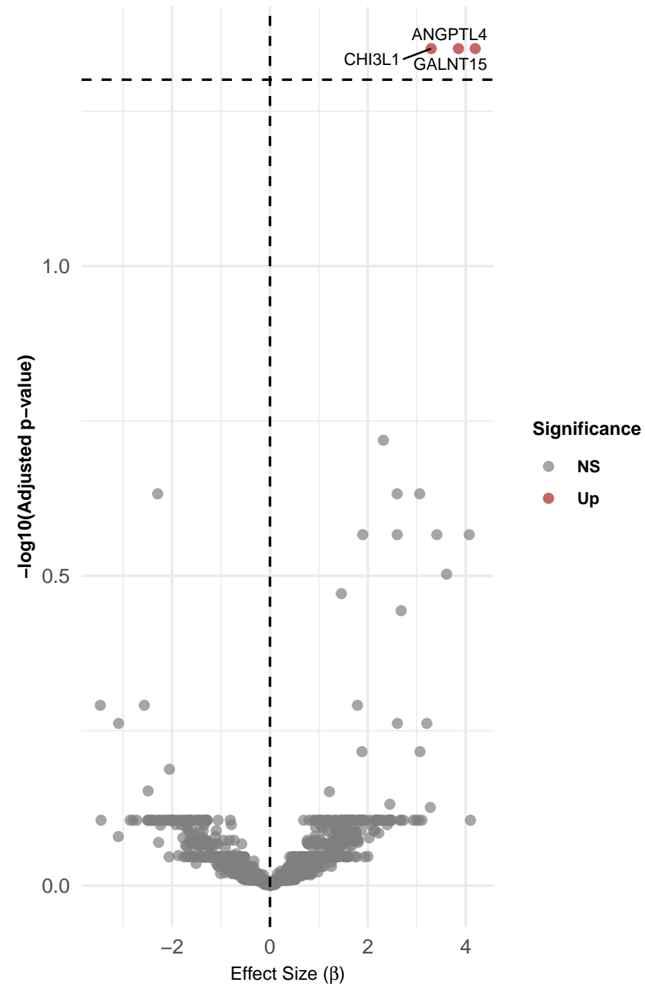
ALSvsHC (BEADdel)
