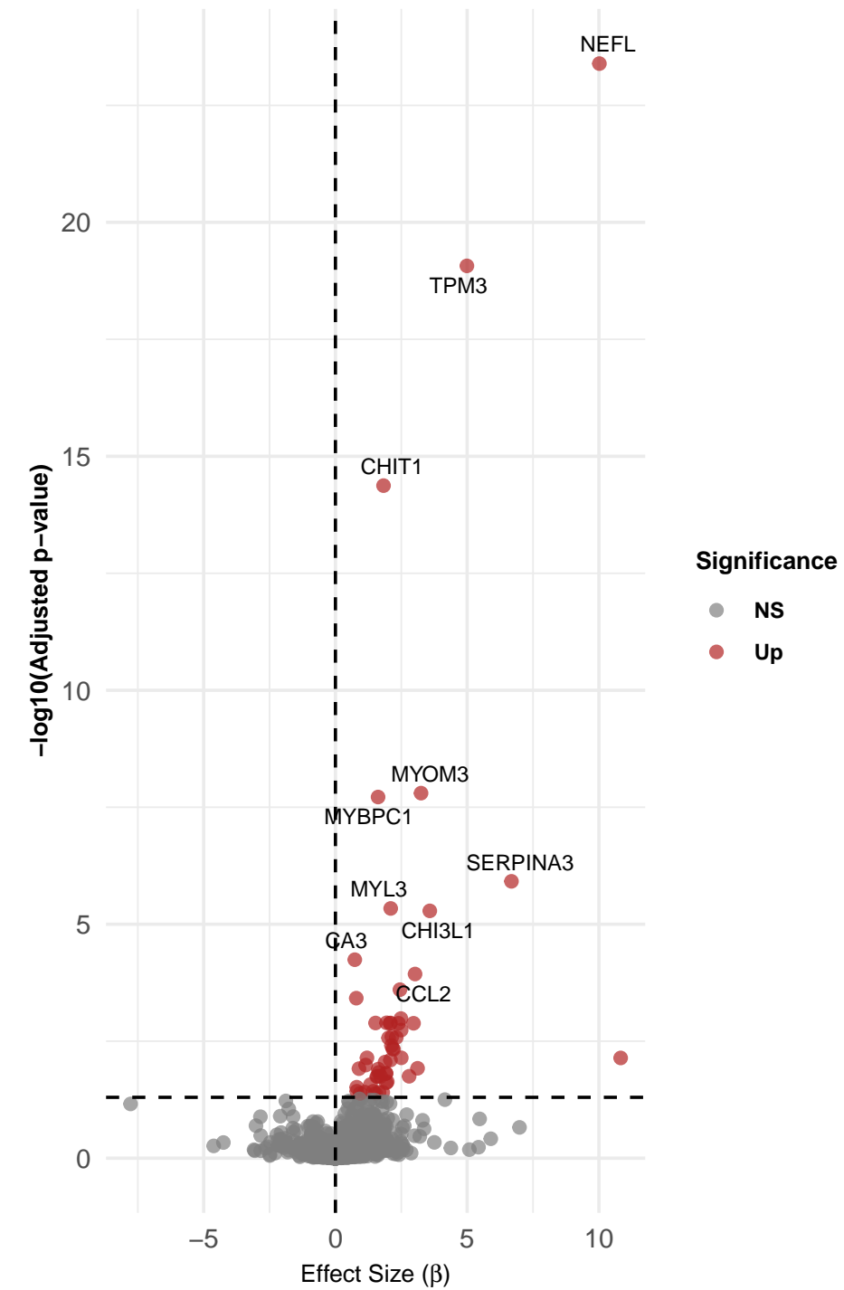
ALSvsHC (Olink)
