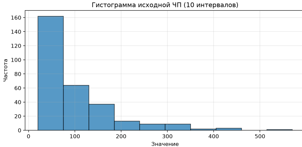
Рис. 3. Гистограмма распределения частот исходной последовательности
