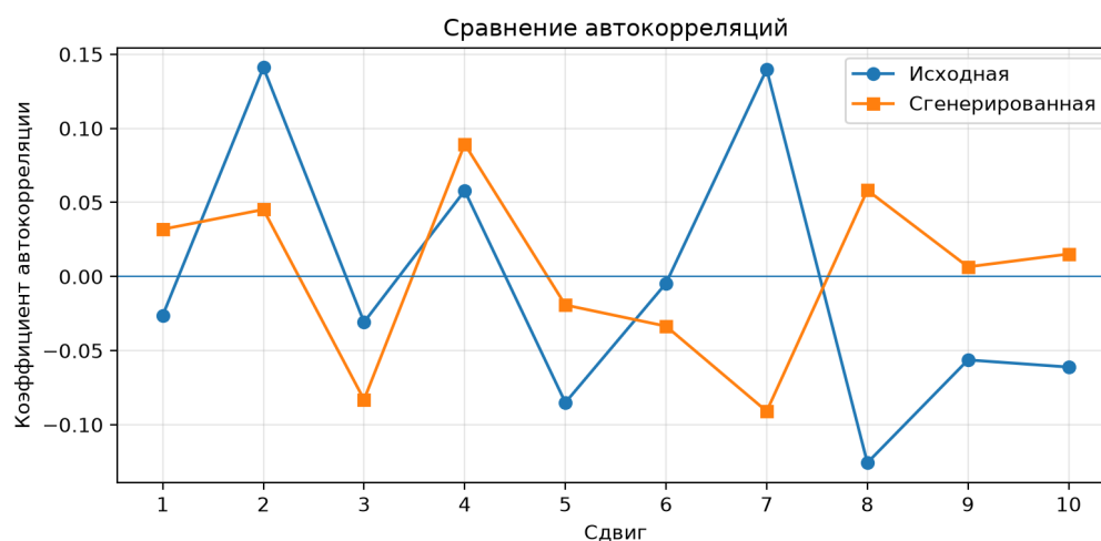
Рис. 7. Сравнение коэффициентов автокорреляции
