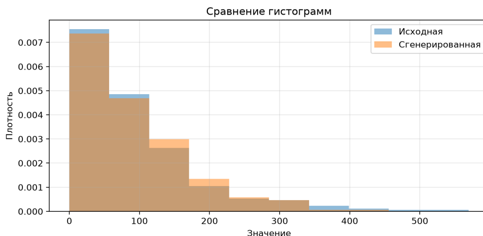
Рис. 6. Сравнение гистограмм исходной и сгенерированной последовательностей
