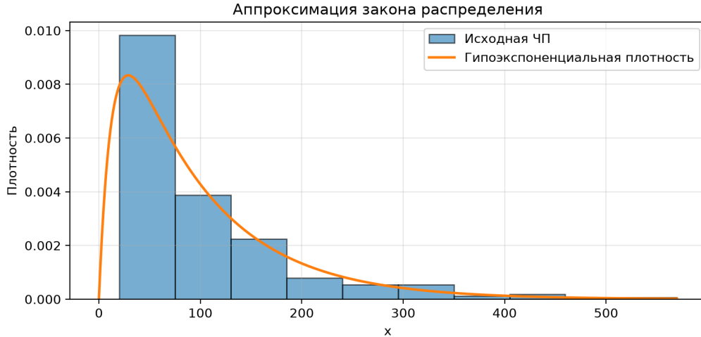
Рис. 4. Сравнение гистограммы исходной ЧП и плотности аппроксимирующего закона
