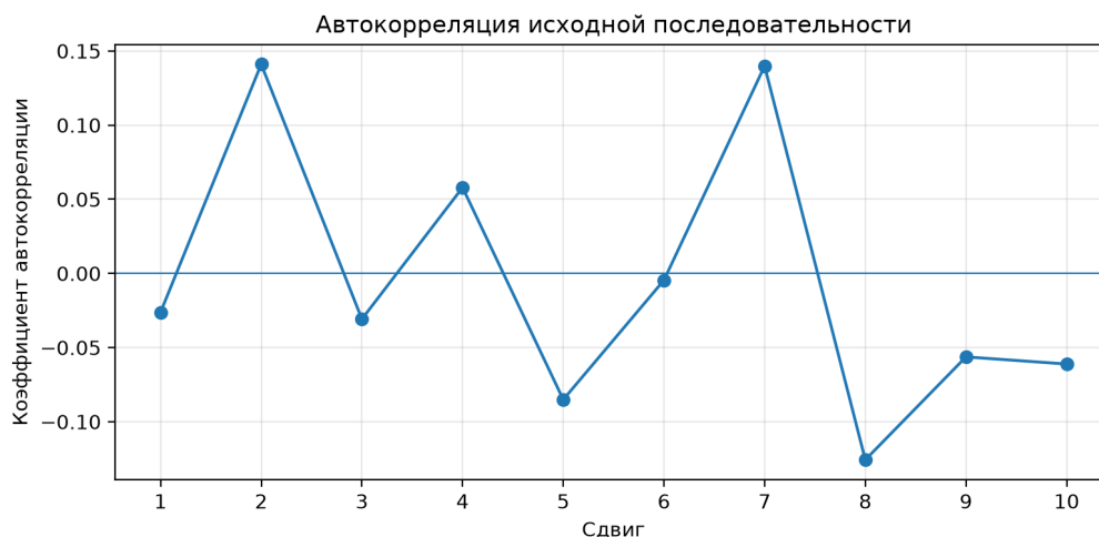
Рис. 2. Автокорреляция исходной последовательности
