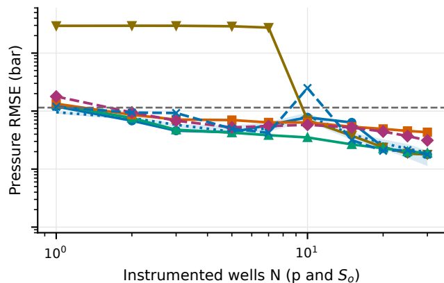
(d) P1, existing wells
