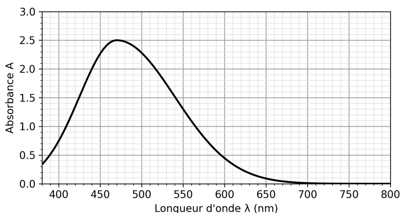
Fig. 2. – Spectre d'absorption du diiode
