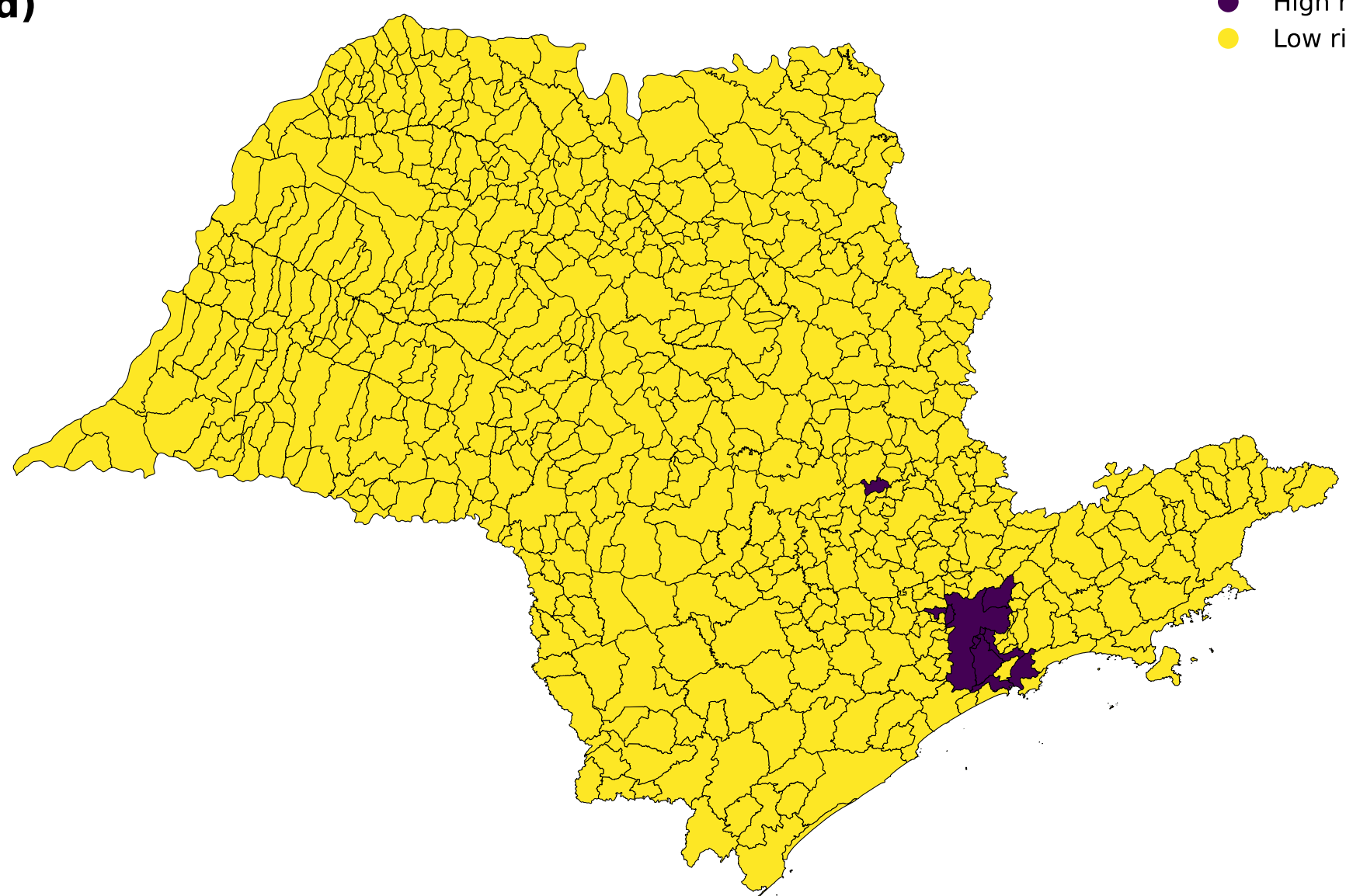
AdaBoost
