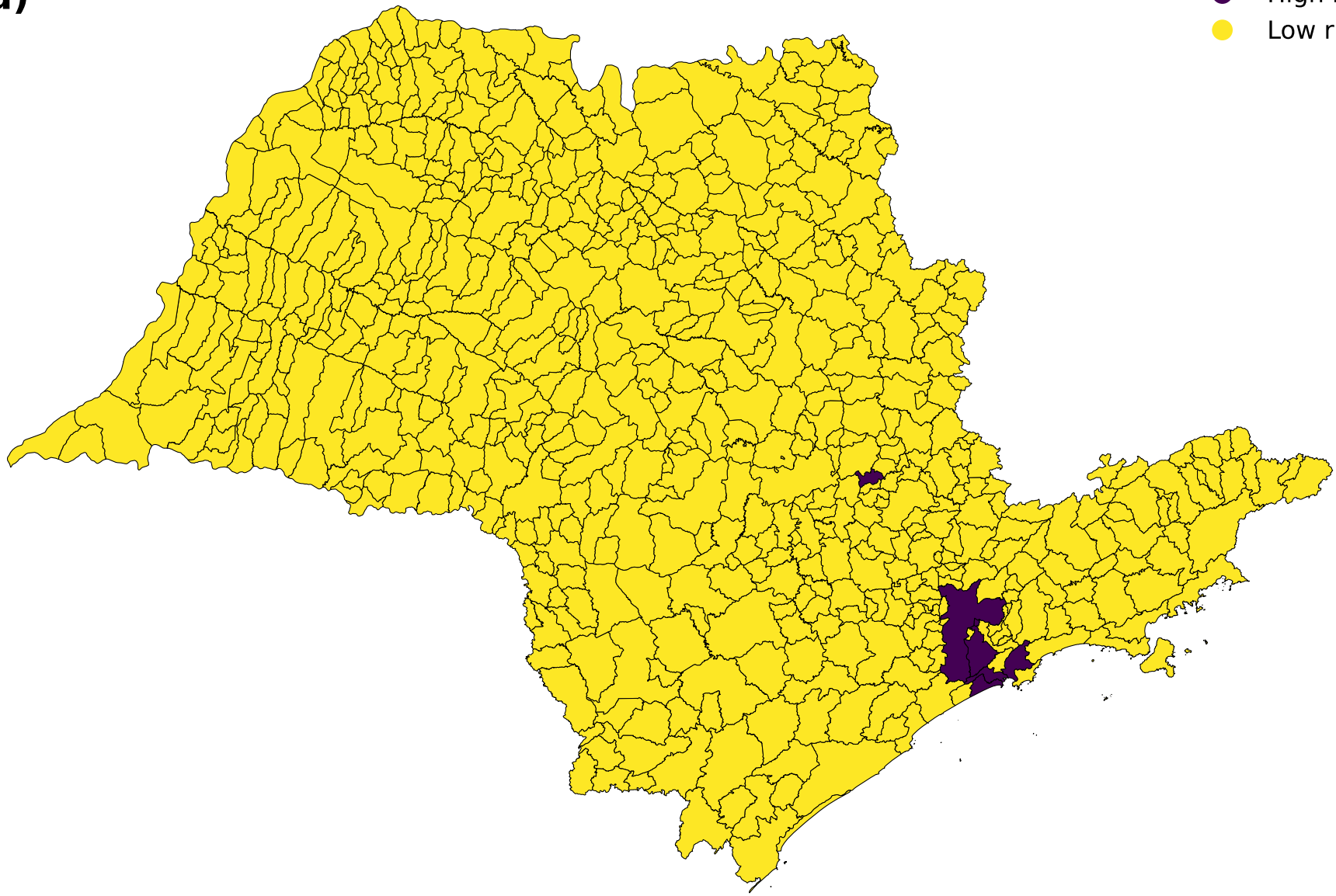
CatBoost
