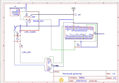
Схема установки
