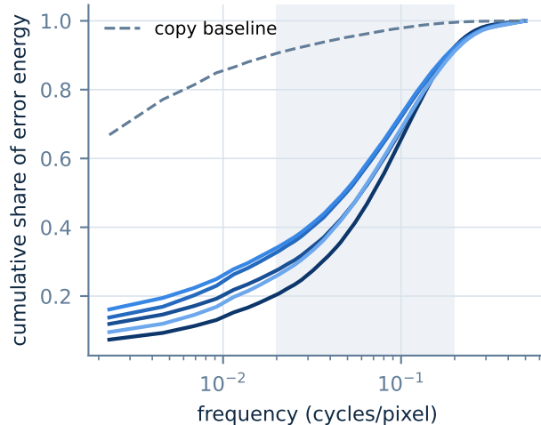
b · cumulative error
