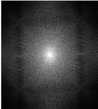
k-space
