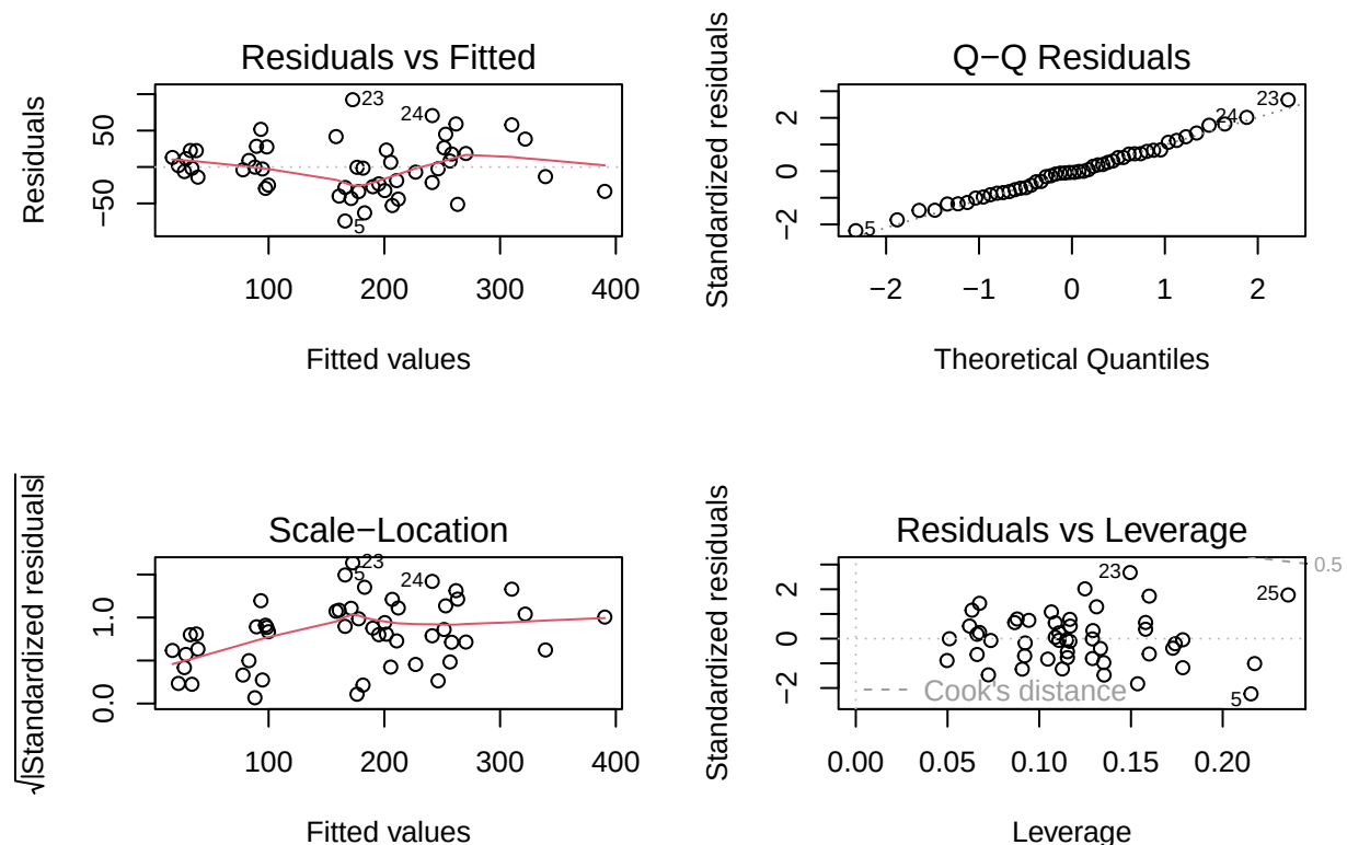
Hình 15: Các đồ thị phân tích thẳng dư đánh giá điều kiện của mô hình hồi quy
