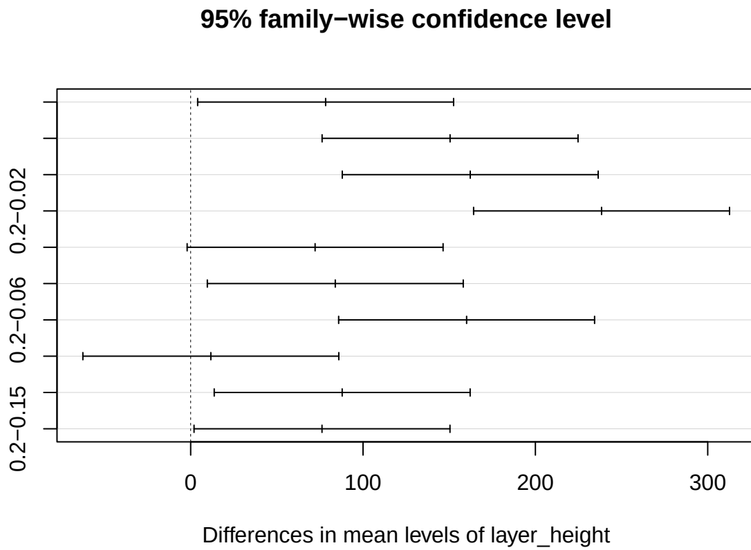
Hình 13: Đồ thị kiểm định hậu kiểm Tukey (Tukey HSD) cho các mức chiều cao lớp in
