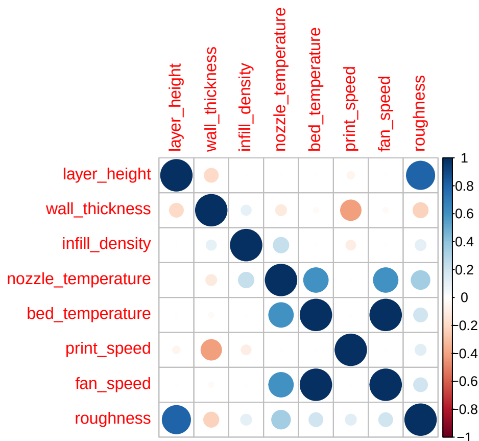
Hình 14: Biểu đồ ma trận tương quan giữa các biến điều chỉnh định lượng
