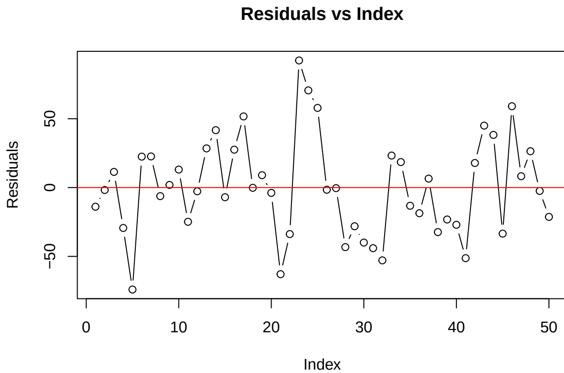
Hình 16: Biểu đồ kiểm tra tính độc lập của các sai số (Residuals vs Index)
