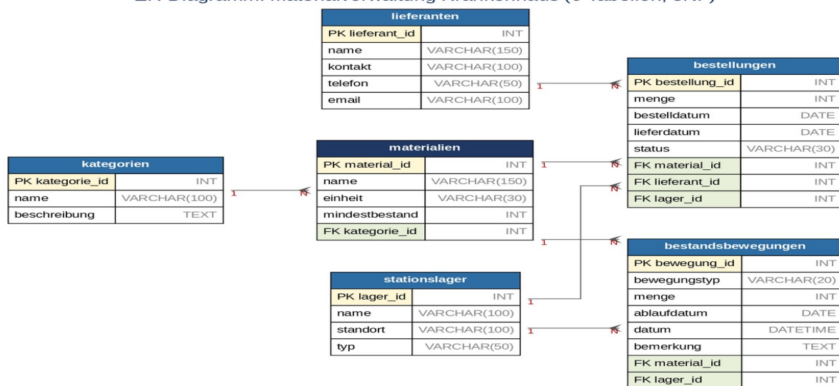
ER-Diagramm: Materialverwaltung Krankenhaus (6 Tabellen, 3NF)
