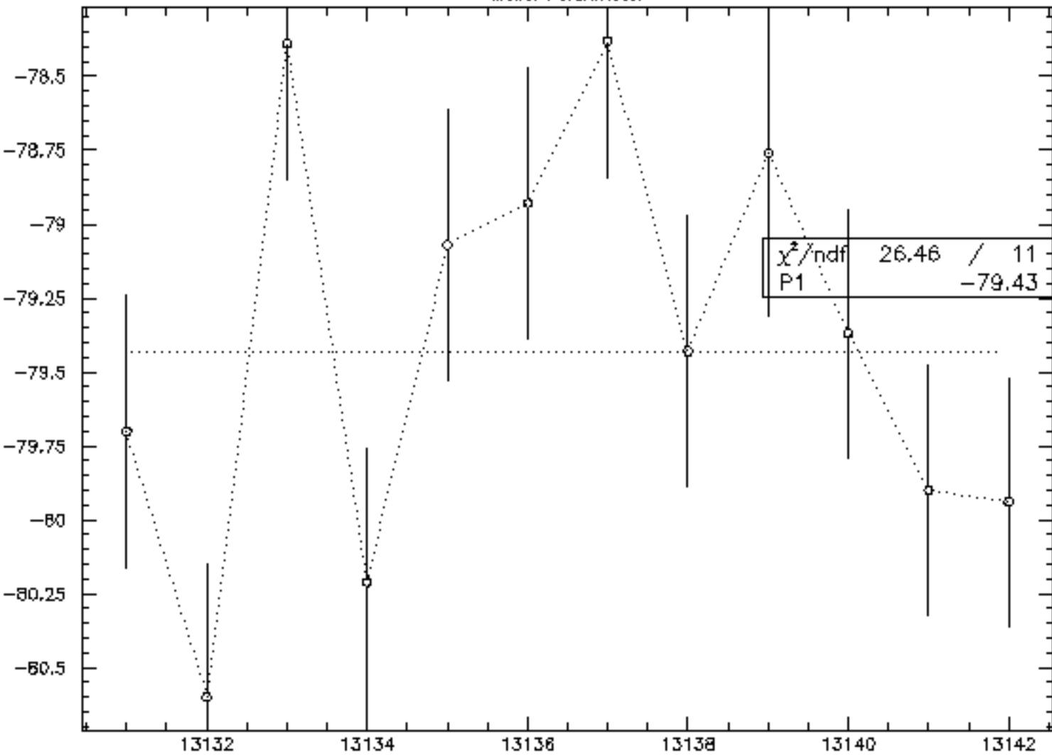
Moller Polarimeter
