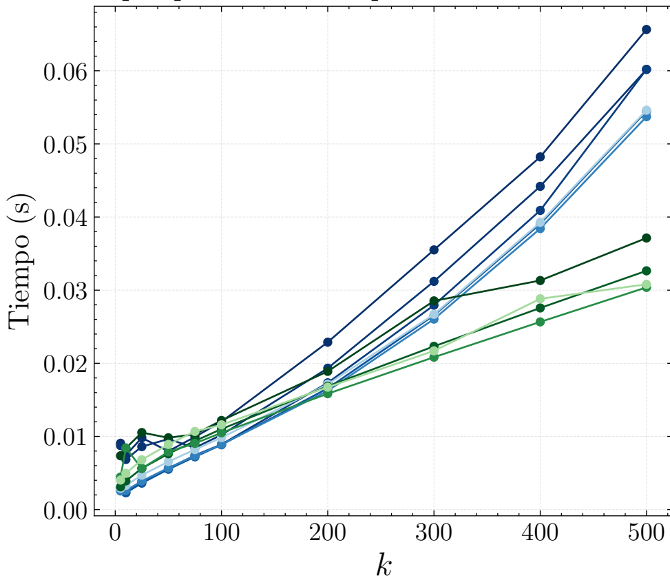
Tiempos para 10000 búsquedas KNN en 5080_54400
