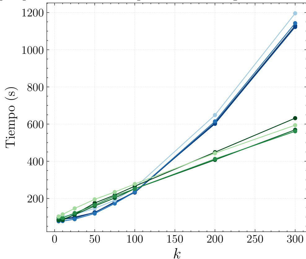
Tiempos para 429615314 búsquedas KNN en sg27_station8 (full searches)
