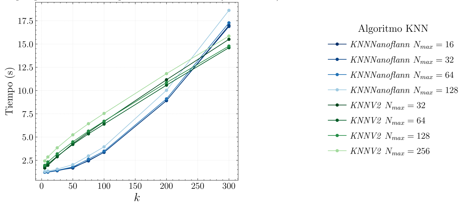
Tiempos para 100000000 búsquedas KNN en Lille_0 (full searches)
