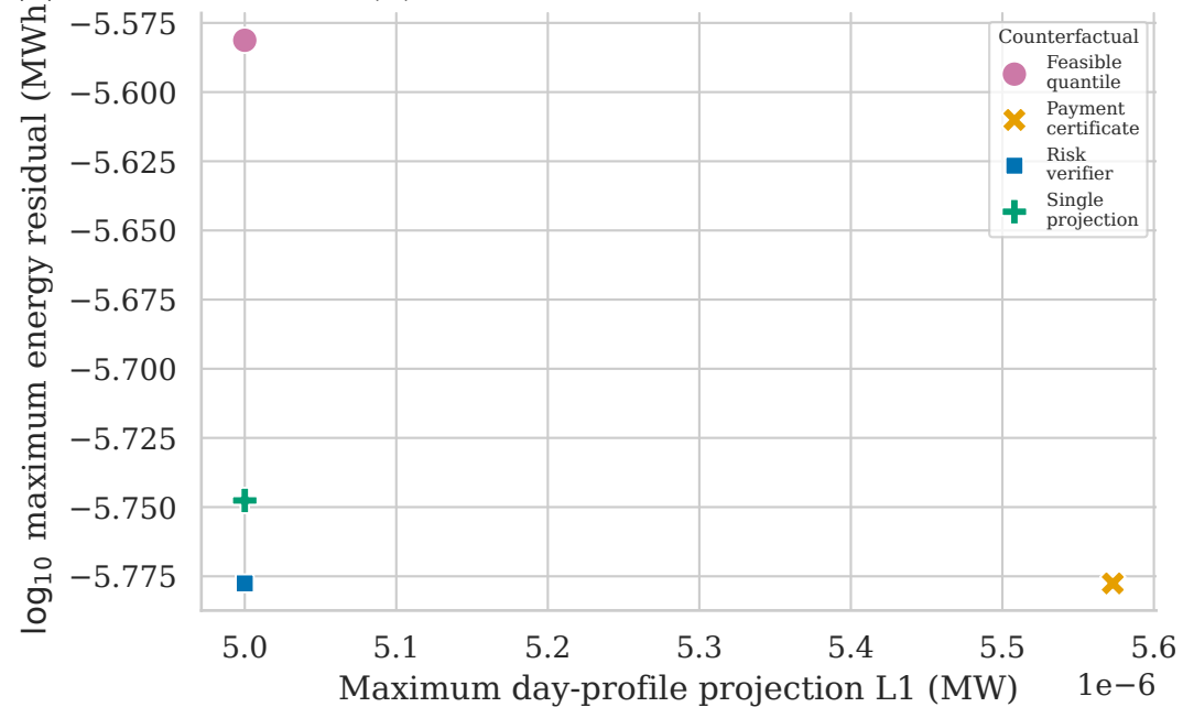
(d) Continuous-horizon certificates
