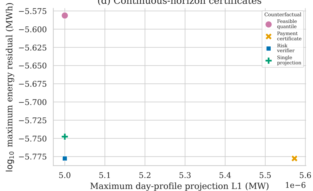
(d) Continuous-horizon certificates
