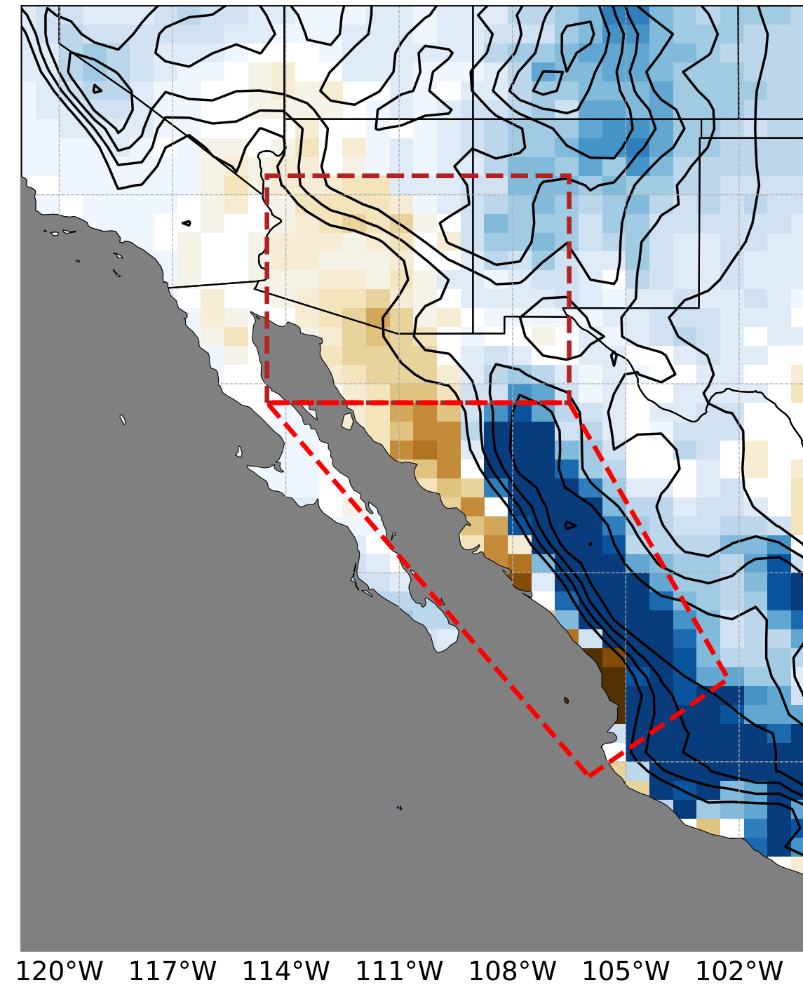
D CTRL-GPCC
