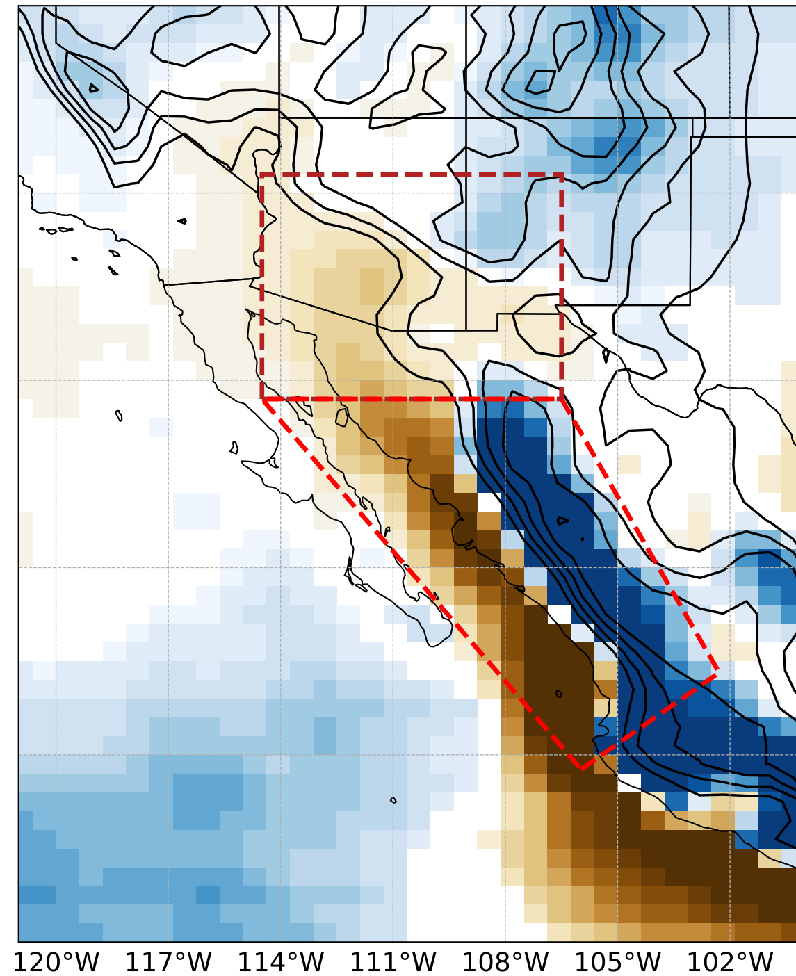
C CTRL-GPCP
