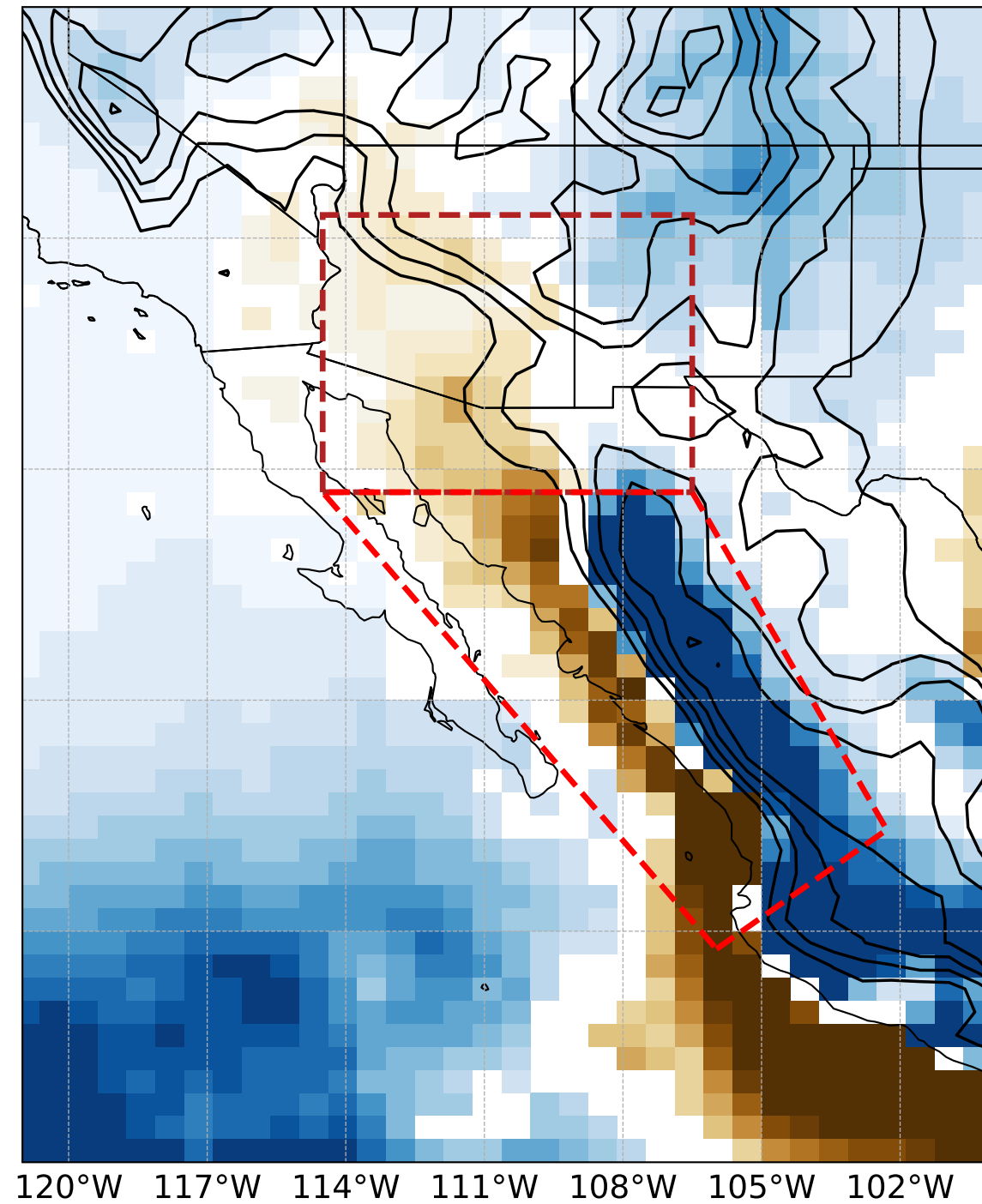
B CTRL-TRMM
