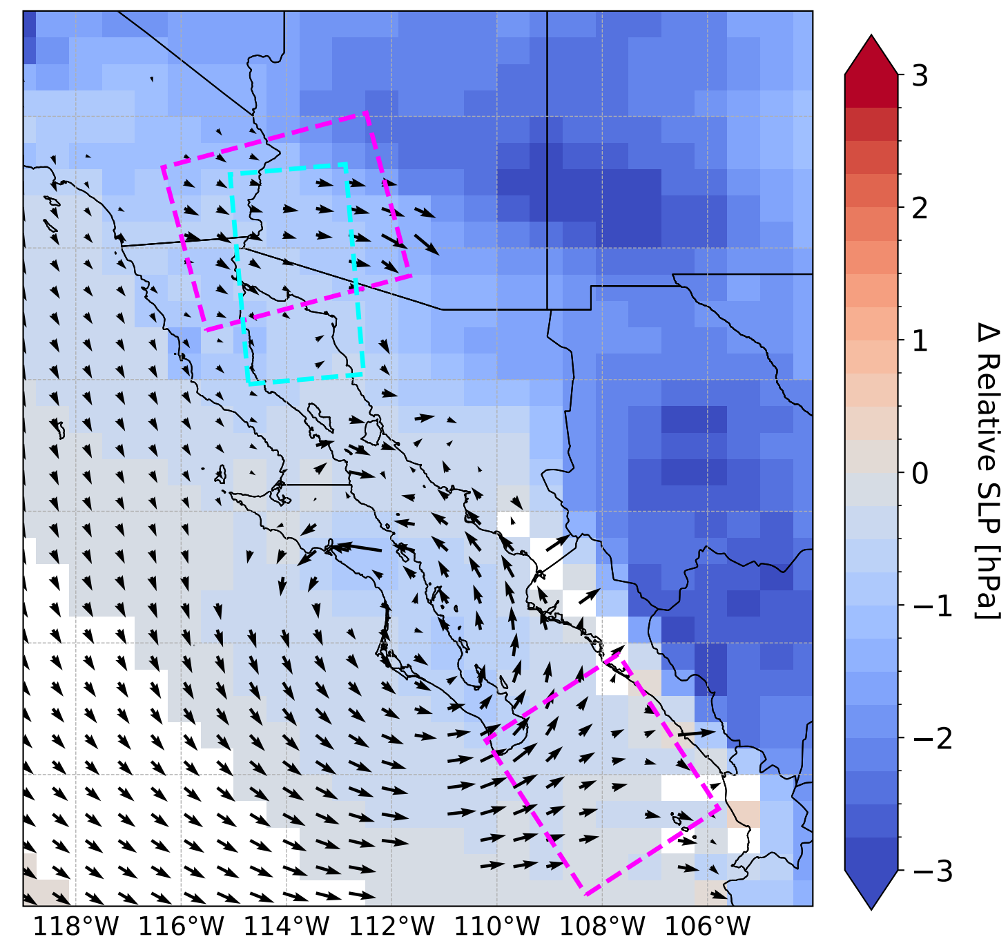
C HI MEX -CTRL
