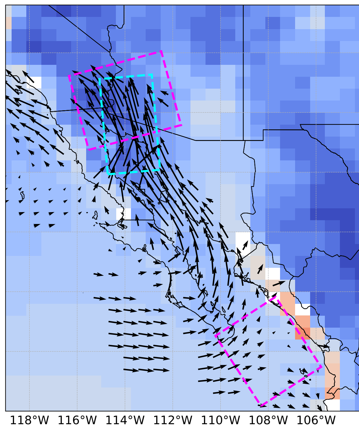
B HI GBL -CTRL
