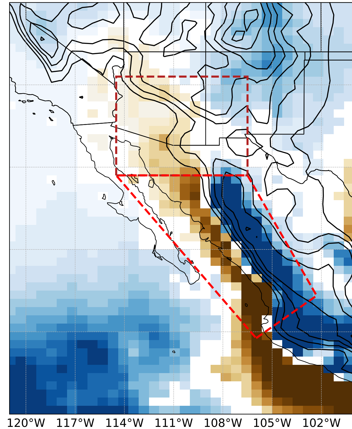
B CTRL-TRMM
