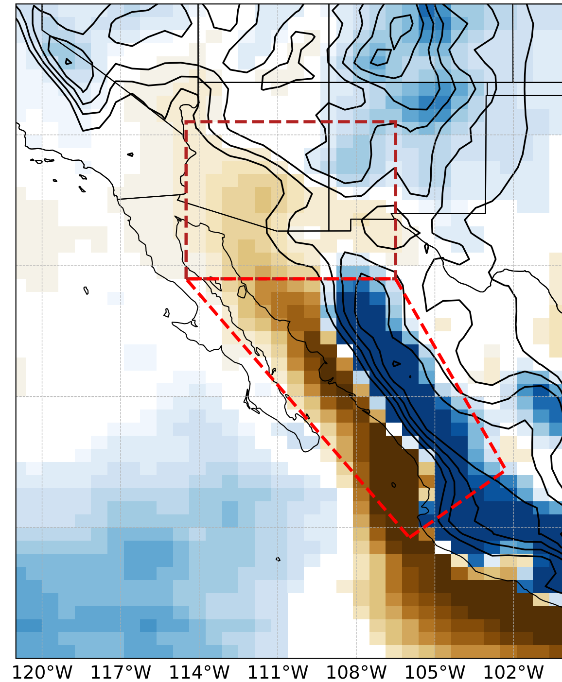
C CTRL-GPCP
