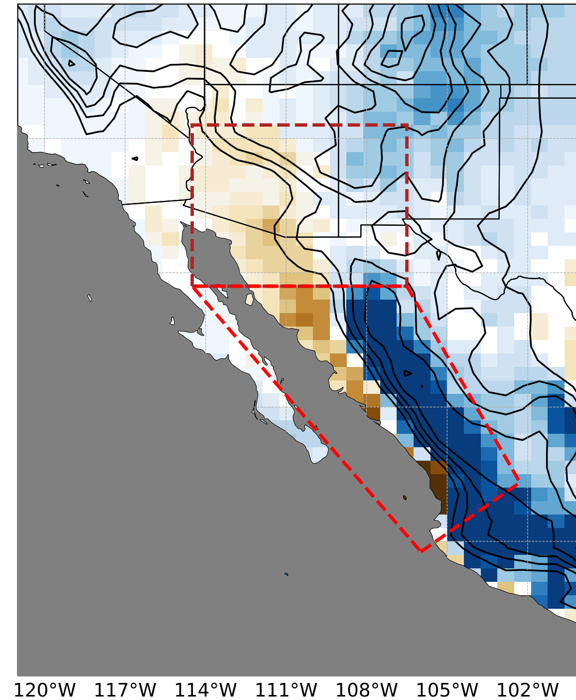
D CTRL-GPCC
