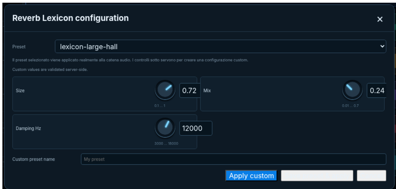
Figura 6 - Schermata reale del configuratore plugin: il preset aggiorna immediatamente i parametri e ogni controllo continuo offre knob e valore numerico sincronizzati.
