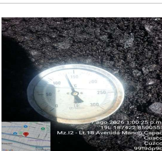
Verificación de la temperatura de la mezcla asfáltica T°: 140°C Verificación de la imprimación
