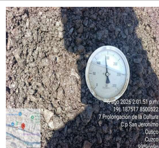
Verificación de la imprimación Verificación de la temperatura de la mezcla asfáltica T°: 140°C
