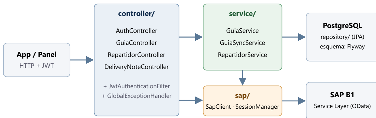
Figura 1 · Capas de la aplicación. El login y la inspección van directo del controller a sap/ ; la sincronización pasa por GuiaSyncService .
