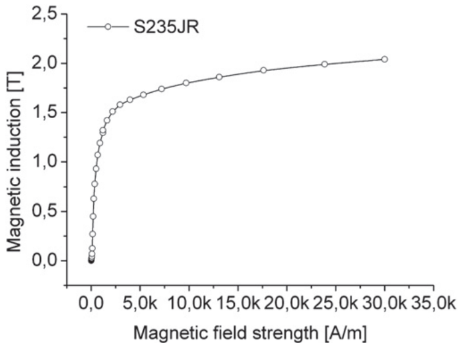
Figuur 5.15: BH -curve van S235JR. Het is belangrijk dat de curve bij onze waarde voor B_g lineair is, zodat er geen saturatie optreedt en er geen magnetisch veld weglekt. [BSE14]
