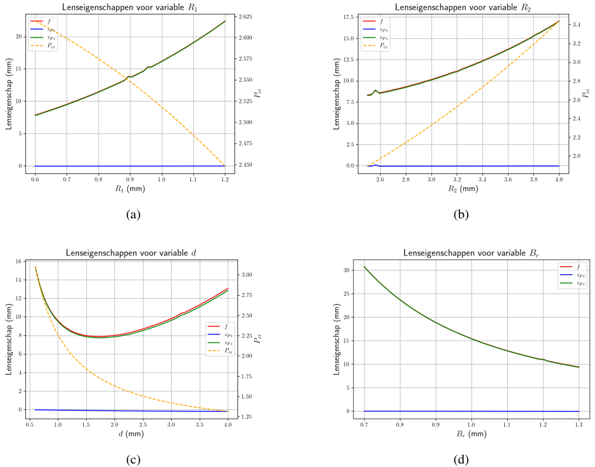
Figuur 5.17: Plots van lenseigenschappen en reluctantieterm in functie van de geometrie van de lens. Deze plots geven een goed beeld van hoe de parameters aangepast kunnen worden om de lenseigenschappen naar wens te optimaliseren. Naast de reluctantieterm moet er ook rekening gehouden worden met de maximale fluxdichtheid in de polepieces, welke niet te hoog mag zijn om saturatie-effecten te voorkomen.
