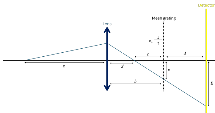
Figuur 4.7: Rear mesh shadowgraph methode voor een puntbron voor het focaalvlak van de lens. Door de magnificatie M = \frac{E}{e} te meten is het mogelijk om het beeldpunt z' en de focale lengte f te bepalen.
