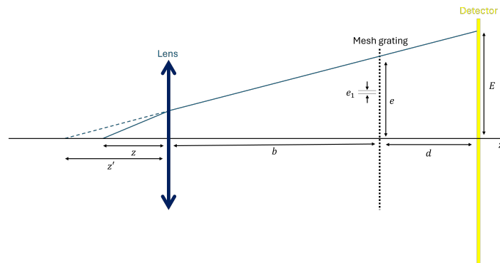
Figuur 4.8: Rear mesh shadowgraph methode voor een puntbron achter het focaalvlak van de lens. De elektronenbundel wordt nu niet gefocuseerd in een punt, maar de elektronenbundel is nog steeds divergerend wat een magnificatie M > 1 geeft.
