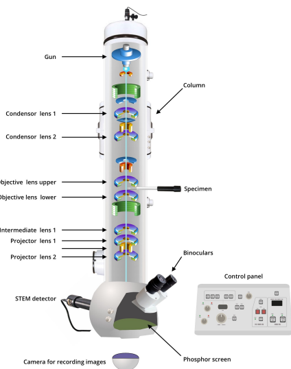
(a) Werkingsprincipe van een TEM waarbij een brede elektronenbundel heel het sample belicht en heel het beeld in 1 keer wordt opgenomen met een detector onder het sample. [19]
