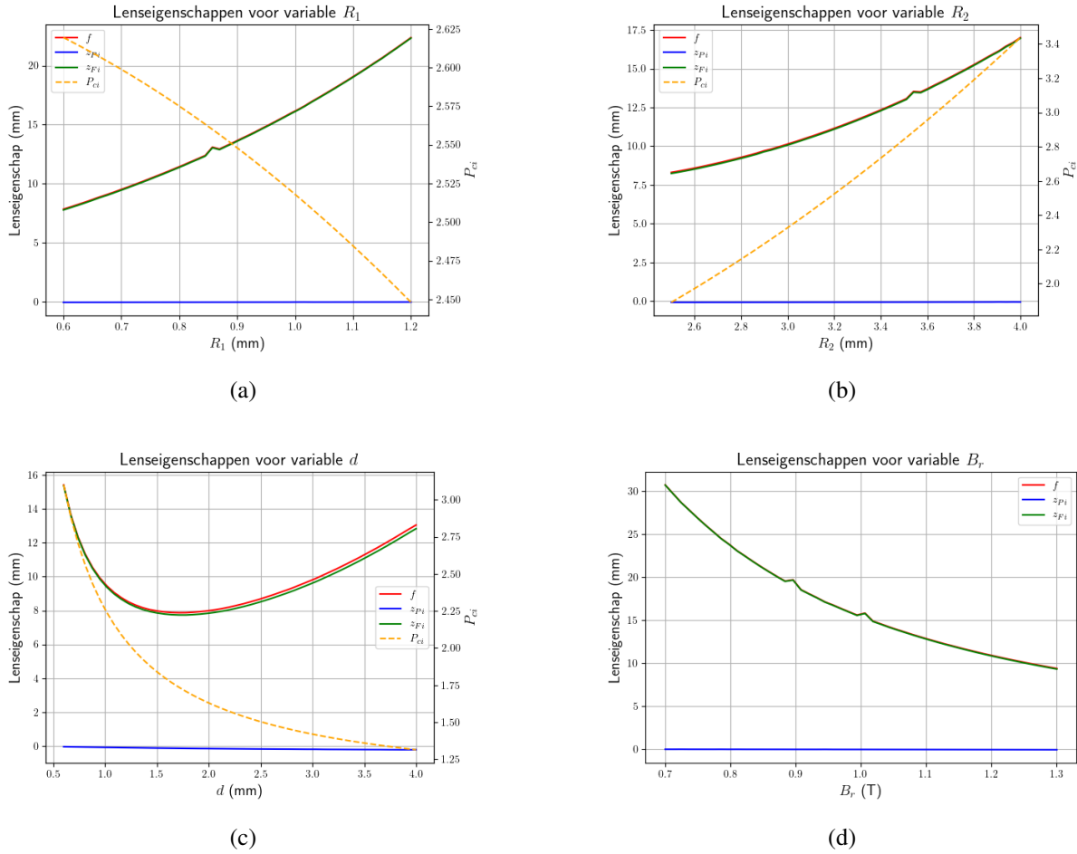
Figuur 4.3: Plots van lenseigenschappen en reluctantieterm in functie van de geometrie van de lens. Deze plots geven een goed beeld van hoe de parameters aangepast kunnen worden om de lenseigenschappen naar wens te optimaliseren. Naast de reluctantieterm moet er ook rekening gehouden worden met de maximale fluxdichtheid in de poolschoenen, welke niet te hoog mag zijn om saturatie-effecten te voorkomen.
