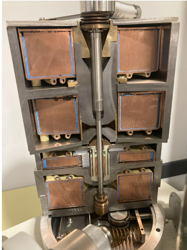
Figuur 1.1: Doorsnede van een Philips CM200 transmissie-elektronenmicroscop. In een typische elektronenlens maakt men gebruik van spoelen om een magnetisch veld op te wekken. [11]
