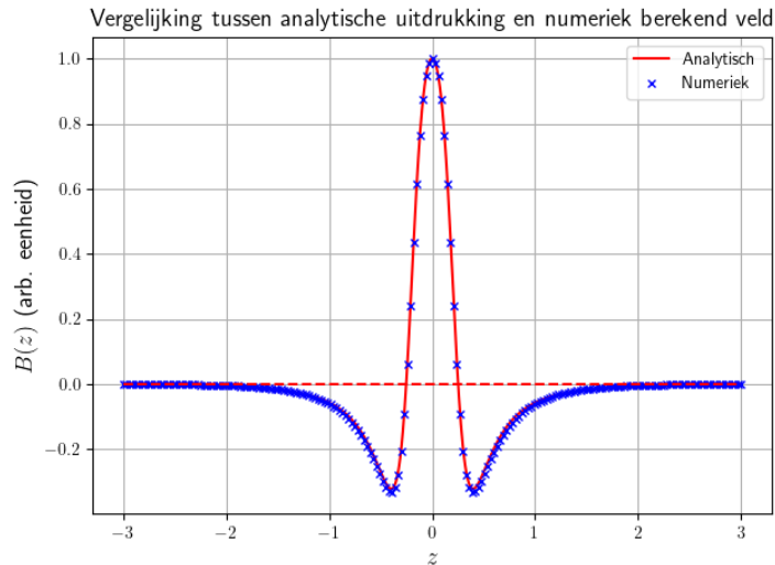
Figuur 3.7: Vergelijking tussen analytische uitdrukking en numeriek gesimuleerd veld voor R_1 = 2\text{mm} , R_2 = 3\text{mm} en d = 4\text{mm} . We zien dat de velden zeer goed overeenkomen.
