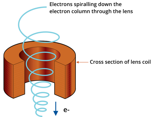
Figuur 2.3: Illustratie van een magnetische solenoïdelens. Dit soort lens maakt een magnetisch veld dat symmetrisch is rond de optische as van het systeem. Door een bundel elektronen door de lens te sturen ondervinden deze zowel een azimuthale als een radiale Lorentzkracht. Deze laatste kan gebruikt worden om de elektronen te focuseren. [20]
