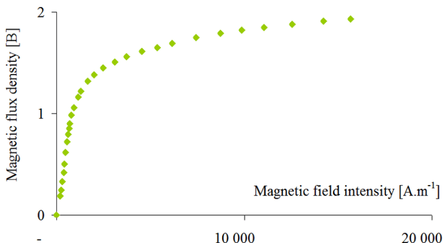
Figuur 4.1: BH-curve van ASI1018. Het is belangrijk dat de curve bij onze waarde voor B_g lineair is, zodat er geen saturatie optreedt en er geen magnetisch veld weglekt. [4]
