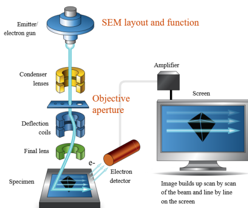
(a) Werkingsprincipe van een SEM waarbij de elektronenbundel over het sample wordt gescand en er secundaire elektronen los worden geslagen. [20]
