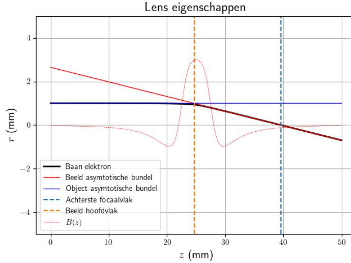
Figuur 3.13: Plot van numerieke oplossing van de paraxiale bewegingsvergelijking. De object en beeld asymptotische bundels snijden elkaar in het beeld hoofdvak, en de beeld asymptotische straal snijdt de symmetrie-as in het achterste focaalvlak van de lens. Deze opstelling heeft de volgende parameters: R_1 = 1.5\text{mm} , R_2 = 5\text{mm} , d = 5\text{mm} , B_g = 0.447\text{T} , \Phi = 30\text{ keV} .
