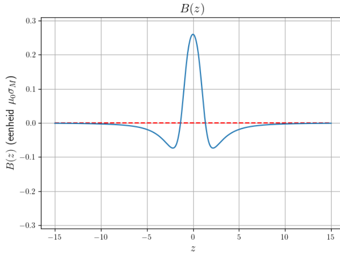
Figuur 3.5: Plot van B volgens vergelijking 3.2 voor parameters R_1 = 1 , R_2 = 2 , en d = 2 . Het veld is nu symmetrisch rond het midden van de lens en maximaal in het midden van de lens, zoals men zou verwachten.
