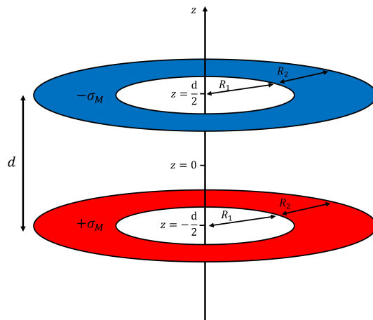
Figuur 3.4: Systeem met 2 annula met een luchtspleetbreedte van d rond een symmetrie-as. De annula hebben homogene oppervlaktepoolladingen gelijk aan \pm\sigma_M , wat aanleiding geeft tot een magnetisch veld. Dit is het systeem dat we beschouwen bij het afschatten van het magnetisch veld in onze lens.
