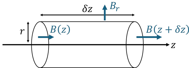
Figuur 2.4: We kunnen de tweede Maxwell gebruiken om een relatie te vinden tussen B_r en B(z) op de symmetrie-as van het systeem. We tekenen daarvoor een cilindervormig Gauss-oppervlak waardoor de totale flux \int \mathbf{B} \cdot d\mathbf{S} moet verdwijnen.
