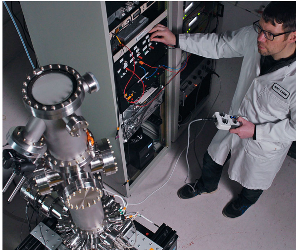
Figuur 1.2: NanoMI is een open-source project waarbij men tracht een modulaire transmissie-elektronenmicroscop met een versnelspanning van 50 keV te ontwikkelen. Men gebruikt elektrostatische Einzellenzen voor het afbuigen van de elektronen. [18]
