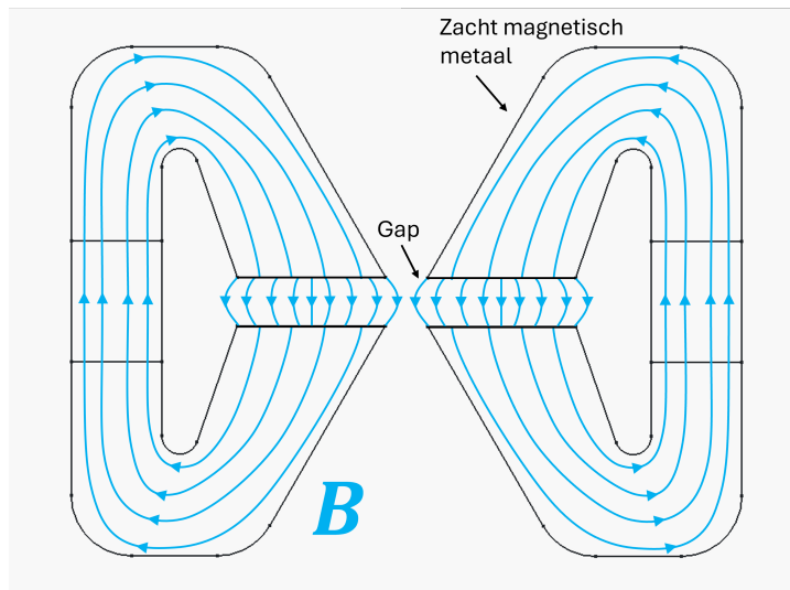
Figuur 3.1: Doorsnede van het ontwerp van onze permanente magneetlens. Een homogeen gemagnetiseerde Nd-ringmagneet maakt een sterk magnetisch veld dat door twee zacht magnetische poolschoenen wordt geconcentreerd in het gat van de lens.
