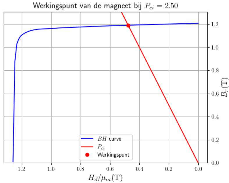
Figuur 4.2: Het werkpunt van de magneet bij P_{ci} = 2.5 . Dit is de ondergrens die we voor voor ons ontwerp kiezen om te voorkomen dat er demagnetisatie van de magneet zou optreden. Het werkpunt kan door een groot aantal onvoorziene factoren dichter dan verwacht bij de elleboog van de curve liggen, dus moeten we ervoor zorgen dat P_{ci} groot genoeg blijft.
