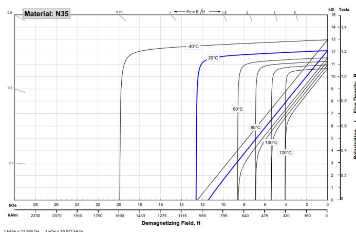
Figuur 3.9: BH-curve van graad N35 NdFeB voor verschillende temperaturen. Het aanleggen van een demagnetiserend veld doet de intrinsieke sterkte van de magneet licht verkleinen. Bij een zeer groot (extern) demagnetiserend veld passeren we de elleboog van de BH-curve en demagnetiseert de magneet, of wordt deze zelfs omgepoold. [3]
