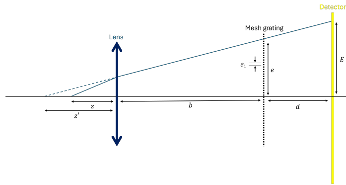
Figuur 4.8: Rear mesh shadowgraph methode voor een puntbron achter het focaalvlak van de lens. De elektronenbundel wordt nu niet gefocusseerd in een punt, maar de elektronenbundel is nog steeds divergerend wat een vergroting M > 1 geeft.
