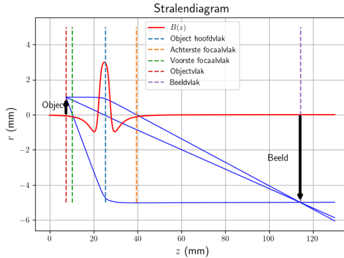
Figuur 3.14: Voorbeeld van beeldvorming met een permanente magneetlens. We beschouwen hier de drie hoofdstralen: de straal die door het achterste brandpunt gaat, de straal die door het midden van de lens gaat, en de straal die door het voorste brandpunt gaat. In dit geval krijgen we een vergroting M = 5 .
