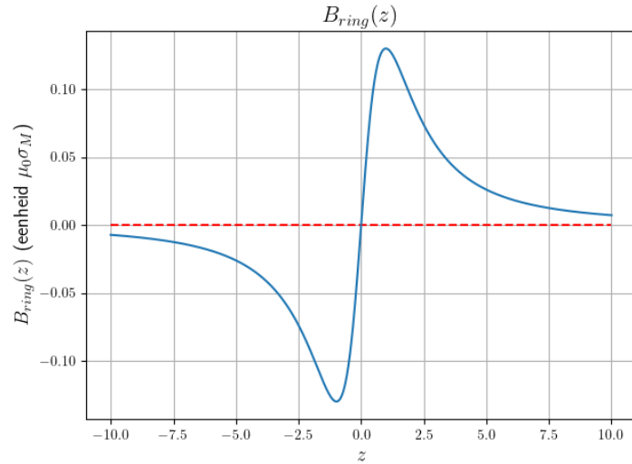
Figuur 3.3: Plot van B_{ring} volgens vergelijking 3.1 voor parameters R_1 = 1 en R_2 = 2 . Het veld is antisymmetrisch rond het midden van de ring, zoals men zou verwachten.
