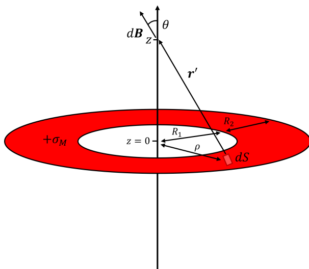
Figuur 3.2: Systeem met 1 annulus rond een symmetrie-as. De annulus heeft een homogene oppervlaktepoollading gelijk aan \sigma_M , wat aanleiding geeft tot een magnetisch veld.
