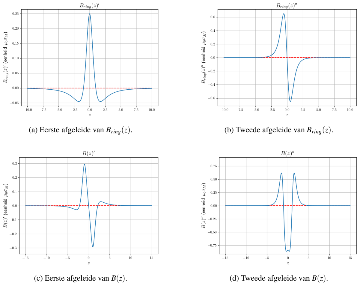
Figuur 3.6: Plots van de analytische afgeleiden van de magnetische velden voor 1 annulus en 2 annula met R_1 = 1 , R_2 = 2 , en d = 2 . Deze afgeleiden zullen we later gebruiken om de asymptotische aberratiecoëfficiënten van de lens te berekenen.
