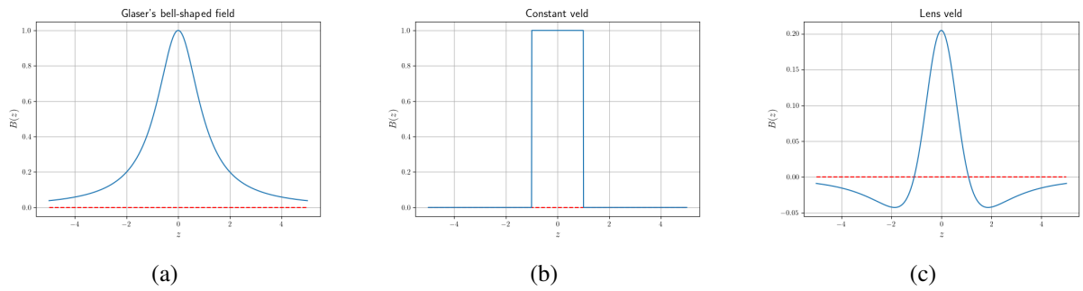
Figuur 3.12: Vergelijking tussen twee velden (Glaser's field en constant veld) waarvoor de paraxiale bewegingsvergelijking analytisch oplosbaar is en ons analytisch afgeschat veld. Het Glaser's field is gelijkaardig, maar heeft een bredere piek en valt trager af dan ons afgeschatte veld. Dit geeft een dikkere lens, wat ongewenst is.
