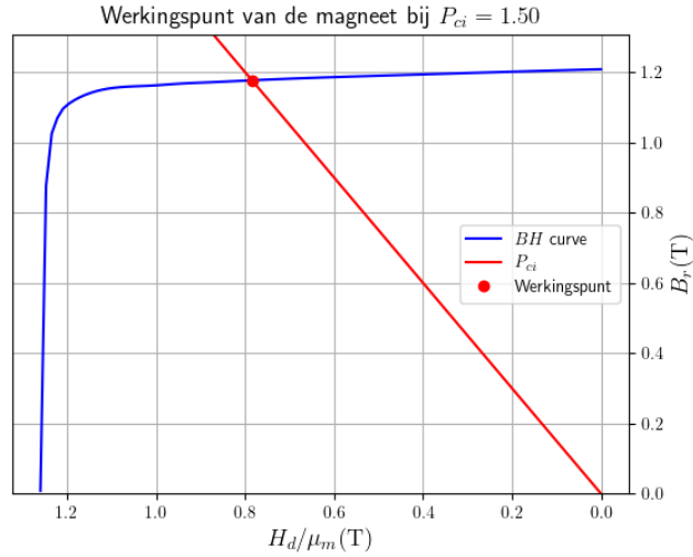
Figuur 3.10: Het werkpunt van de magneet kunnen we vinden door het snijpunt te bepalen van de BH-curve en de load line, waarvan de richtingscoëfficiënt afhangt van de intrinsieke permeantiecoëfficiënt P_c . Als het werkpunt niet voorbij de elleboog van de curve ligt, dan zal de magneet niet demagnetiseren.
