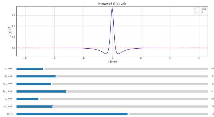
Figuur 3.11: Interactieve plot van B(z) in functie van de lensparameters. Deze functie kunnen we gebruiken om de afhankelijkheid van de verschillende parameters te bestuderen, en de lensparameters te optimaliseren om een gewenst magnetisch veld te krijgen. In dit geval gebruiken we de parameters R_1 = 0.8\text{mm} , R_2 = 3.25\text{mm} , en d_g = 0.8\text{mm} . De B_r instelling zorgt voor een herschaling van de BH-curve.
