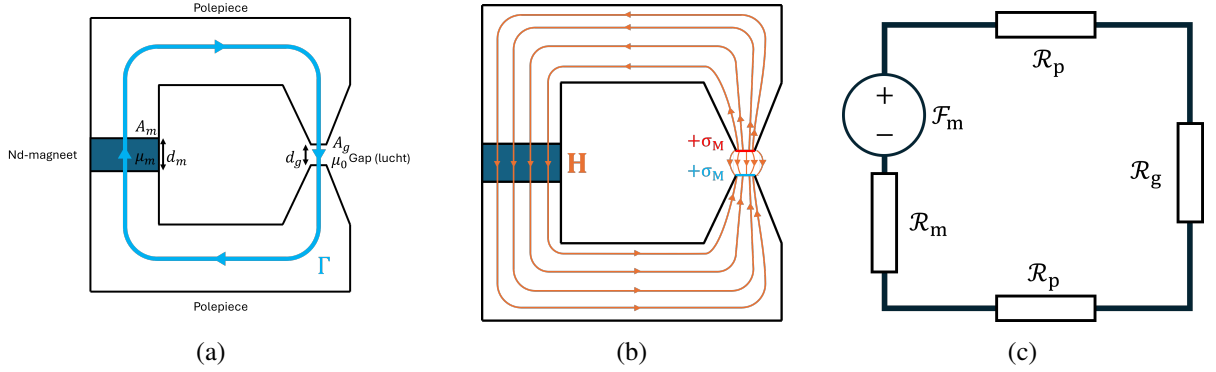
Figuur 3.8: Illustratie van het magnetisch circuit equivalent aan dat van de lens. De luchtspleet veroorzaakt demagnetiserend veld dat ervoor zorgt dat het oppervlakteveld B_m van de magneet kleiner wordt dan haar remanent veld B_r . Dit kunnen we wiskundig beschrijven door de analogie te maken met elektrische circuits, waarbij de magneet een bron van magnetomotorische kracht, en de luchtspleet een reluctantie voorstellen.
