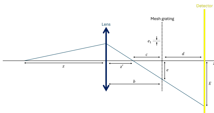
Figuur 4.7: Rear mesh shadowgraph methode voor een puntbron voor het focaalvlak van de lens. Door de vergroting M = \frac{E}{e} te meten is het mogelijk om het beeldpunt z' en de focale lengte f te bepalen.
