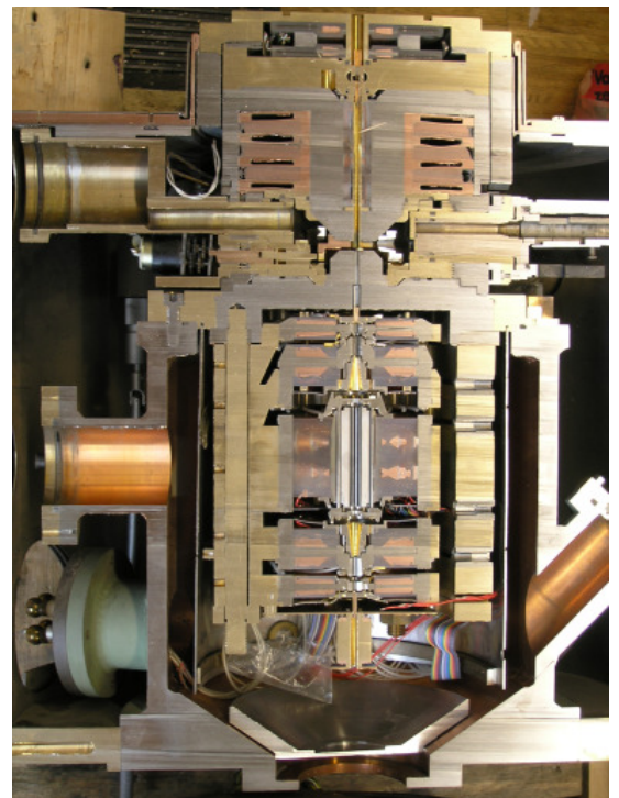
Figuur 1.1: Doorsnede van een Darmstadt aberratiecorrector. In een typische elektronenlens maakt men gebruik van spoelen om een magnetisch veld op te wekken. [11]
