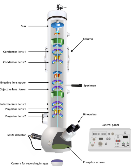
(a) Werkingsprincipe van een TEM waarbij een brede elektronenbundel heel het sample belicht en heel het beeld in 1 keer wordt opgenomen met een detector onder het sample. [21]
