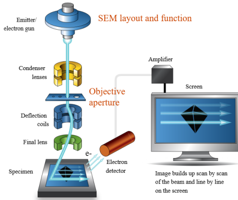
(a) Werkingsprincipe van een SEM waarbij de elektronenbundel over het sample wordt gescand en er secundaire elektronen los worden geslagen. [21]
