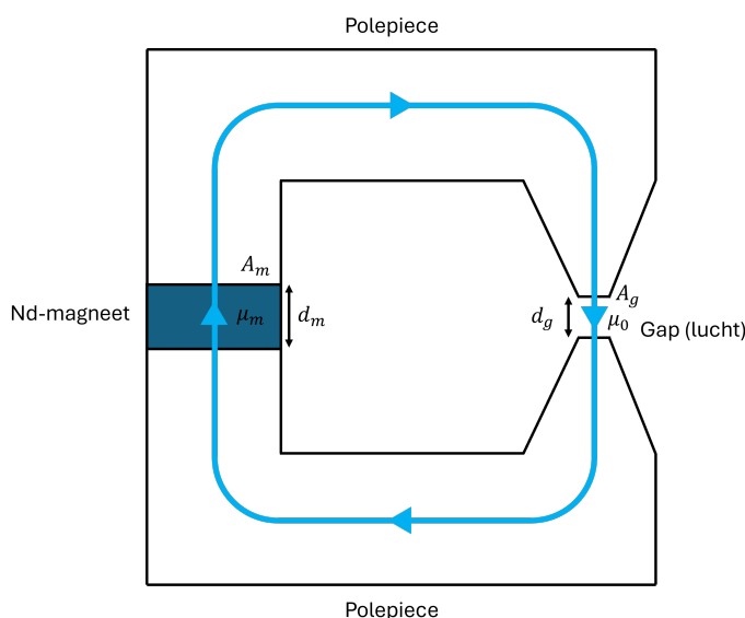
Figuur 5.7: Illustratie van het magnetisch circuit equivalent aan dat van de lens. De gap veroorzaakt een reluctantie die ervoor zorgt dat het oppervlakteveld B_m van de magneet kleiner wordt dan haar remanent veld B_r .
