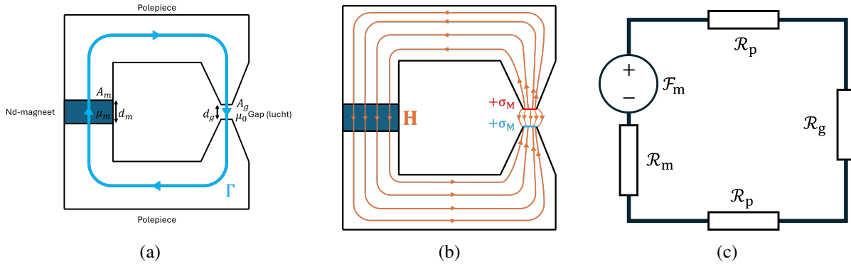
Figuur 5.8: Illustratie van het magnetisch circuit equivalent aan dat van de lens. De gap veroorzaakt demagnetiserend veld dat ervoor zorgt dat het oppervlakteveld B_m van de magneet kleiner wordt dan haar remanent veld B_r . Dit kunnen we wiskundig beschrijven door de analogie te maken met elektrische circuits, waarbij de magneet een bron van magnetomotorische kracht, en de gap een reluctantie voorstellen.
