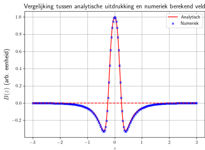
Figuur 5.7: Vergelijking tussen analytische uitdrukking en numeriek gesimuleerd veld voor R_1 = 2\text{mm} , R_2 = 3\text{mm} en d = 4\text{mm} . We zien dat de velden zeer goed overeenkomen.
