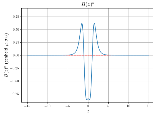
(d) Tweede afgeleide van B(z) .
