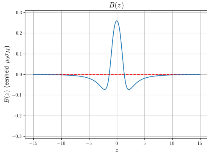
Figuur 5.5: Plot van B volgens vergelijking 5.2 voor parameters R_1 = 1 , R_2 = 2 , en d = 2 . Het veld is nu symmetrisch rond het midden van de lens en maximaal in het midden van de lens, zoals men zou verwachten.
