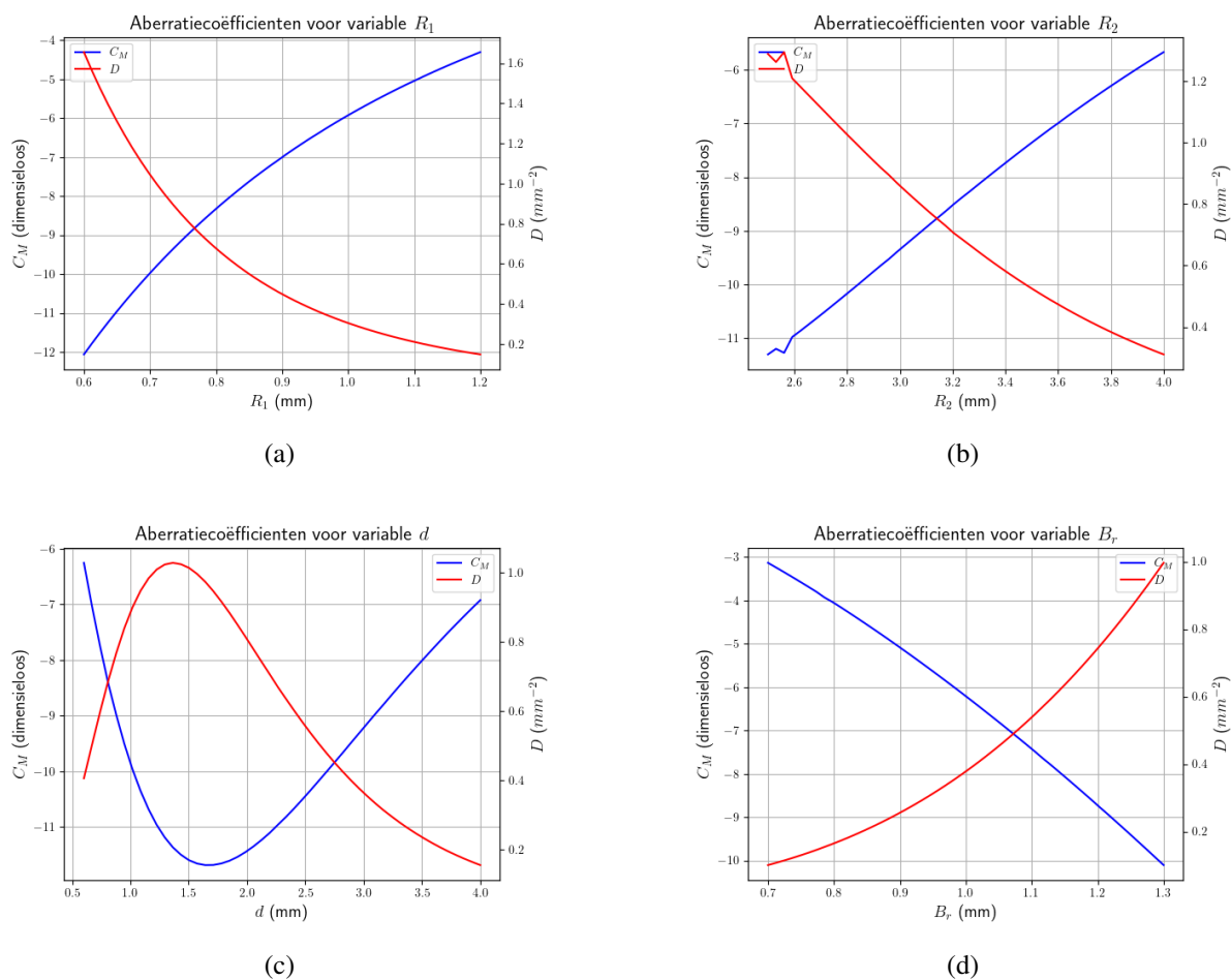
Figuur 5.19: Plots van aberratiecoëfficiënten D en C_M in functie van de geometrie van de lens. Deze plots geven een goed beeld van hoe de parameters aangepast kunnen worden om de aberratiecoëfficiënten te minimaliseren.
