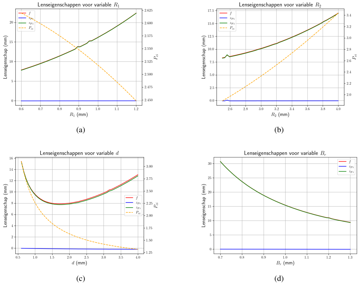
Figuur 5.17: Plots van lenseigenschappen en reluctantieterm in functie van de geometrie van de lens.
