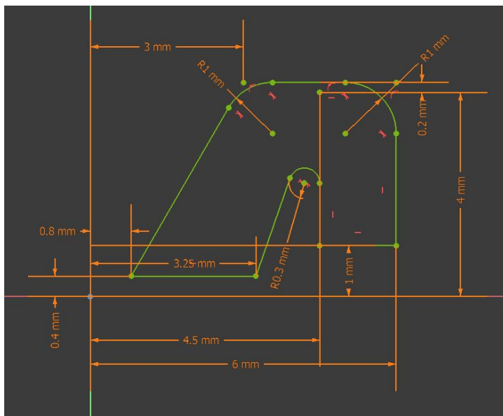
Figuur 5.20: 2D sketch in FreeCAD van een polepiece met de gekozen lensparameters Vervangen door technische tekening? .
