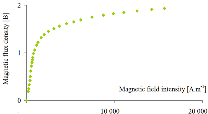
Figuur 5.15: BH -curve van ASI1018. Het is belangrijk dat de curve bij onze waarde voor B_g lineair is, zodat er geen saturatie optreedt en er geen magnetisch veld weglekt. [6]
