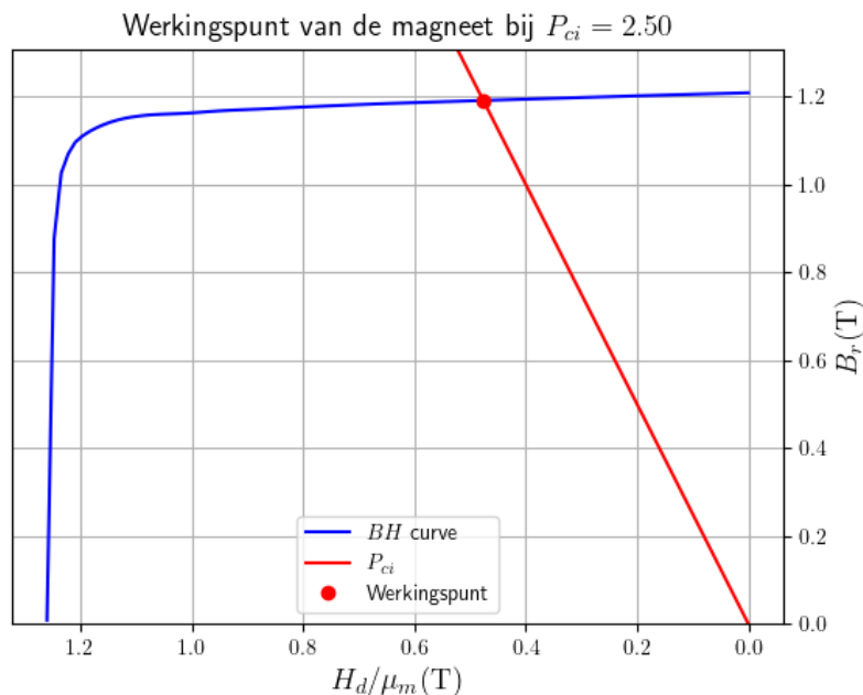
Figuur 5.16: Het werkpunt van de magneet bij P_{ci} = 2.5 . Dit is de ondergrens die we voor voor ons ontwerp kiezen om te voorkomen dat er demagnetisatie van de magneet zou optreden. Het werkpunt kan door een groot aantal onvoorziene factoren dichterbij de elleboog van de curve liggen, dus moeten we ervoor zorgen dat P_{ci} groot genoeg blijft.
