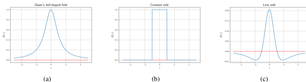
Figuur 5.10: Vergelijking tussen twee velden (Glaser's field en constant veld) waarvoor de paraxiale bewegingsvergelijking analytisch oplosbaar is en ons analytisch afgeschat veld. Het Glaser's field is gelijkaardig, maar heeft een bredere piek en valt trager af dan ons afgeschatte veld. Dit geeft een dikkere lens, wat ongewenst is.
