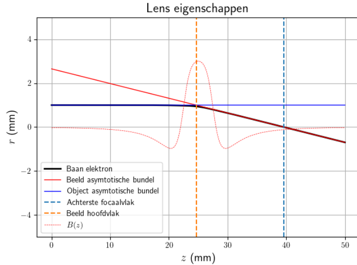
Figuur 5.11: Plot van numerieke oplossing van de paraxiale bewegingsvergelijking. De object en beeld asymptotische bundels snijden elkaar in het beeld hoofdvak, en de beeld asymptotische straal snijdt de symmetrie-as in het achterste focaalvlak van de lens. Deze opstelling heeft de volgende parameters: R_1 = 1.5\text{mm} , R_2 = 5\text{mm} , d = 5\text{mm} , B_g = 0.447\text{T} , \Phi = 30\text{KeV} .
