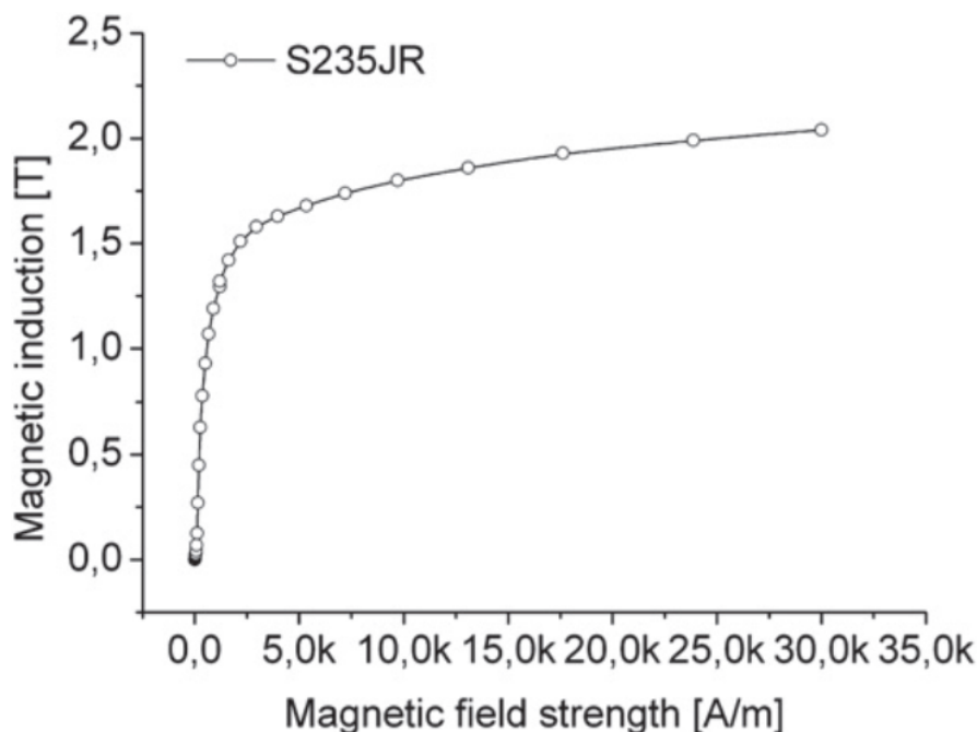
Figuur 5.13: BH -curve van S235JR. Het is belangrijk dat de curve bij onze waarde voor B_g lineair is, zodat er geen saturatie optreedt en er geen magnetisch veld weglekt. [BSE14]
