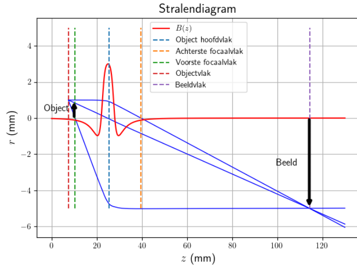
Figuur 5.12: Voorbeeld van beeldvorming met een permanente magneetlens. We beschouwen hier de drie hoofdstralen: de straal die door het achterste brandpunt gaat, de straal die door het midden van de lens gaat, en de straal die door het voorste brandpunt gaat. In dit geval krijgen we een magnificatie M = 5 .
