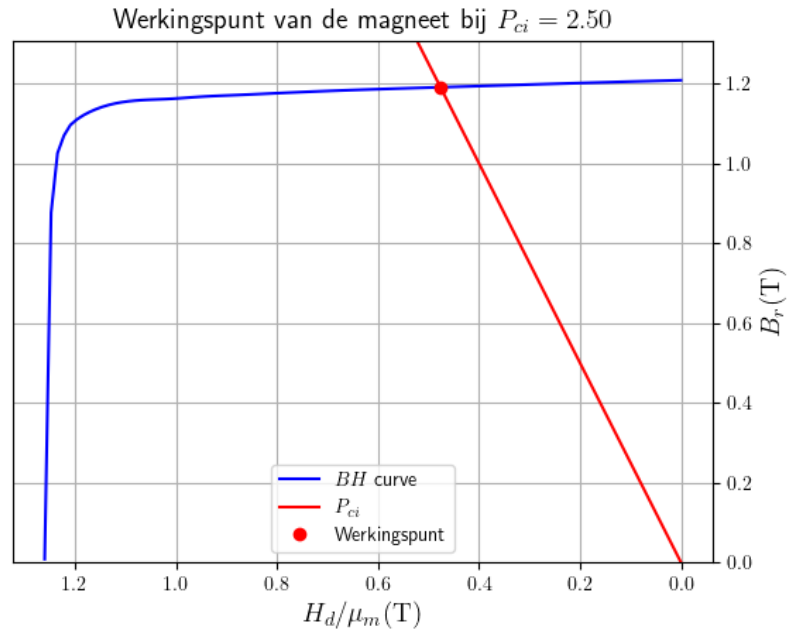
Figuur 5.14: Het werkingpunt van de magneet bij P_{ci} = 2.5 . Dit is de ondergrens die we voor voor ons ontwerp kiezen om te voorkomen dat er demagnetisatie van de magneet zou optreden. Het werkingpunt kan door een groot aantal onvoorziene factoren dichterbij de elleboog van de curve liggen, dus moeten we ervoor zorgen dat P_{ci} groot genoeg blijft.
