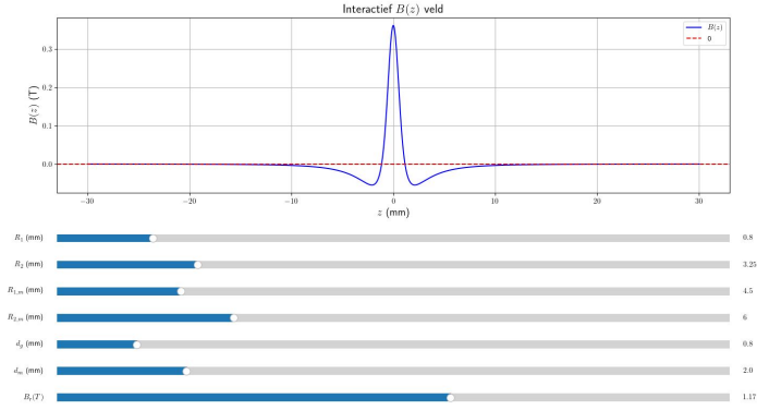
Figuur 4.10: Interactieve plot van B(z) in functie van de lensparameters. Deze functie kunnen we gebruiken om de afhankelijkheid van de verschillende parameters te bestuderen, en de lensparameters te optimaliseren om een gewenst magnetisch veld te krijgen. In dit geval gebruiken we de parameters R_1 = 0.8\text{mm} , R_2 = 3.25\text{mm} , en d_g = 0.8\text{mm} . De B_r instelling zorgt voor een herschaling van de BH-curve.
