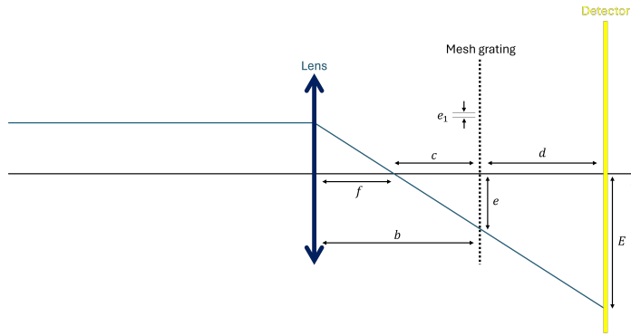
Figuur 5.9: Rear mesh shadowgraph methode voor een parallelle bundel. Door het gebruik van een parallelle bundel worden de inkomende elektronenbundels door de lens gefocuseerd in het focaalvlak achter de lens, wat de bepaling van de focale lengte iets vereenvoudigt.
