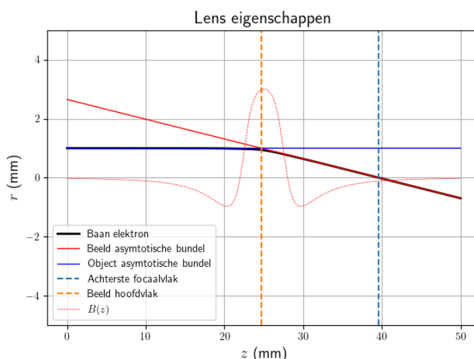
Figuur 4.12: Plot van numerieke oplossing van de paraxiale bewegingsvergelijking. De object en beeld asymptotische bundels snijden elkaar in het beeld hoofdvlak, en de beeld asymptotische straal snijdt de symmetrie-as in het achterste focaalvlak van de lens. Deze opstelling heeft de volgende parameters: R_1 = 1.5\text{mm} , R_2 = 5\text{mm} , d = 5\text{mm} , B_g = 0.447\text{T} , \Phi = 30\text{keV} .
