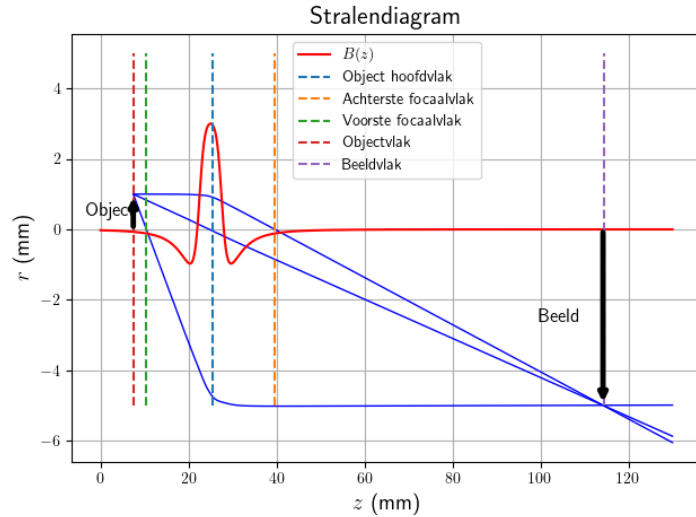
Figuur 4.13: Voorbeeld van beeldvorming met een permanente magneetlens. We beschouwen hier de drie hoofdstralen: de straal die door het achterste brandpunt gaat, de straal die door het midden van de lens gaat, en de straal die door het voorste brandpunt gaat. In dit geval krijgen we een magnificatie M = 5 .
