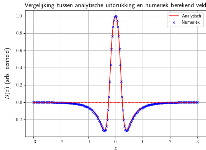
Figuur 4.6: Vergelijking tussen analytische uitdrukking en numeriek gesimuleerd veld voor R_1 = 2\text{mm} , R_2 = 3\text{mm} en d = 4\text{mm} . We zien dat de velden zeer goed overeenkomen.
