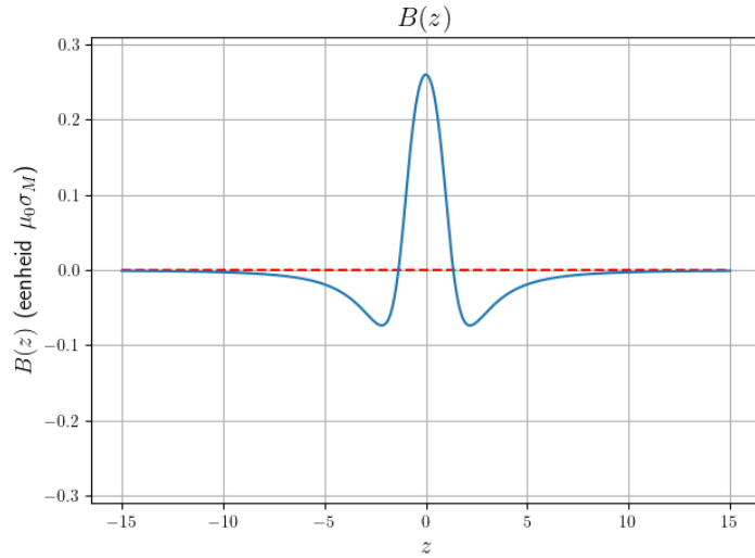
Figuur 4.4: Plot van B volgens vergelijking 4.2 voor parameters R_1 = 1 , R_2 = 2 , en d = 2 . Het veld is nu symmetrisch rond het midden van de lens en maximaal in het midden van de lens, zoals men zou verwachten.
