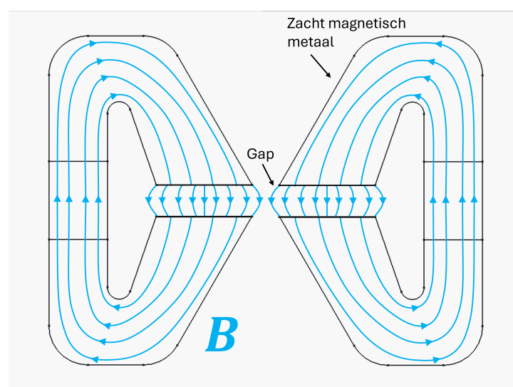
Figuur 3.1: Cross-sectie van het ontwerp van onze permanente magneetlens. Een homogeen gemagnetiseerde Nd-ringmagneet maakt een sterk magnetisch veld dat door twee zacht magnetische poleschoenen wordt geconcentreerd in het het gat van de lens.
