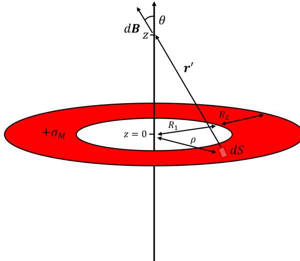
Figuur 4.1: Systeem met 1 annulus rond een symmetrie-as. De annulus heeft een homogene oppervlaktepoolloading gelijk aan \sigma_M , wat aanleiding geeft tot een magnetisch veld.
