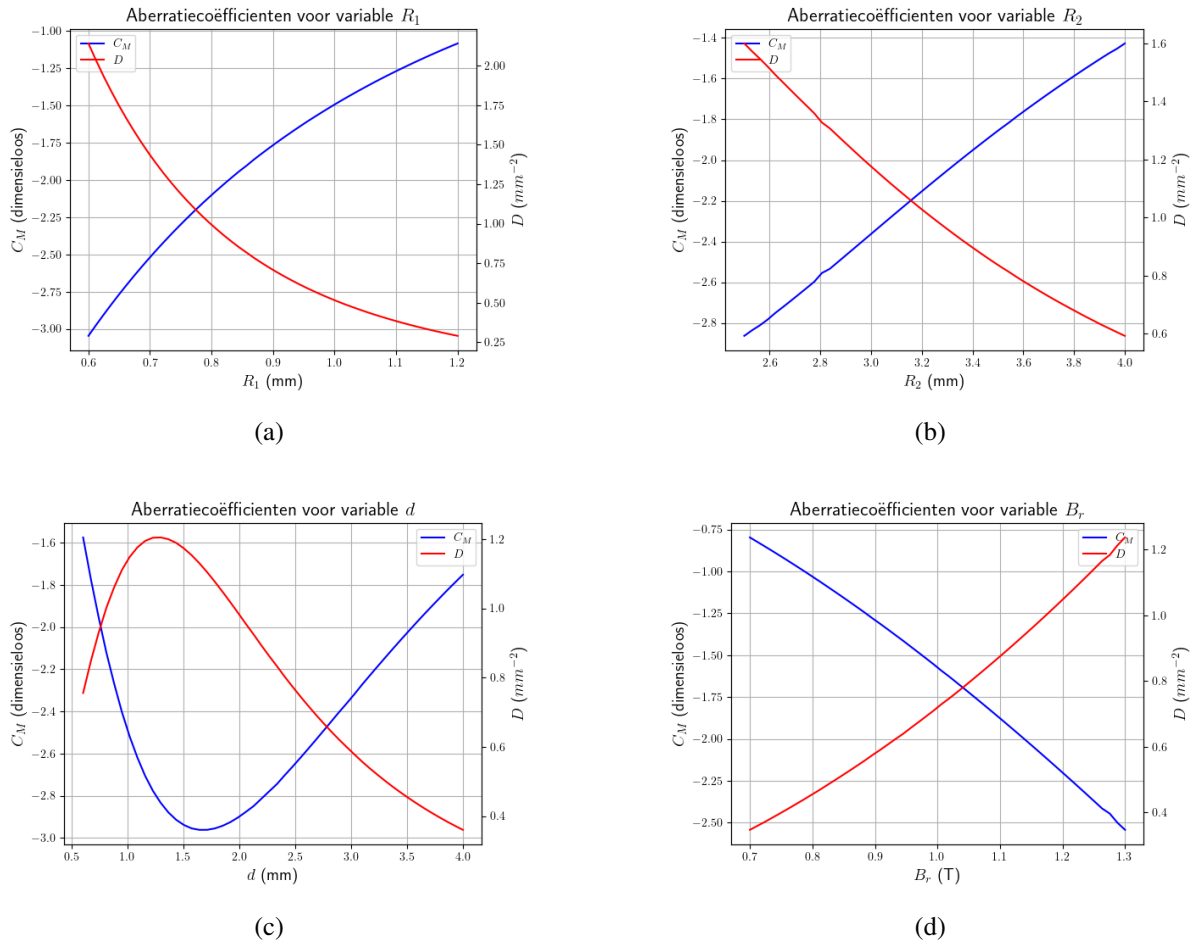
Figuur 5.5: Plots van aberratiecoëfficiënten D en C_M in functie van de geometrie van de lens bij z_0 = 25\text{mm} . Deze plots geven een goed beeld van hoe de parameters aangepast kunnen worden om de aberratiecoëfficiënten te minimaliseren.
