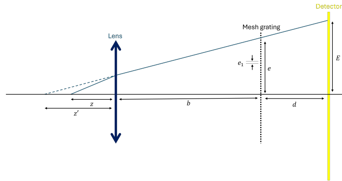
Figuur 5.8: Rear mesh shadowgraph methode voor een puntbron achter het focaalvlak van de lens. De elektronenbundel wordt nu niet gefocuseerd in een punt, maar de elektronenbundel is nog steeds divergerend wat een magnificatie M > 1 geeft.
