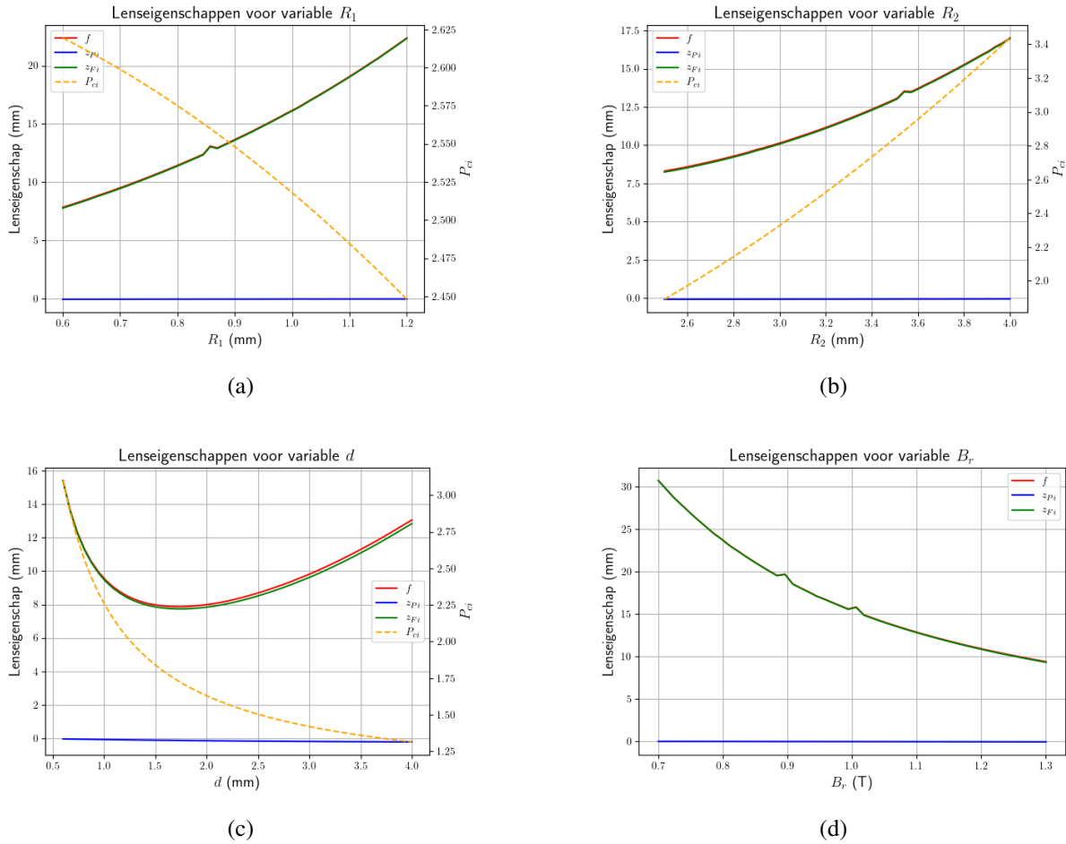
Figuur 5.3: Plots van lenseigenschappen en reluctantieterm in functie van de geometrie van de lens. Deze plots geven een goed beeld van hoe de parameters aangepast kunnen worden om de lenseigenschappen naar wens te optimaliseren. Naast de reluctantieterm moet er ook rekening gehouden worden met de maximale fluxdichtheid in de poleschoenen, welke niet te hoog mag zijn om saturatie-effecten te voorkomen.
