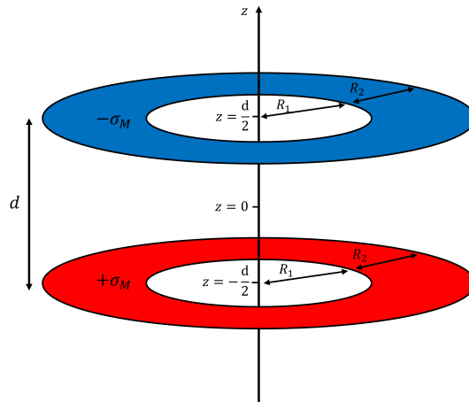
Figuur 4.3: Systeem met 2 annula met een gapbreedte van d rond een symmetrie-as. De annula hebben homogene oppervlaktepoo-ladings gelijk aan \pm\sigma_M , wat aanleiding geeft tot een magnetisch veld. Dit is het systeem dat we beschouwen bij het afschatten van het magnetisch veld in onze lens.
