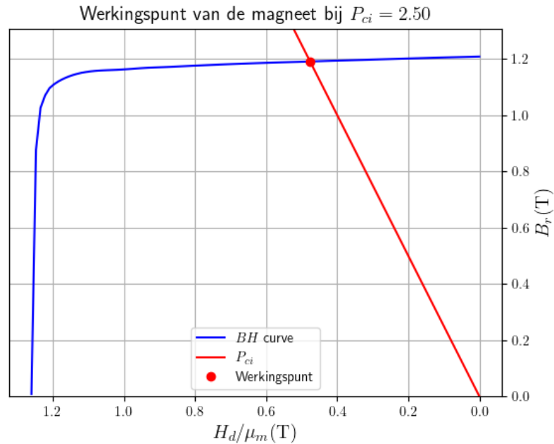
Figuur 5.2: Het werkpunt van de magneet bij P_{ci} = 2.5 . Dit is de ondergrens die we voor ons ontwerp kiezen om te voorkomen dat er demagnetisatie van de magneet zou optreden. Het werkpunt kan door een groot aantal onvoorziene factoren dichter dan verwacht bij de elleboog van de curve liggen, dus moeten we ervoor zorgen dat P_{ci} groot genoeg blijft.
