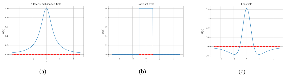
Figuur 4.11: Vergelijking tussen twee velden (Glaser's field en constant veld) waarvoor de paraxiale bewegingsvergelijking analytisch oplosbaar is en ons analytisch afgeschat veld. Het Glaser's field is gelijkaardig, maar heeft een bredere piek en valt trager af dan ons afgeschatte veld. Dit geeft een dikkere lens, wat ongewenst is.
