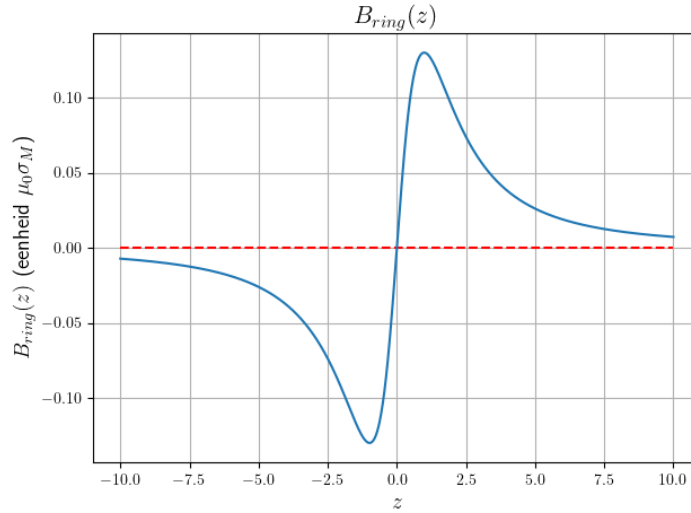
Figuur 4.2: Plot van B_{ring} volgens vergelijking 4.1 voor parameters R_1 = 1 en R_2 = 2 . Het veld is antisymmetrisch rond het midden van de ring, zoals men zou verwachten.
