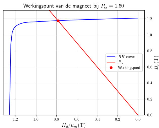
Figuur 5.9: Het werkpunt van de magneet kunnen we vinden door het snijpunt te bepalen van de BH -curve en de load line, waarvan de richtingscoëfficiënt afhangt van de intrinsieke permeantiecoëfficiënt P_c . Als het werkpunt niet voorbij de elleboog van de curve ligt, dan zal de magneet niet demagnetiseren.
