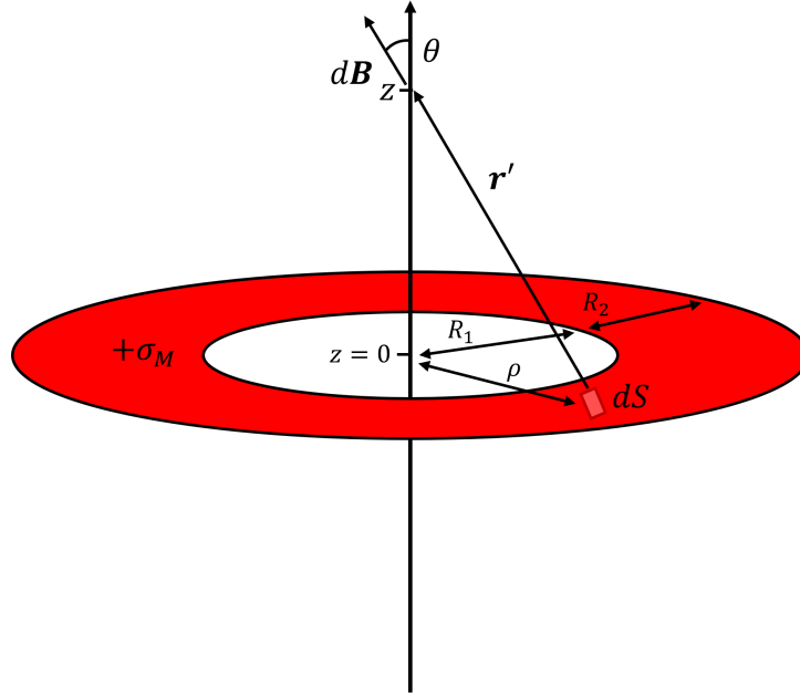
Figuur 5.2: Systeem met 1 annulus rond een symmetrie-as. De annulus heeft een homogene oppervlaktepooilading gelijk aan \sigma_M , wat aanleiding geeft tot een magnetisch veld.
