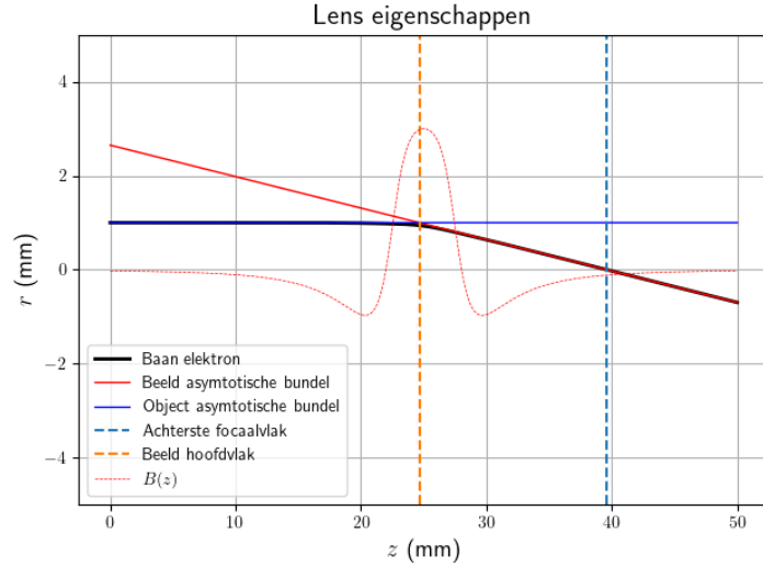
Figuur 4.13: Plot van numerieke oplossing van de paraxiale bewegingsvergelijking. De object en beeld asymptotische bundels snijden elkaar in het beeld hoofdvlak, en de beeld asymptotische straal snijdt de symmetrie-as in het achterste focaalvlak van de lens. Deze opstelling heeft de volgende parameters: R_1 = 1.5\text{mm} , R_2 = 5\text{mm} , d = 5\text{mm} , B_g = 0.447\text{T} , \Phi = 30\text{KeV} .
