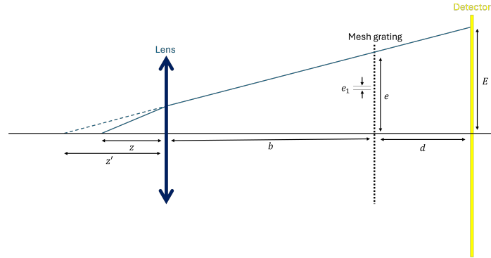
Figuur 4.22: Rear mesh shadowgraph methode voor een puntbron achter het focaalvlak van de lens. De elektronenbundel wordt nu niet gefocusseerd in een punt, maar de elektronenbundel is nog steeds divergerend wat een magnificatie M > 1 geeft.
