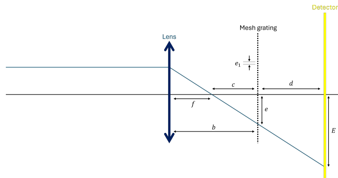
Figuur 4.23: Rear mesh shadowgraph methode voor een parallelle bundel. Door het gebruik van een parallelle bundel worden de inkomende elektronenbundels door de lens gefocusseerd in het focaalvlak achter de lens, wat de bepaling van de focale lengte iets vereenvoudigt.
