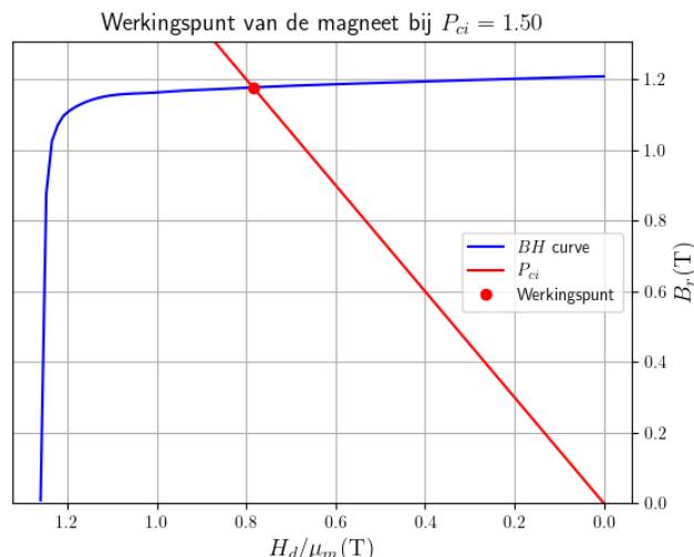
Figuur 4.10: Het werkingpunt van de magneet kunnen we vinden door het snijpunt te bepalen van de BH -curve en de load line, waarvan de richtingscoëfficiënt afhangt van de intrinsieke permeantiecoëfficiënt P_c . Als het werkingpunt niet voorbij de elleboog van de curve ligt, dan zal de magneet niet demagnetiseren.
