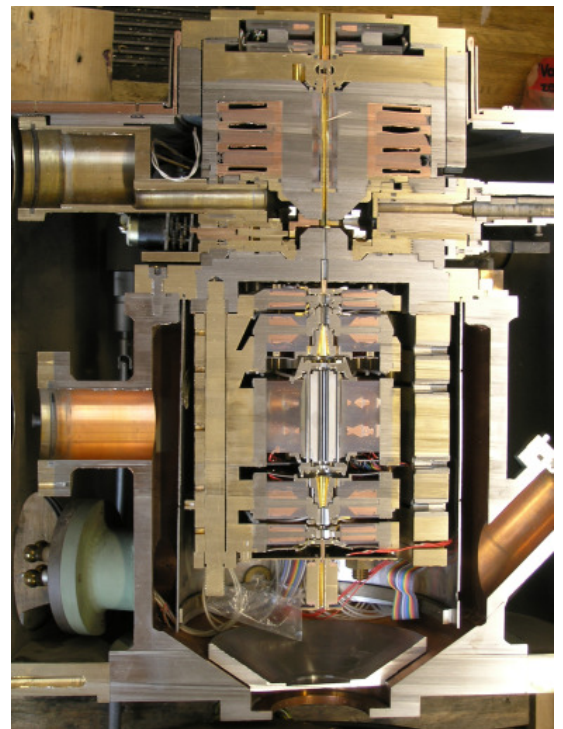
Figuur 1.1: Doorsnede van een Darmstadt aberratiecorrector. In een typische elektronenlens maakt men gebruik van spoelen om een magnetisch veld op te wekken. [12]
