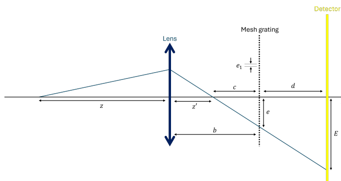
Figuur 4.21: Rear mesh shadowgraph methode voor een puntbron voor het focaalvlak van de lens. Door de magnificatie M = \frac{E}{e} te meten is het mogelijk om het beeldpunt z' en de focale lengte f te bepalen.
