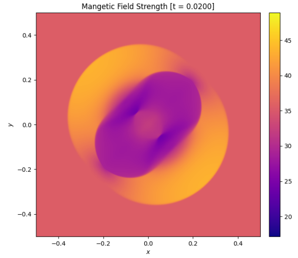
(b) 2D, |\mathbf{B}|
