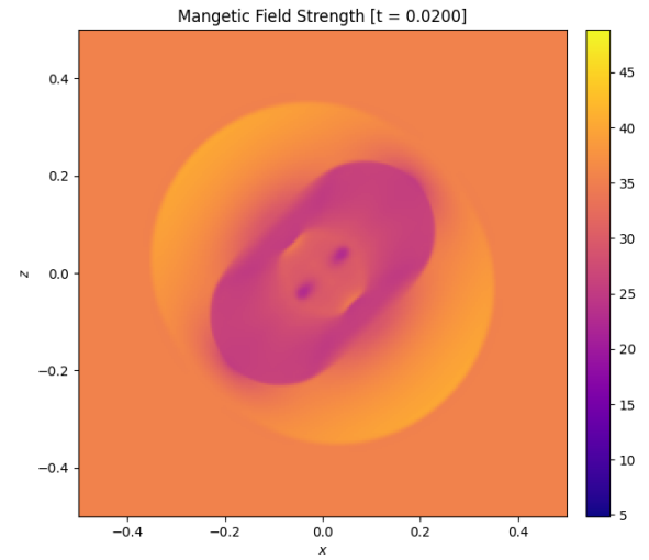
(d) 3D, |\mathbf{B}| (mid-plane slice)
